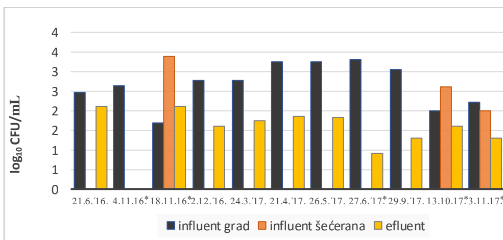
Slika 16. Sulfit-reducirajuće bakterije u ulaznoj i izlaznoj otpadnoj vodi na Uređaju za pročišćavanje otpadnih voda u Virovitici. Datumi uzorkovanja tijekom kojih su se gradska otpadna voda i otpadne voda tvornice šećera pročišćavale zajedno označeni su zvjezdicom (*).
