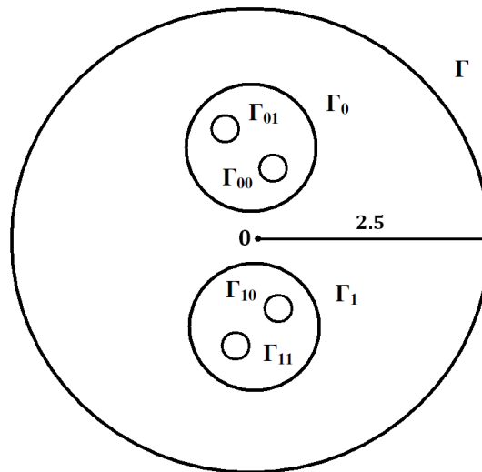
Slika 2.3: Konstrukcija Cantorova skupa
