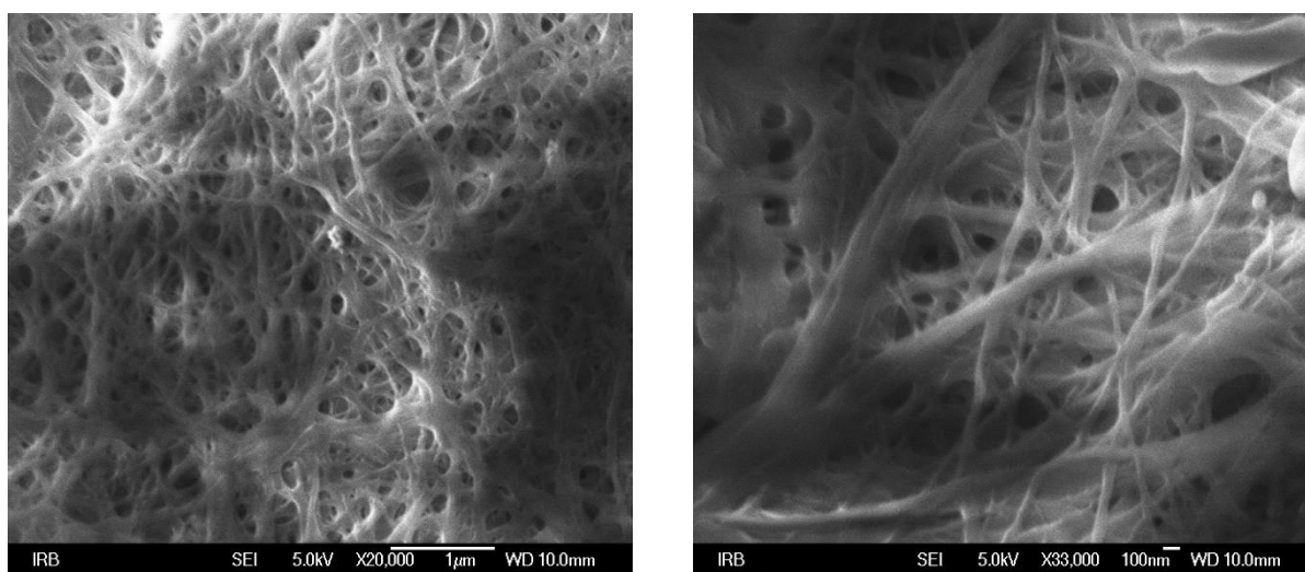
Slika 105. Prikaz morfologije polimera nastalog iz acetonitrilnog gela spoja 17 Grubbsovim katalizatorom II. generacije
