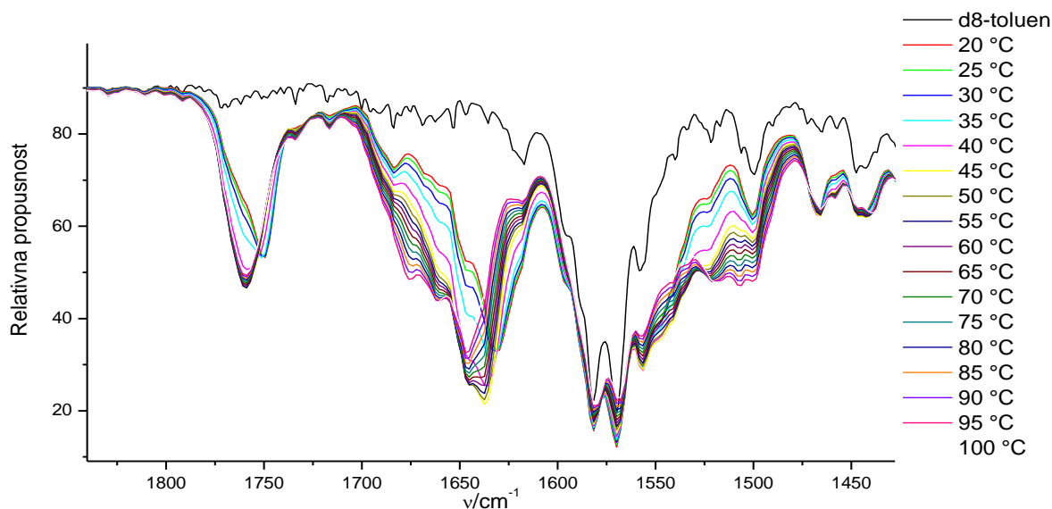
Slika 52. FTIR-spektri spoja 17 u toluenskom gelu pri različitim temperaturama.
