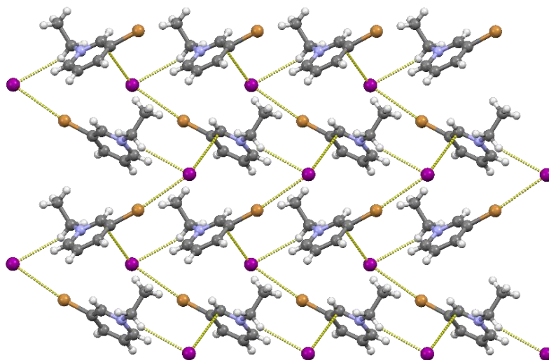
Slika 16. Kationi [ N -Et-3-BrPy] + i jodidni anioni povezani u slojeve halogenskim vezama C–Br···I − , vodikovim vezama C–H···I − i kontaktima anion- \pi u strukturi [ N -Et-3-BrPy]I.
