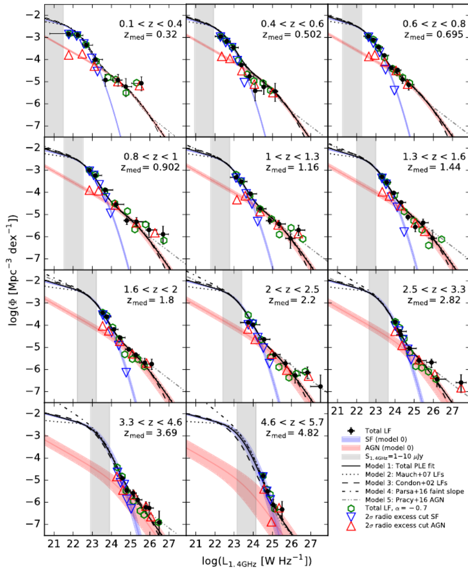
Slika 1.11: Prikaz ukupnih funkcija luminozitetu za različite vrijednosti crvenog pomaka. Kružićima su označene vrijednosti funkcija luminozitetu koje su dobivene V_{max} metodom iz kataloga COSMOS polja. Pune crne krivulje predstavljaju funkcije luminozitetu za ukupan broj izvora dobivene evolucijom lokalne funkcije luminozitetu. Lokalna funkcija luminozitetu je opisana analitičkim modelom i dobivena je prilagodbom na podatke iz kataloga. Plavom linijom su prikazani rezultati modela za SF galaksije, dok su crvenom bojom prikazani rezultati modela za AGN galaksije. Preuzeto iz [19].
