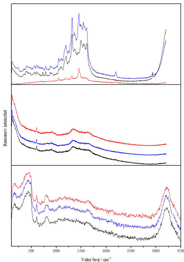
Slika 25. SERS spektri DTB koncentracije 1 \times 10^{-7} \text{ mol L}^{-1} (crno), 1 \times 10^{-6} \text{ mol L}^{-1} (plavo) i 1 \times 10^{-5} \text{ mol L}^{-1} (crveno), u koloidnoj suspenziji AgNP_PVP nakon pobude zračenjem pri 532, 785 i 1064 nm.
