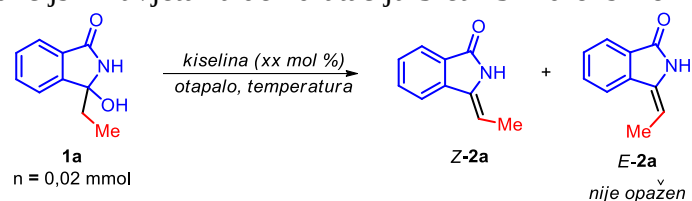
Tablica 2. Probir reakcijskih uvjeta za dehidraciju 3-etil-3-hidroksiizoinolinona 1a
