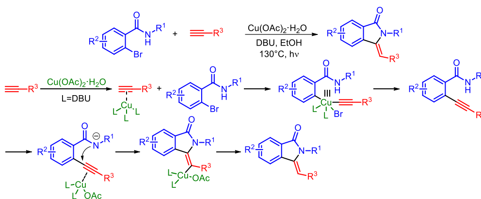
Shema 22. Mikrovalno potpomognuta priprava Z-3-metilenizindolinona reakcijom 2-brombenzamida i terminalnih alkina katalizirana s \text{Cu}(\text{OAc})_2 \cdot \text{H}_2\text{O}
