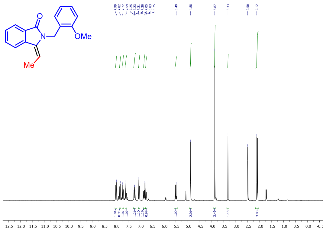
Slika D53. ^1\text{H} NMR spektar ( E )-3-etiliden-2-(2-metoksibenzil)izoindolinona ( E -2h)
