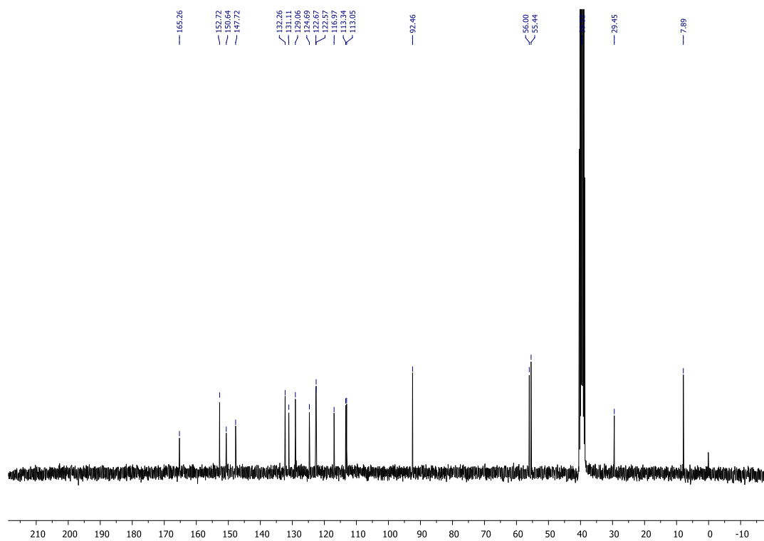
Slika D21. 13 C NMR spektar 2-(2,5-dimetoksifenil)-3-etil-3-hidroksiizoinolinona ( 10 )
