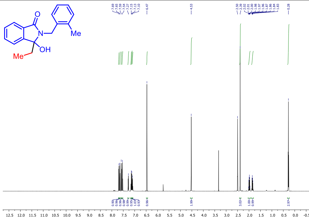
Slika D10. 1 H NMR spektar 3-etil-3-hidroksi-2-(2-metilbenzil)izoidolinona ( 1i )
