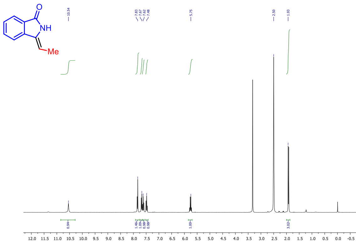
Slika D34. 1 H NMR spektar (Z)-3-etilidenizoindolinona (2a)
