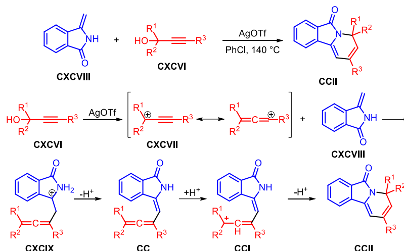
Shema 38. Reakcija i mehanizam nastajanja 1,5-dihidroindolizin-3(2H)-ona iz 3-metilenizindolinona i propargilnih alkohola katalizirana s AgOTf
