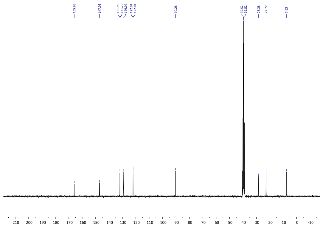
Slika D5. 13 C NMR spektar 3-etil-3-hidroksi-2-metilizoindolinona (1f)
