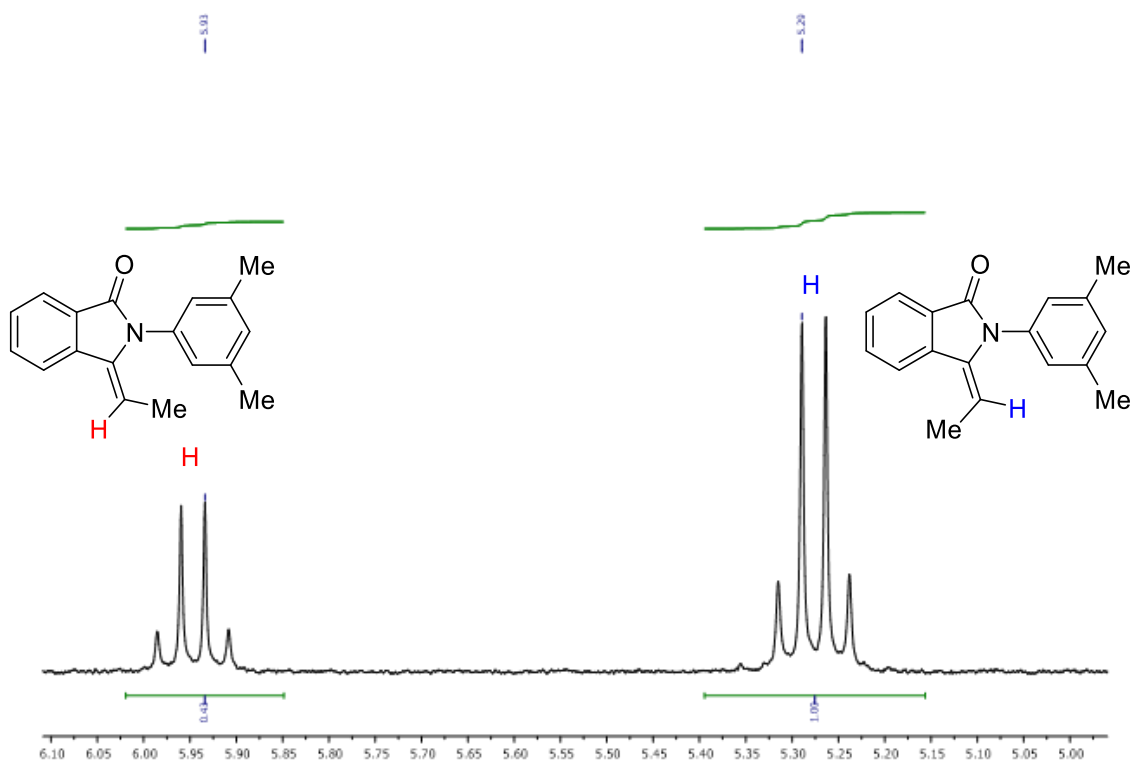
Slika D78. Segment ^1\text{H} NMR spektra spoja 2q
