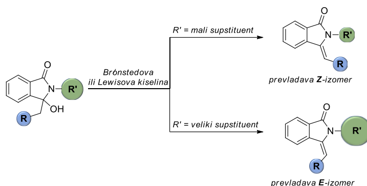
Shema 1. Koncept stereoselektivnog dehidratiranja 3-alkil-3-hidroksiizindolinona
