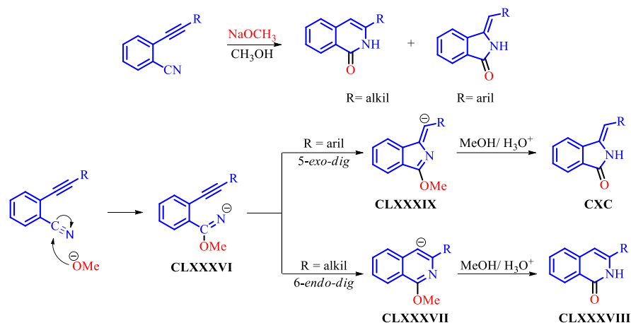
Shema 34. Priprava izoindolinonskih i izokinolinonskih struktura iz o -alkinilbenzonitrila
