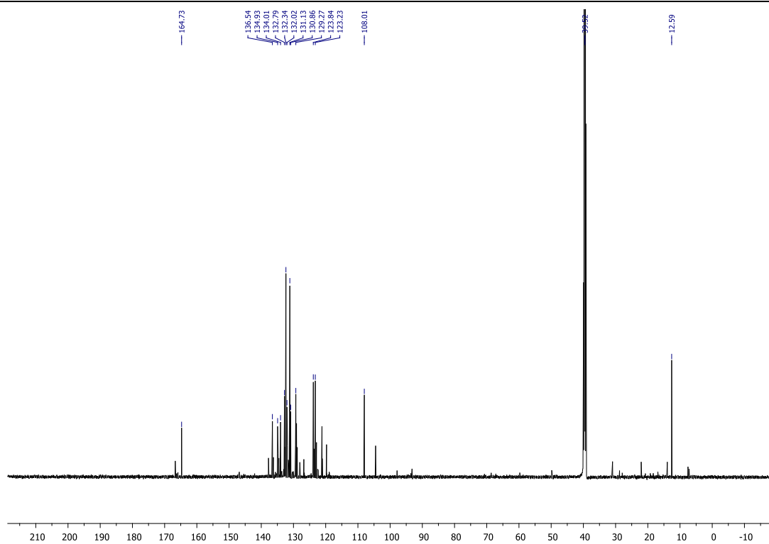
Slika D87. ^{13}\text{C} NMR spektar ( E )-2-(4-bromfenil)-3-etilidenizoindolinona ( E -2s)
