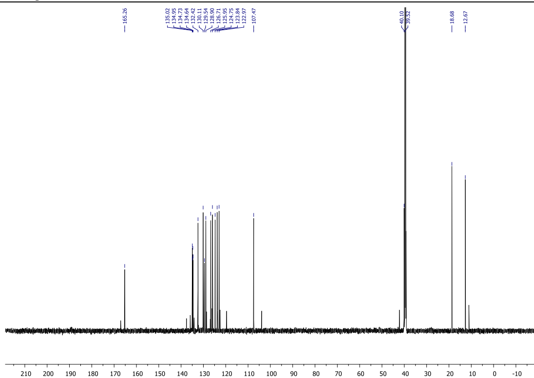
Slika D59. 13 C NMR spektar ( E )-3-etiliden-2-(2-metilbenzil)izoindolinona ( E -2i)
