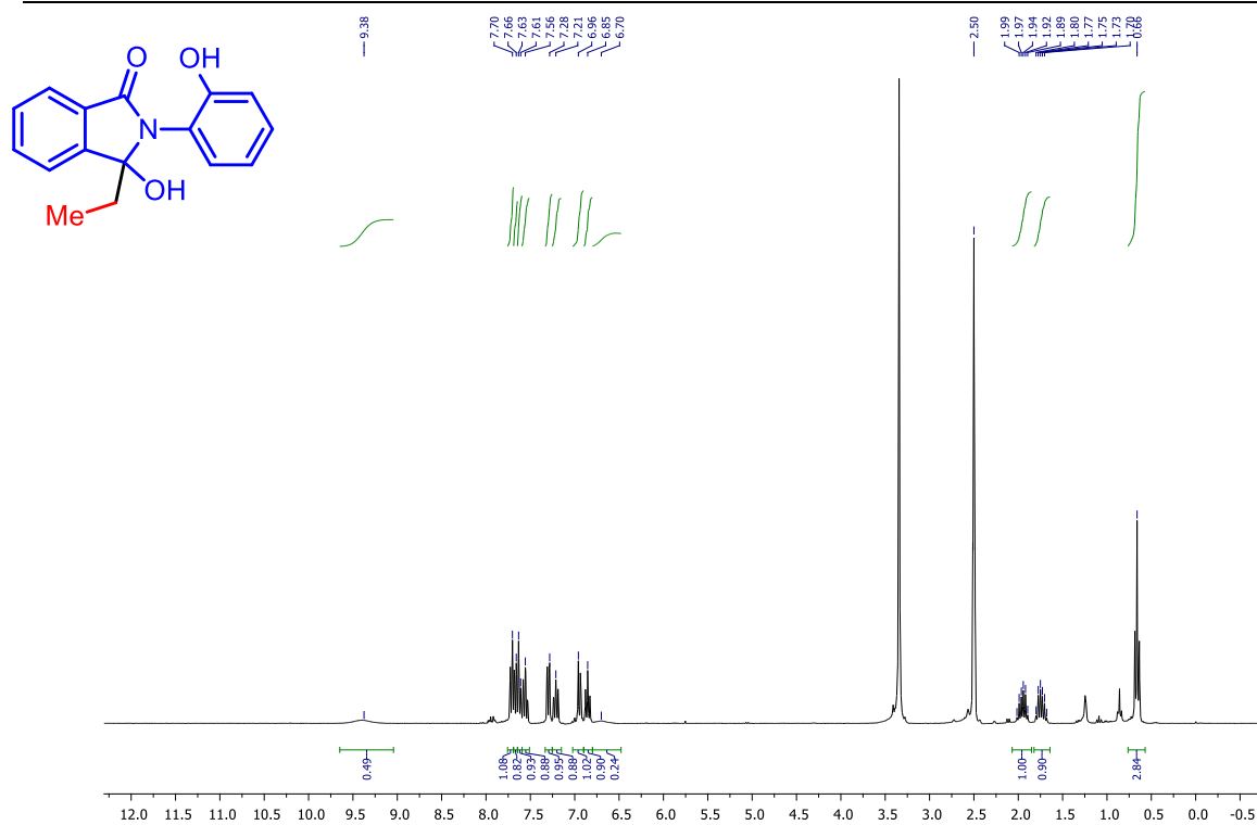
Slika D14. 1 H NMR spektar 3-etil-3-hidroksi-2-(2-hidroksifenil)izoinolinona (1k)
