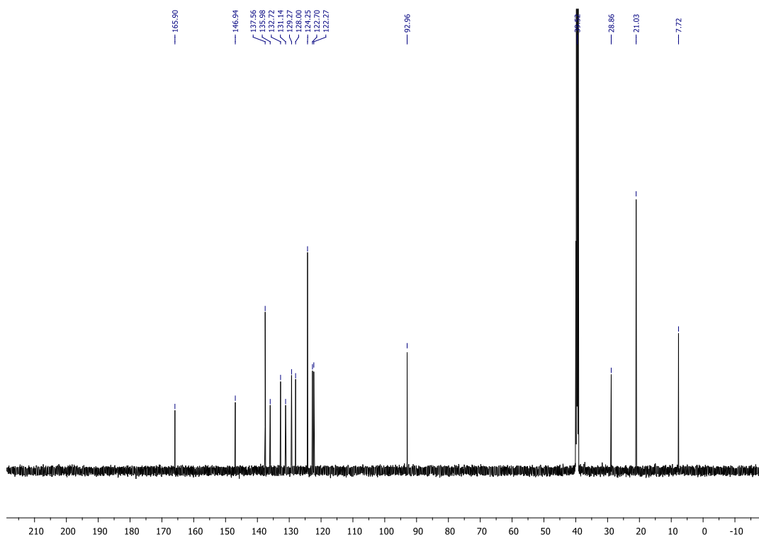
Slika D25. 13 C NMR spektar 2-(3,5-dimetilfenil)-3-etil-3-hidroksiizoinolinona ( 1q )
