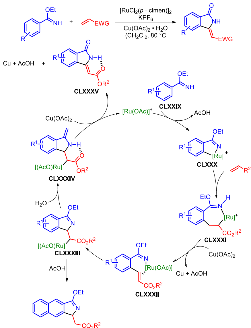
Shema 29. Oksidativno alkeniliranje i anulacija benzimidata i alkena katalizirana kompleksom [(RuCl 2 ( p -cimen)) 2 ]
