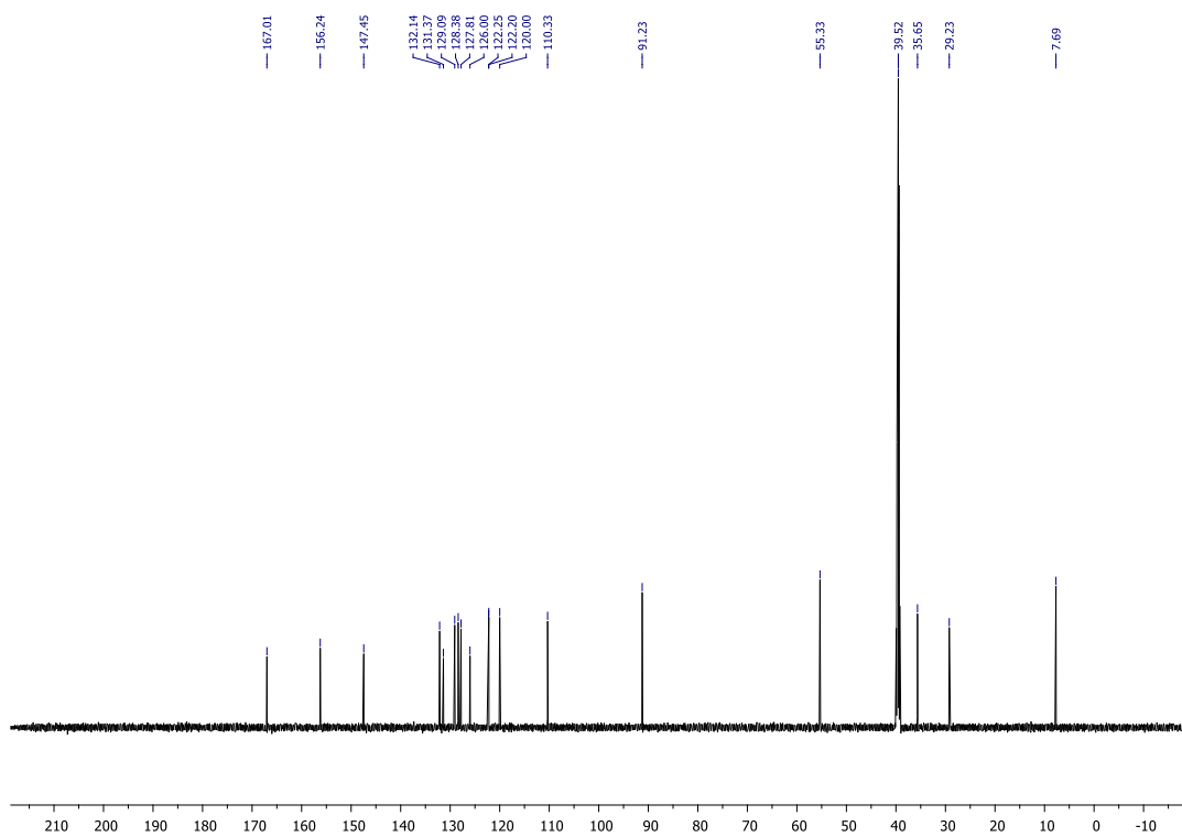
Slika D9. 13 C NMR spektar 3-etil-3-hidroksi-2-(2-metoksibenzil)izoindolinona ( 1h )
