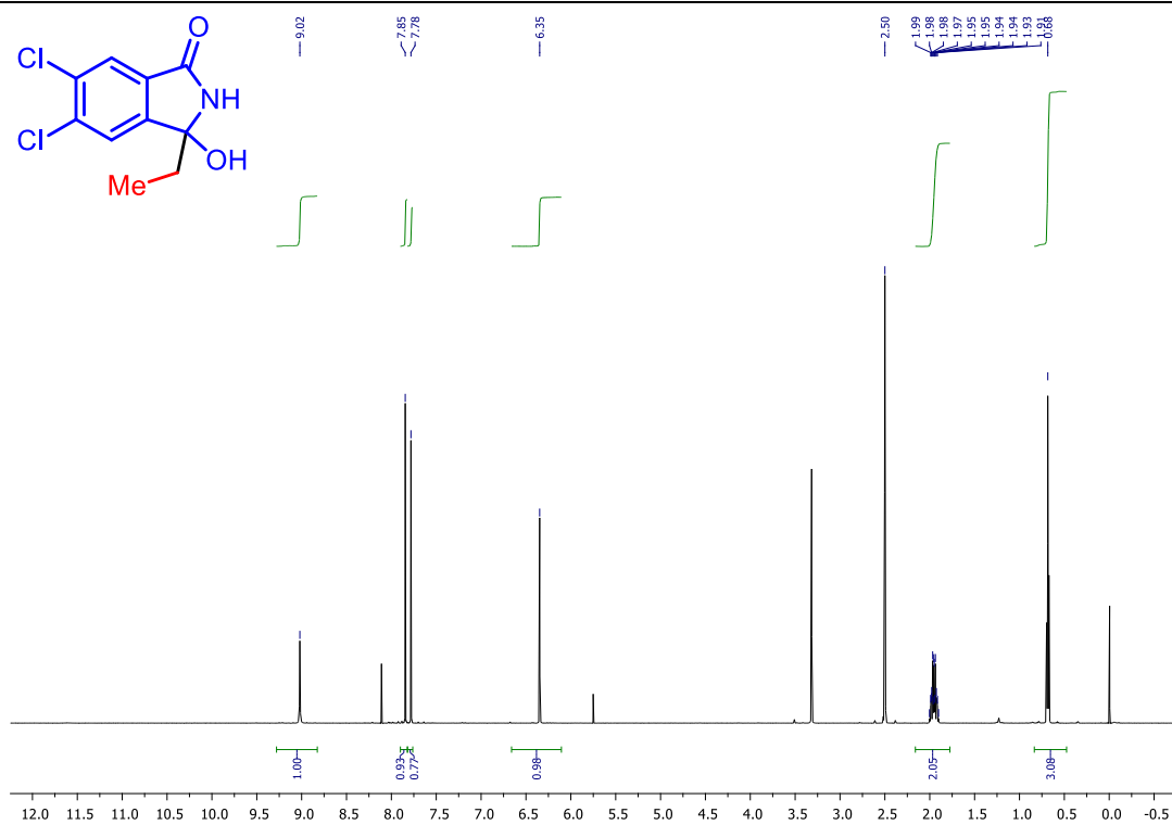
Slika D2. ^1\text{H} NMR spektar 5,6-diklor-3-etil-3-hidroksiizoinolinona ( 1e )
