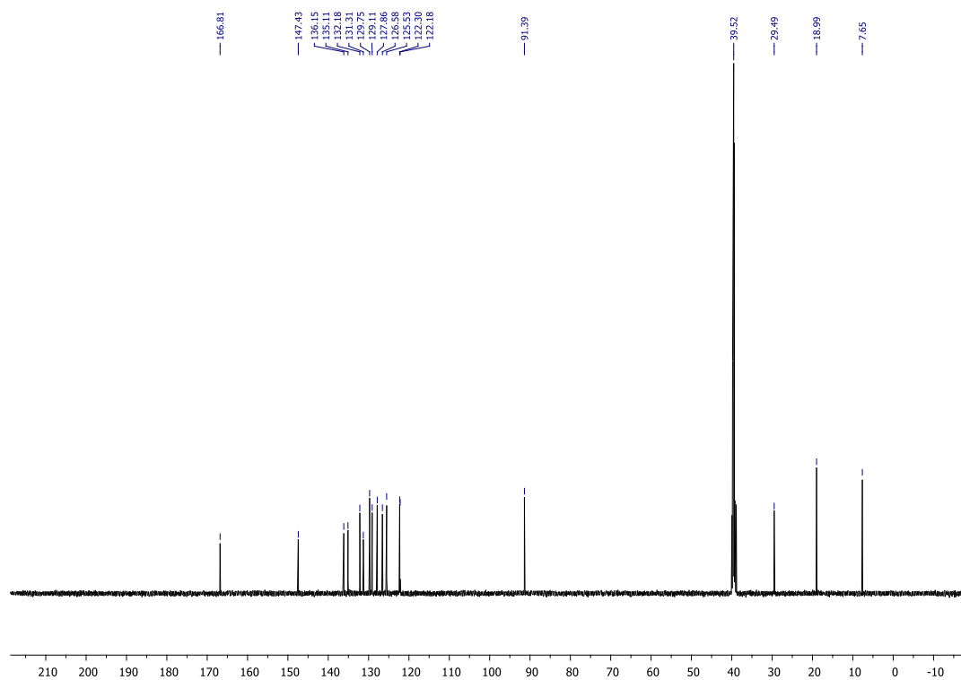
Slika D11. 13 C NMR spektar 3-etil-3-hidroksi-2-(2-metilbenzil)izoidolinona ( 1i )
