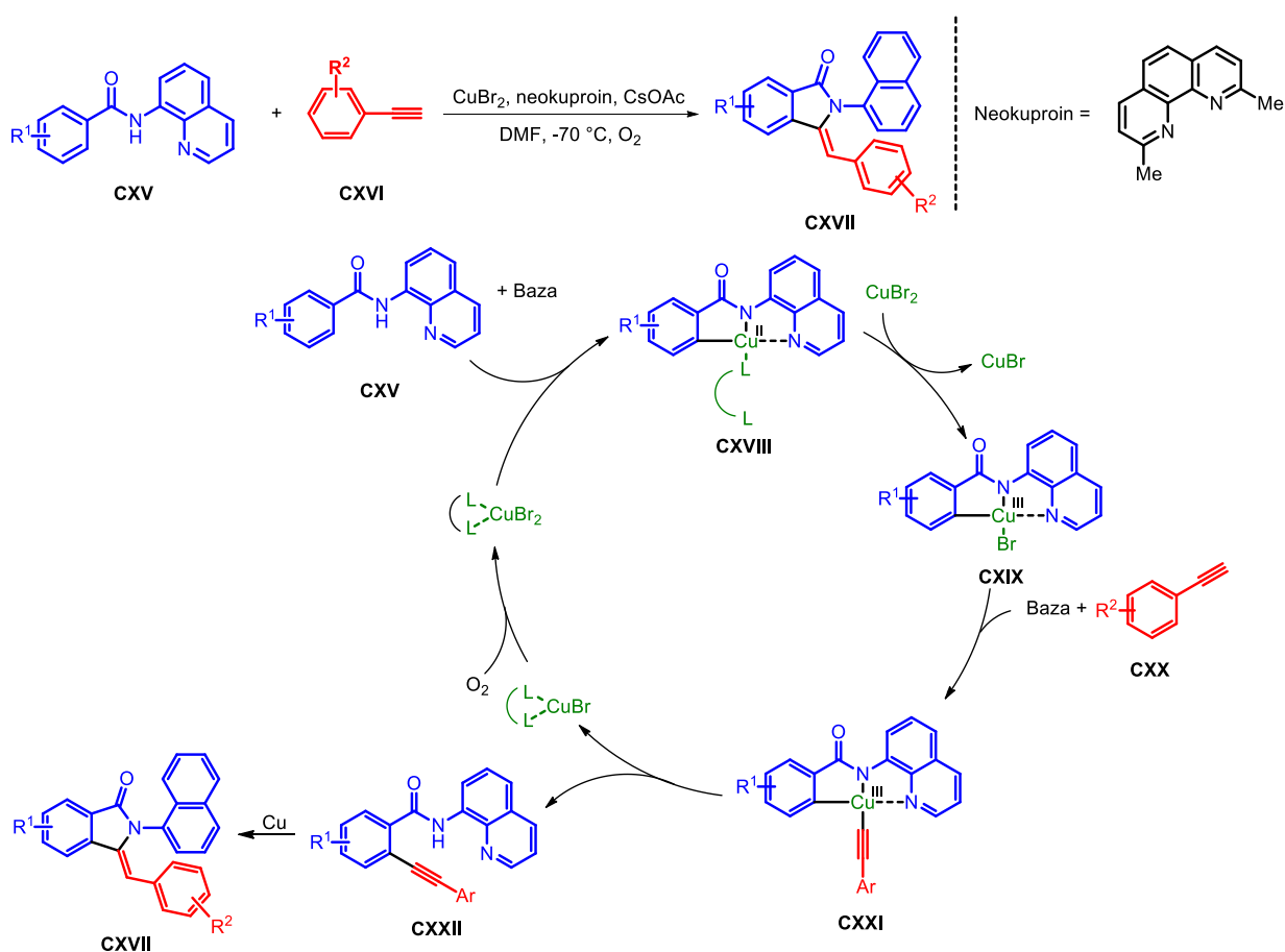
Shema 20. Anulacija 2-alkinilbenzamida katalizirana s CuBr 2 u aerobnim uvjetima
