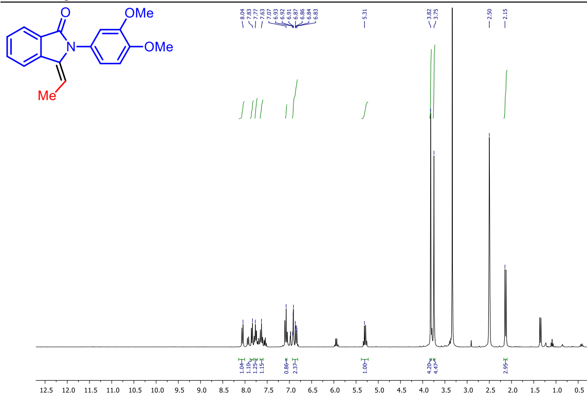
Slika D73. ^1\text{H} NMR spektar ( E )-2-(3,4-dimetoksifenil)-3-etilidenizoidolinona ( E -2p)
