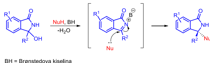
Shema 47. Nastajanje elektrofilnog N -acilketimina
