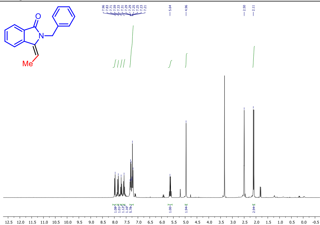
Slika D49. 1 H NMR spektar ( E )-2-benzil-3-etilidenizindolinona ( E-2g )
