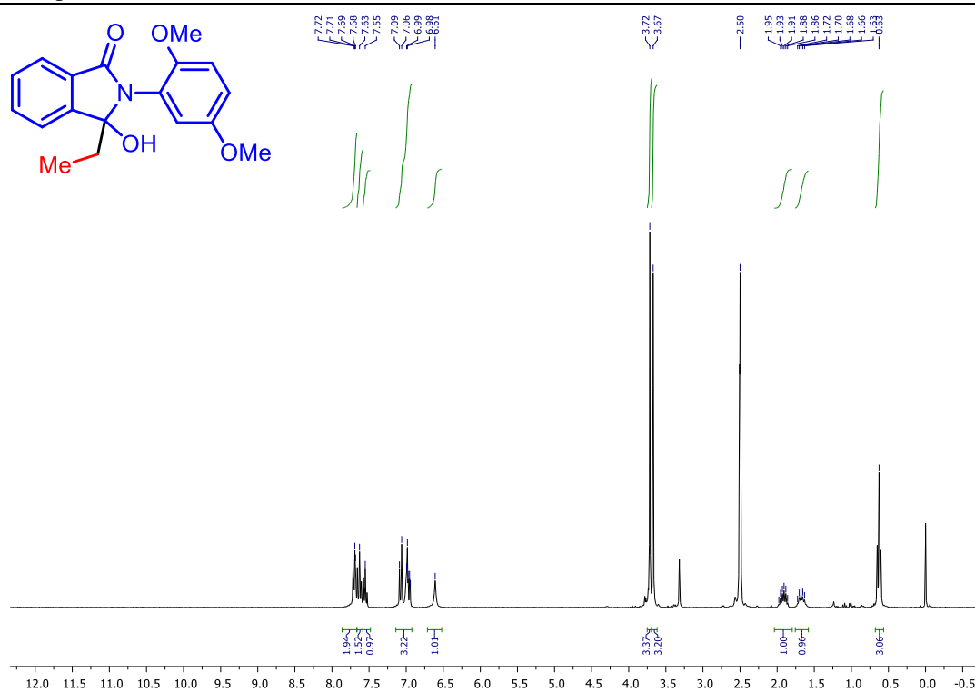
Slika D20. 1 H NMR spektar 2-(2,5-dimetoksifenil)-3-etil-3-hidroksiizoinolinona ( 10 )
