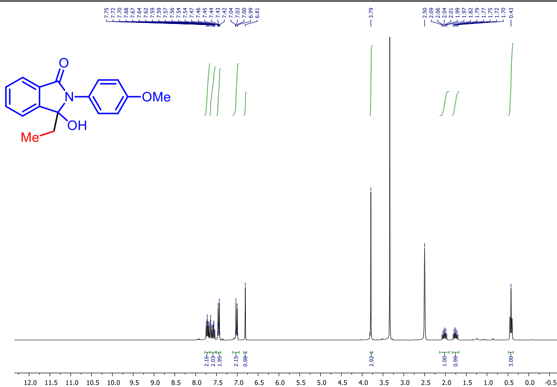
Slika D30. 1 H NMR spektar 3-etil-3-hidroksi-2-(4-metoksifenil)izoinolinona (1t)
