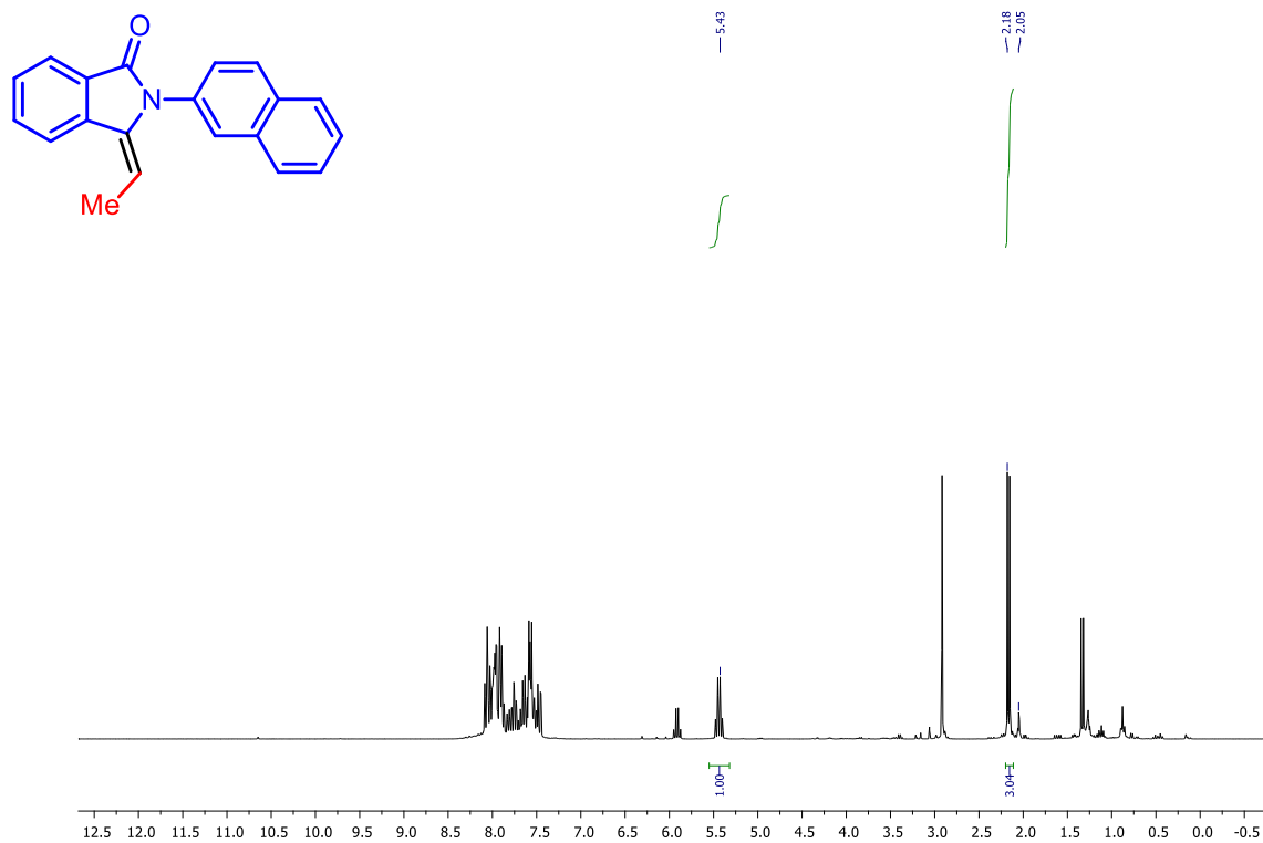
Slika D81. ^1\text{H} NMR spektar ( E )-3-etiliden-2-(naftalen-2-il)izoindolinona ( E - 2r )
