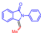
Slika 33. Strukturna formula molekule spoja E-2j
