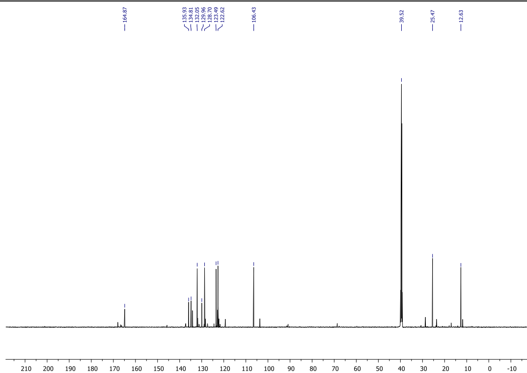
Slika D47. ^{13}\text{C} NMR spektar ( E )-3-etiliden-2-metilizoindolinona ( E -2f)
