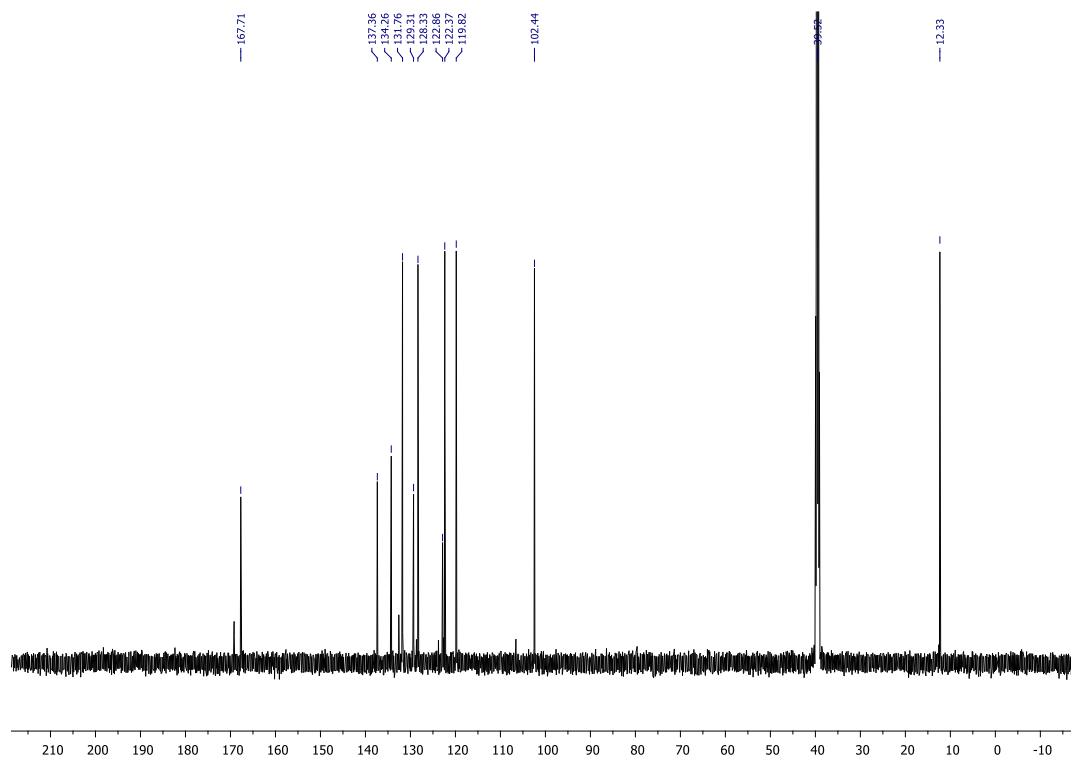
Slika D35. 13 C NMR spektar (Z)-3-etilidenizoindolinona (2a)
