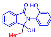
Slika 15. Strukturna formula molekule spoja 1k
