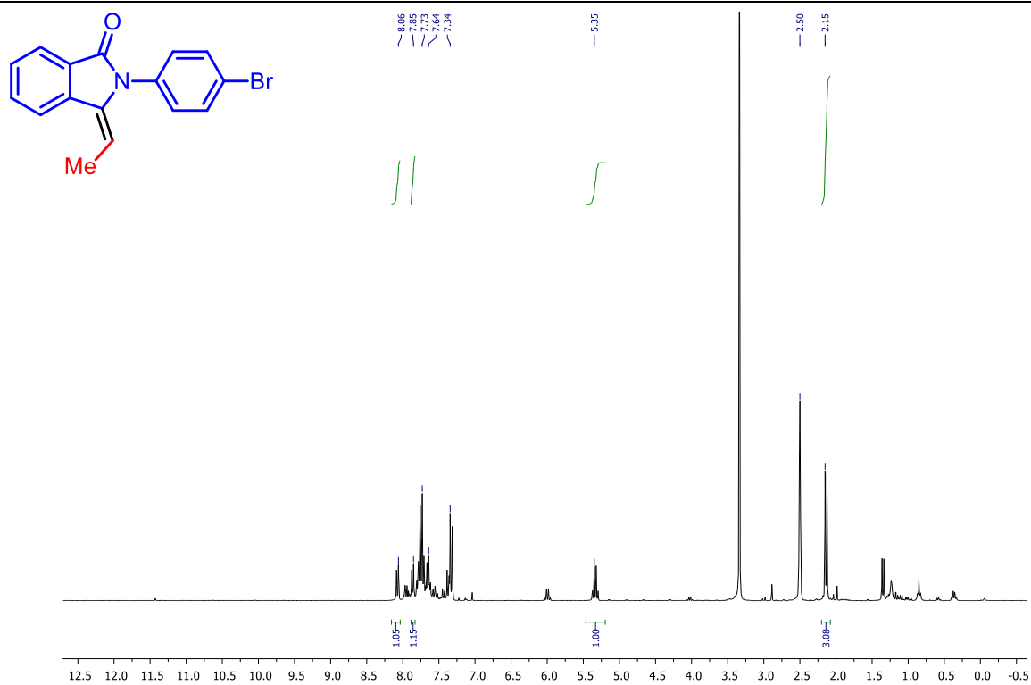
Slika D85. ^1\text{H} NMR spektar ( E )-2-(4-bromfenil)-3-etilidenizoidolinona ( E -2s)
