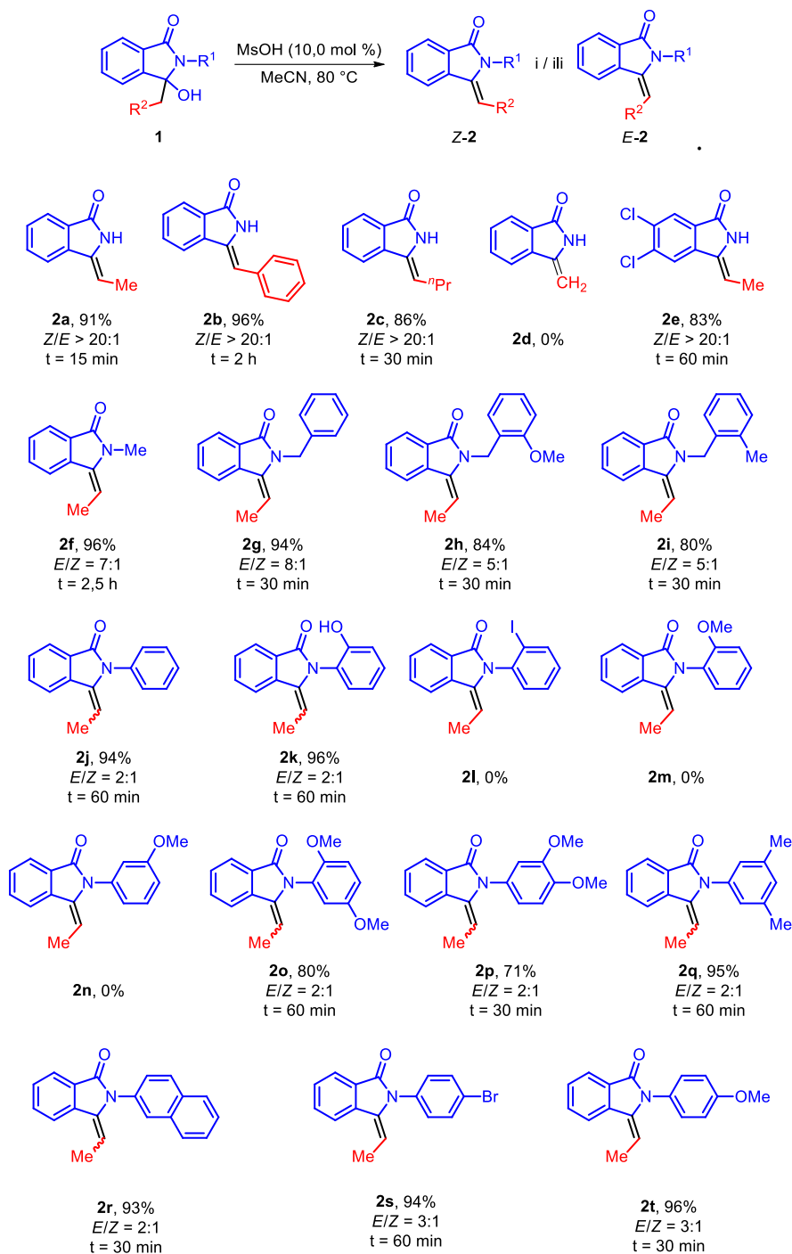
Slika 45. Priprava 3-alkilidenizindolinona
