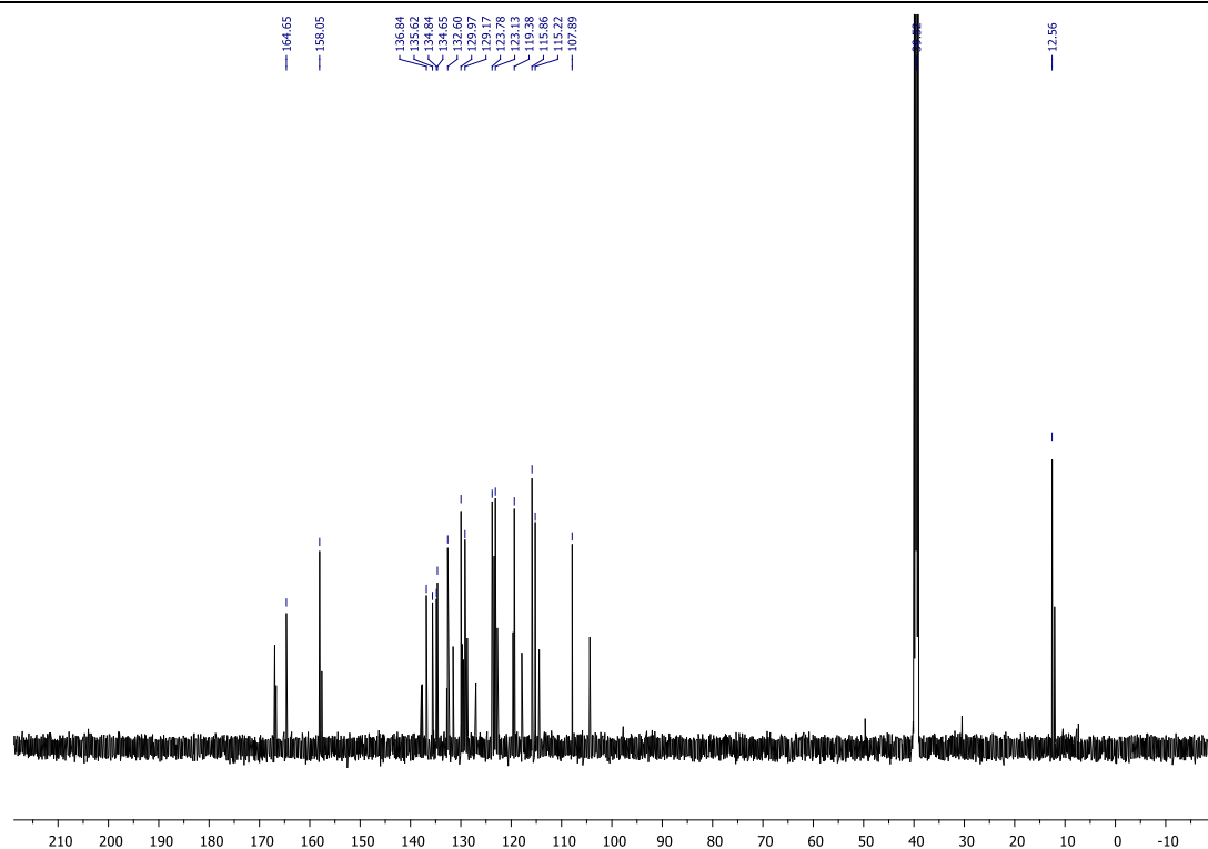
Slika D67. ^{13}\text{C} NMR spektar ( E )-3-etiliden-2-(2-hidroksifenil)izoindolinona ( E -2k)
