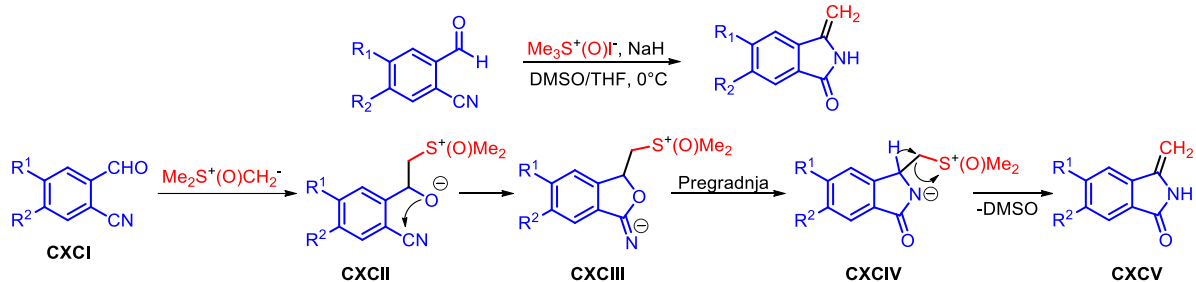
Shema 36. Reakcija i mehanizam formiranja 3-alkil- ili 3-arilmetilidenizoidol-1-ona iz 2-formilbenzonitrila i dimetiloksosulfonijevog metilida
