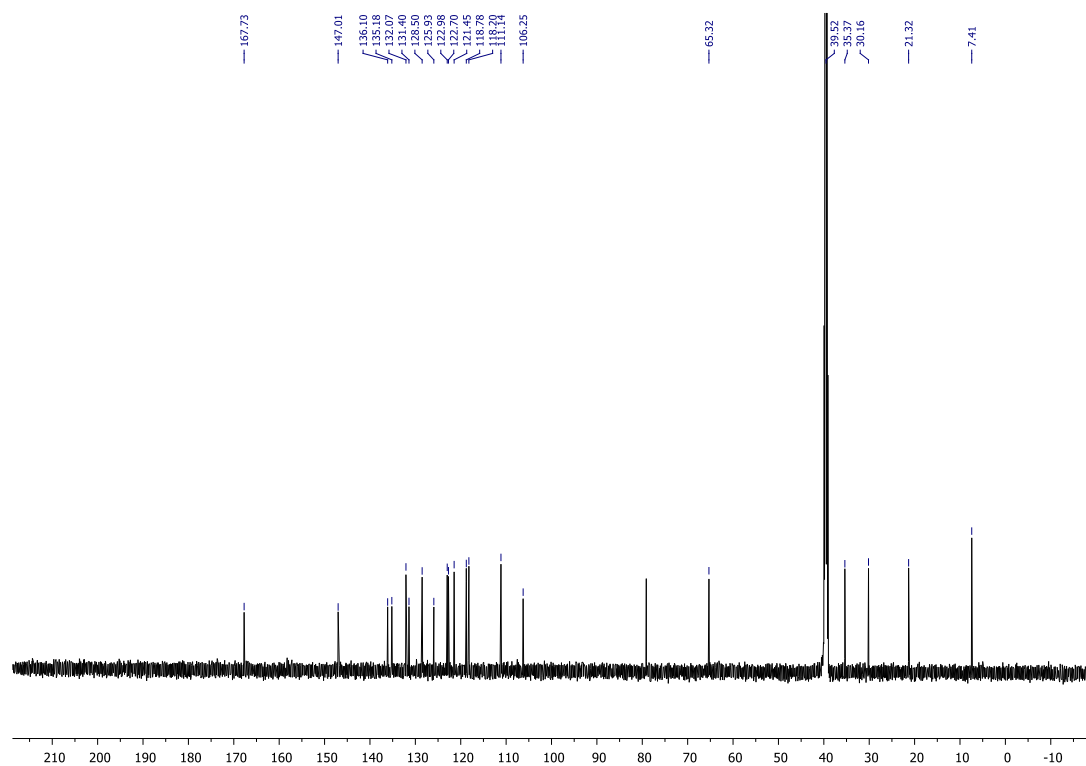
Slika D95. 13 C NMR spektar 13b-etil-7,8,13,13b-tetrahidro-5 H -benzo[1,2]indolizino[8,7- b ]indol-5-ona ( 4 )
