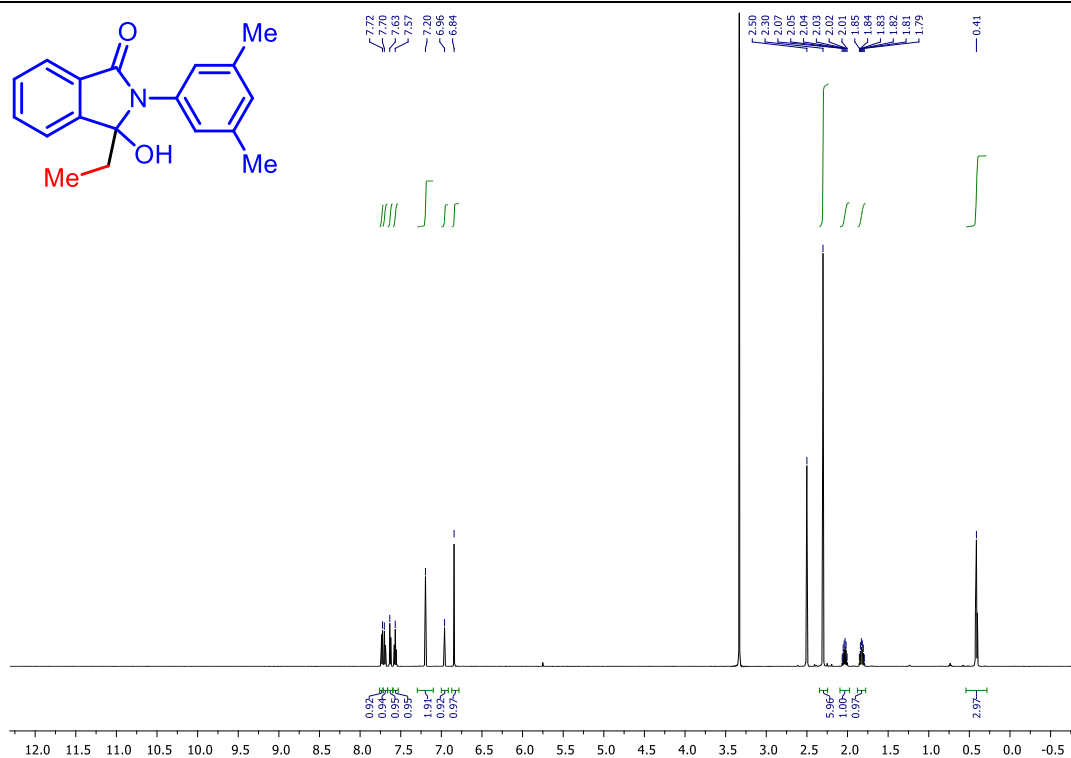
Slika D24. 1 H NMR spektar 2-(3,5-dimetilfenil)-3-etil-3-hidroksiizoinolinona ( 1q )
