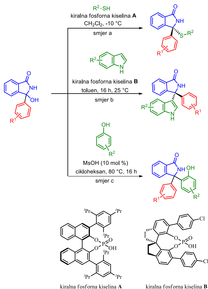
Shema 43. Mogući produkti kiselinom kataliziranih reakcija 3-aril-3-hidroksiizoindolinona.
