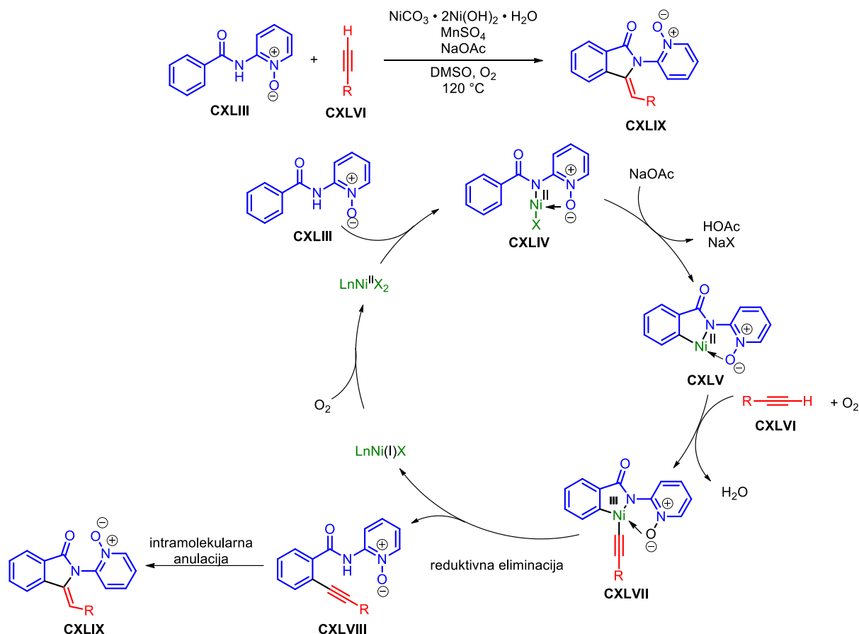
Shema 25. Priprava 3-alkil/aril-metilenizoidolinona alkiniliranjem 2-benzamidopiridin-1-oksida uz katalizu s NiCO_3 \cdot 2 Ni(OH)_2 \cdot H_2O
