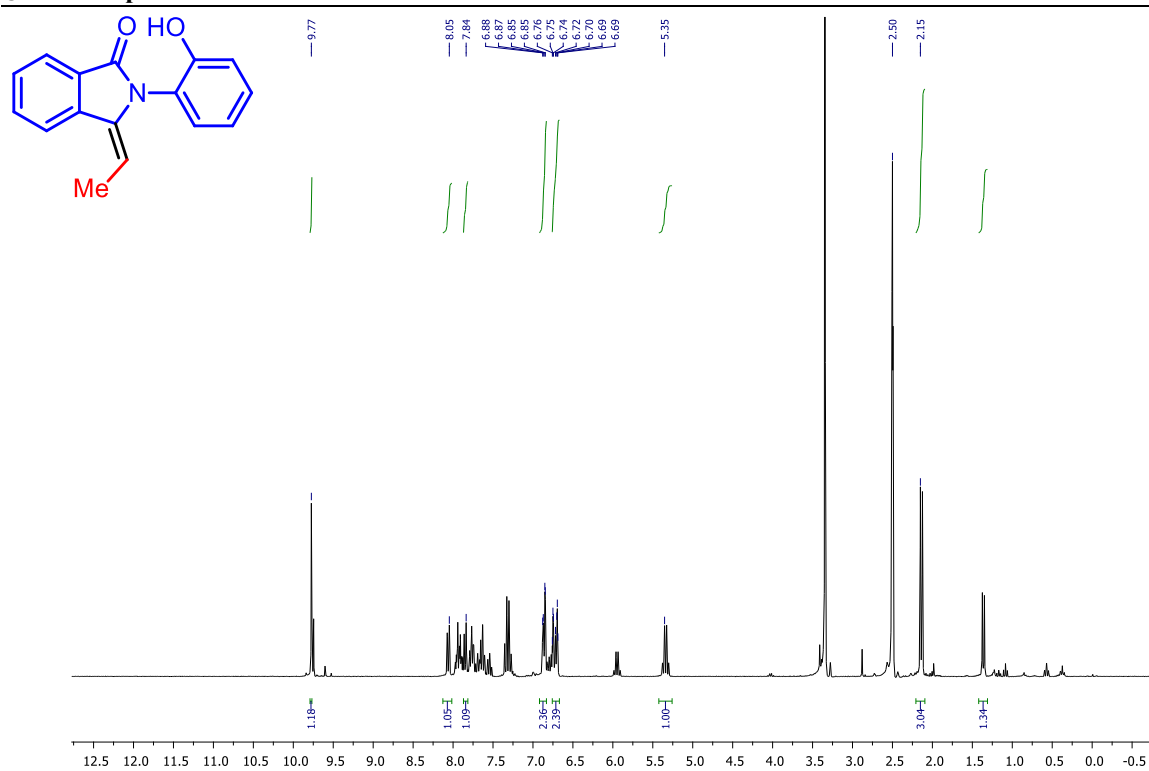
Slika D65. 1 H NMR spektar ( E )-3-etiliden-2-(2-hidroksifenil)izoindolinona ( E -2k)
