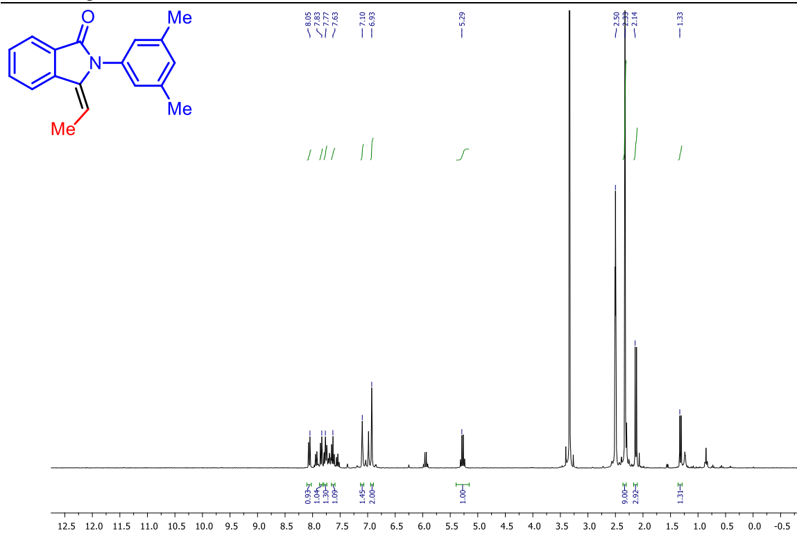
Slika D77. ^1\text{H} NMR spektar ( E )-2-(3,5-dimetilfenil)-3-etilidenizindolinona ( E -2q)
