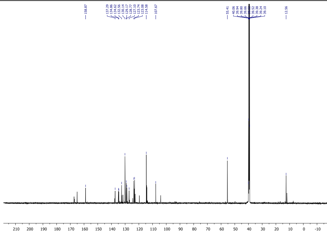
Slika D91. 13 C NMR spektar ( E )-3-etiliden-2-(4-metoksifenil)izoindolinona ( E -2t)
