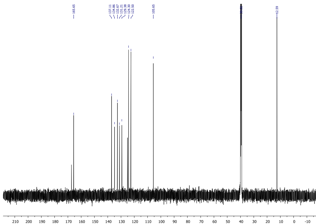
Slika D43. 13 C NMR spektar (Z)-5,6-diklor-3-etilidenizindolinona (Z-2e)
