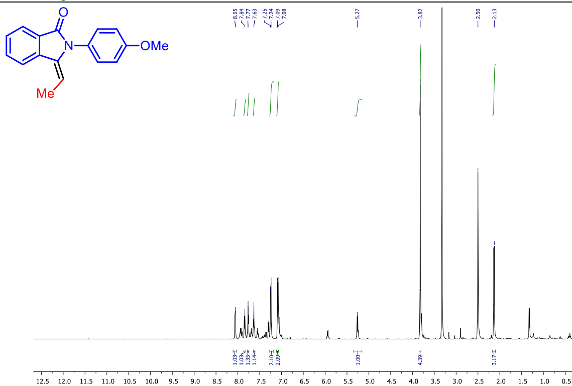
Slika D89. 1 H NMR spektar ( E )-3-etiliden-2-(4-metoksifenil)izoindolinona ( E -2t)
