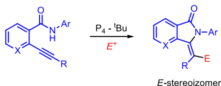
Shema 31. Priprava E -enamida intramolekularnom ciklizacijom
