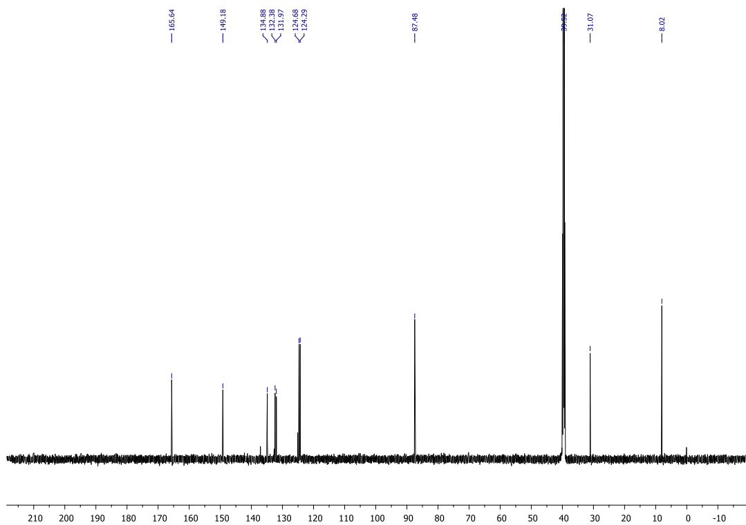
Slika D3. ^{13}\text{C} NMR spektar 5,6-diklor-3-etil-3-hidroksiizoinolinona ( 1e )
