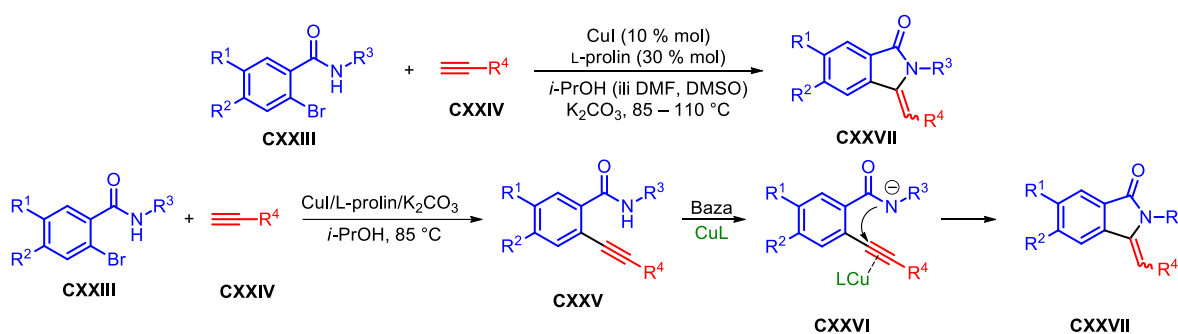
Shema 21. CuI/L-prolin kataliza u formiranju 3-metilenizoidolinona
