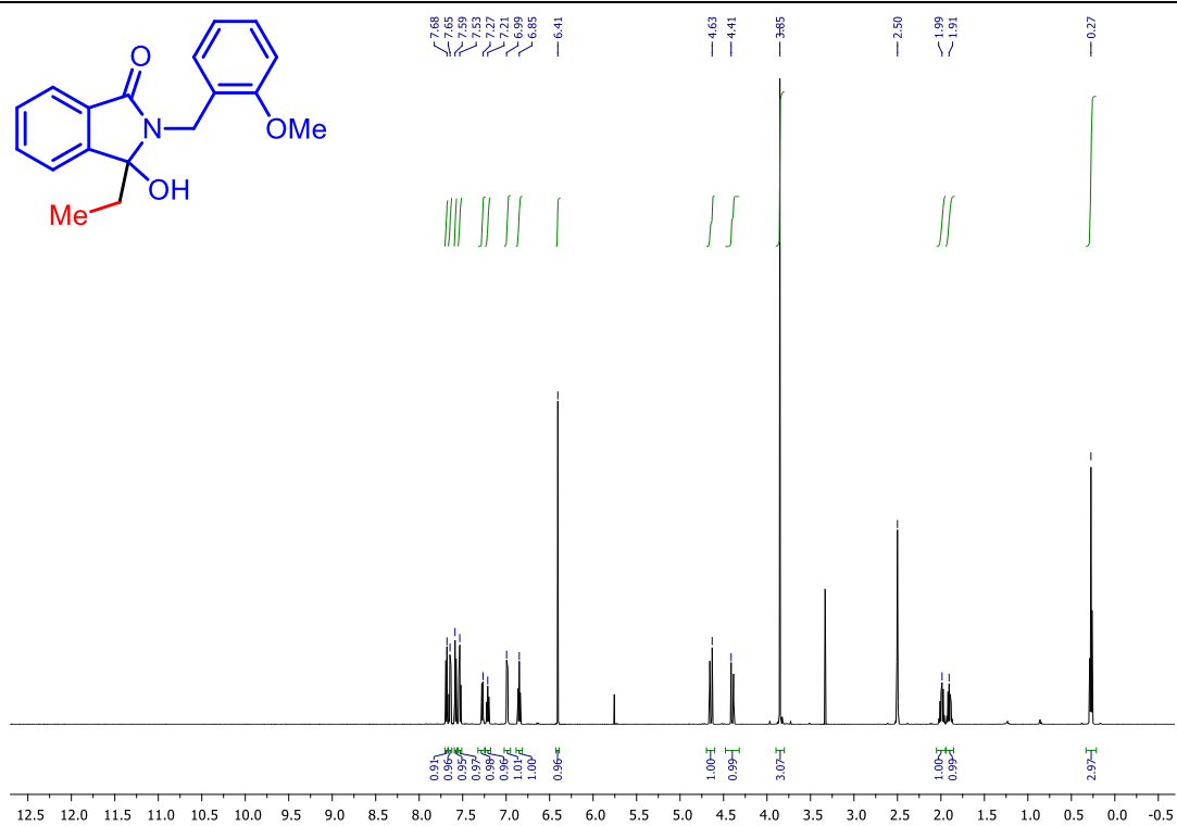
Slika D8. 1 H NMR spektar 3-etil-3-hidroksi-2-(2-metoksibenzil)izoindolinona ( 1h )
