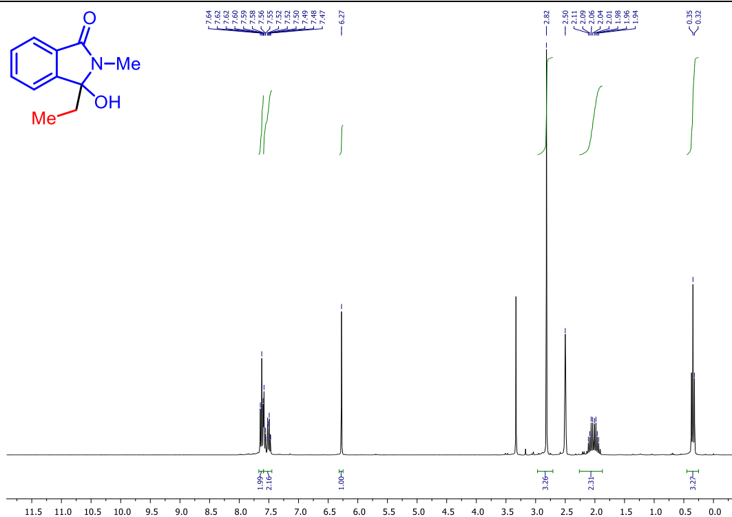
Slika D4. 1 H NMR spektar 3-etil-3-hidroksi-2-metilizoindolinona (1f)
