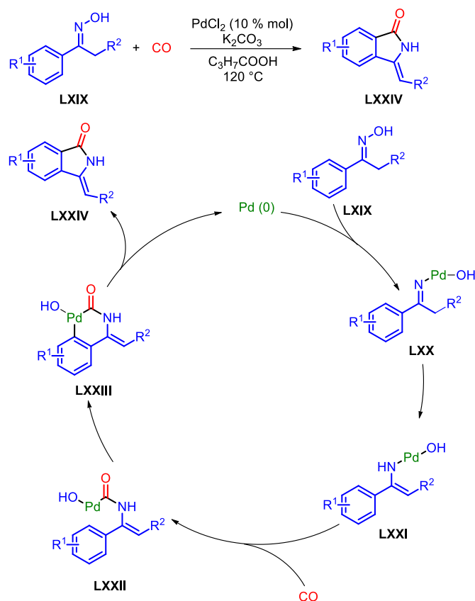
Shema 11. Reakcija i katalitički ciklus priprave raznih N -nezaštićenih 3-metilenizoidolinon derivata katalizom paladijev(II) kloridom
