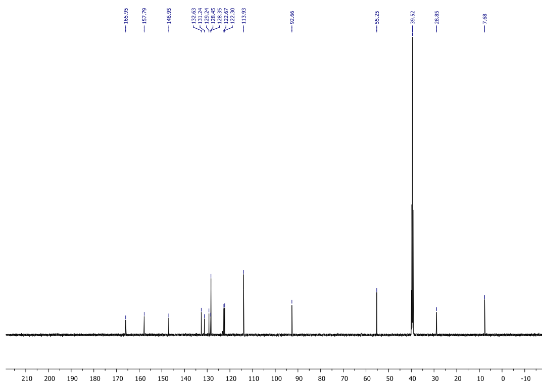
Slika D31. 13 C NMR spektar 3-etil-3-hidroksi-2-(4-metoksifenil)izoinolinona (1t)
