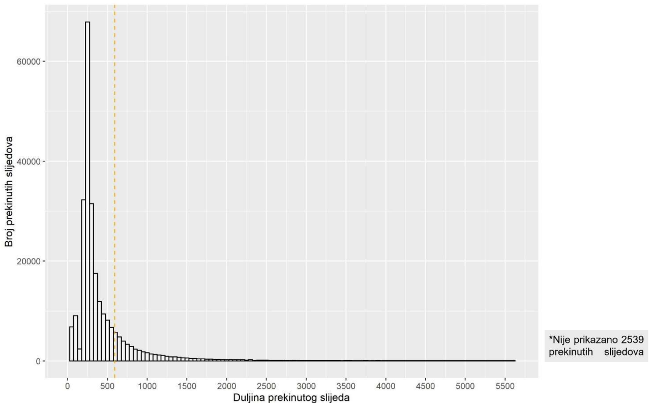
Slika 6 Histogram duljina sastavljenih metagenomskih prekinutih sljedova. Prikazan je 99. percentil duljina. Narandčastom iscrtkanom linijom označena je prosječna duljina prekinutoga slijeda.
