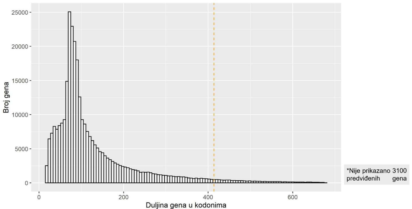
Slika 8 Histogram duljina gena (u kodonima) koji su predviđeni iz skela metagenoma pomoću programa MetaGeneMark; prikazan je 99. percentil duljina. Veličina koraka histograma je 6. Narančastom iscrtkanom linijom označena je prosječna duljina predviđenih gena.
