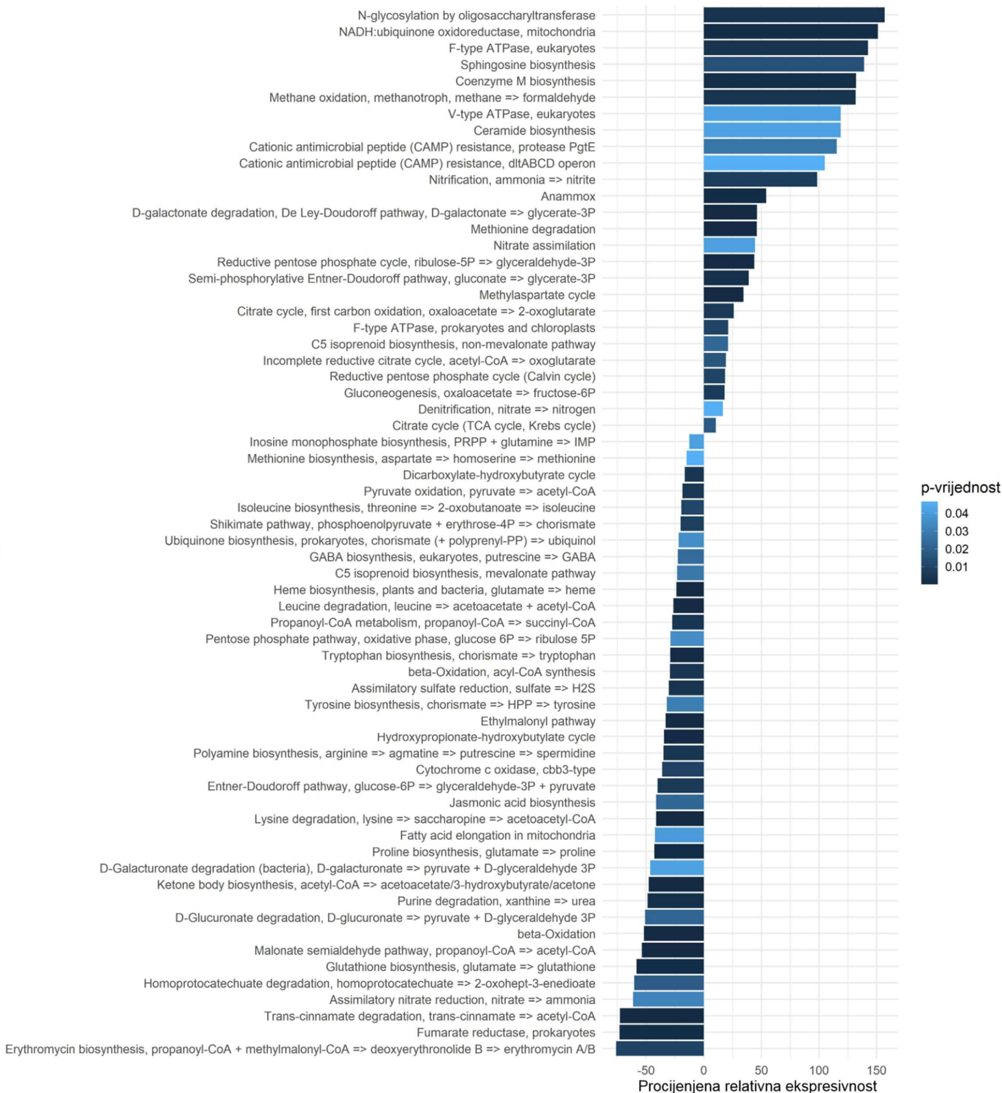
Slika 13 Graf relativne ekspresivnosti kategorija KEGG modula gena grupiranih po kategoriji. Relativna ekspresivnost za svaki modul x definirana je kao E_x u jednačbi (5). Prikazani su samo rezultati s p < 0,05 .
