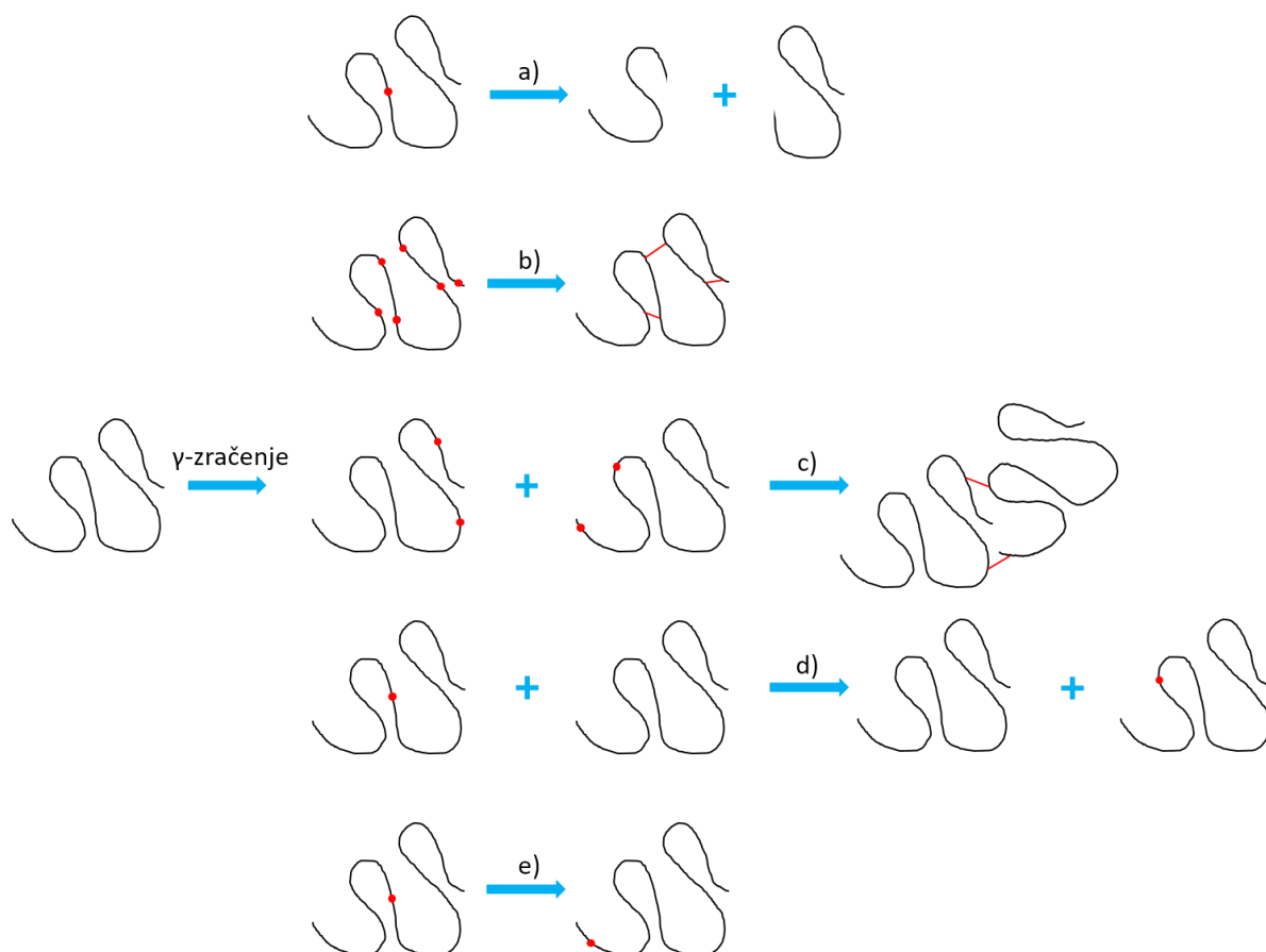
Slika 19. Reakcije makroradikala: a) degradacija ili cijepanje lanaca, b) unutarmolekulska umrežavanje, c) međumolekulska umrežavanje, d) međumolekulska disproporcioniranje, e) unutarmolekulska disproporcioniranje; crvene točke predstavljaju makroradikale, a crvene linije novoformirane veze (prilagođeno prema referenci 60)
