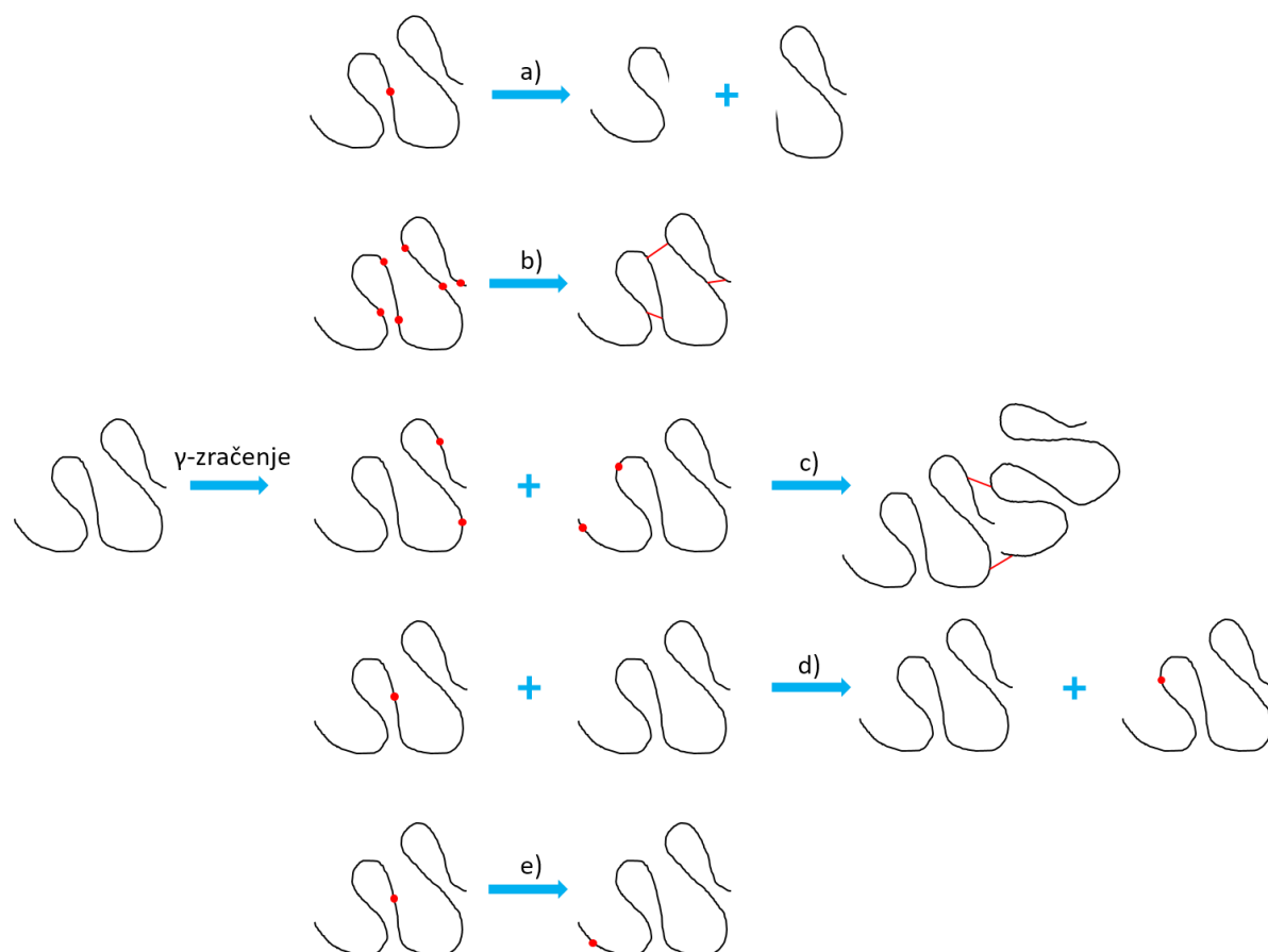
Slika 19. Reakcije makroradikala: a) degradacija ili cijepanje lanca, b) unutarmolekulska umrežavanje, c) međumolekulska umrežavanje, d) međumolekulska disproportioniranje, e) unutarmolekulska disproportioniranje; crvene točke predstavljaju makroradikale, a crvene linije novoformirane veze (prilagođeno prema referenci 60)
