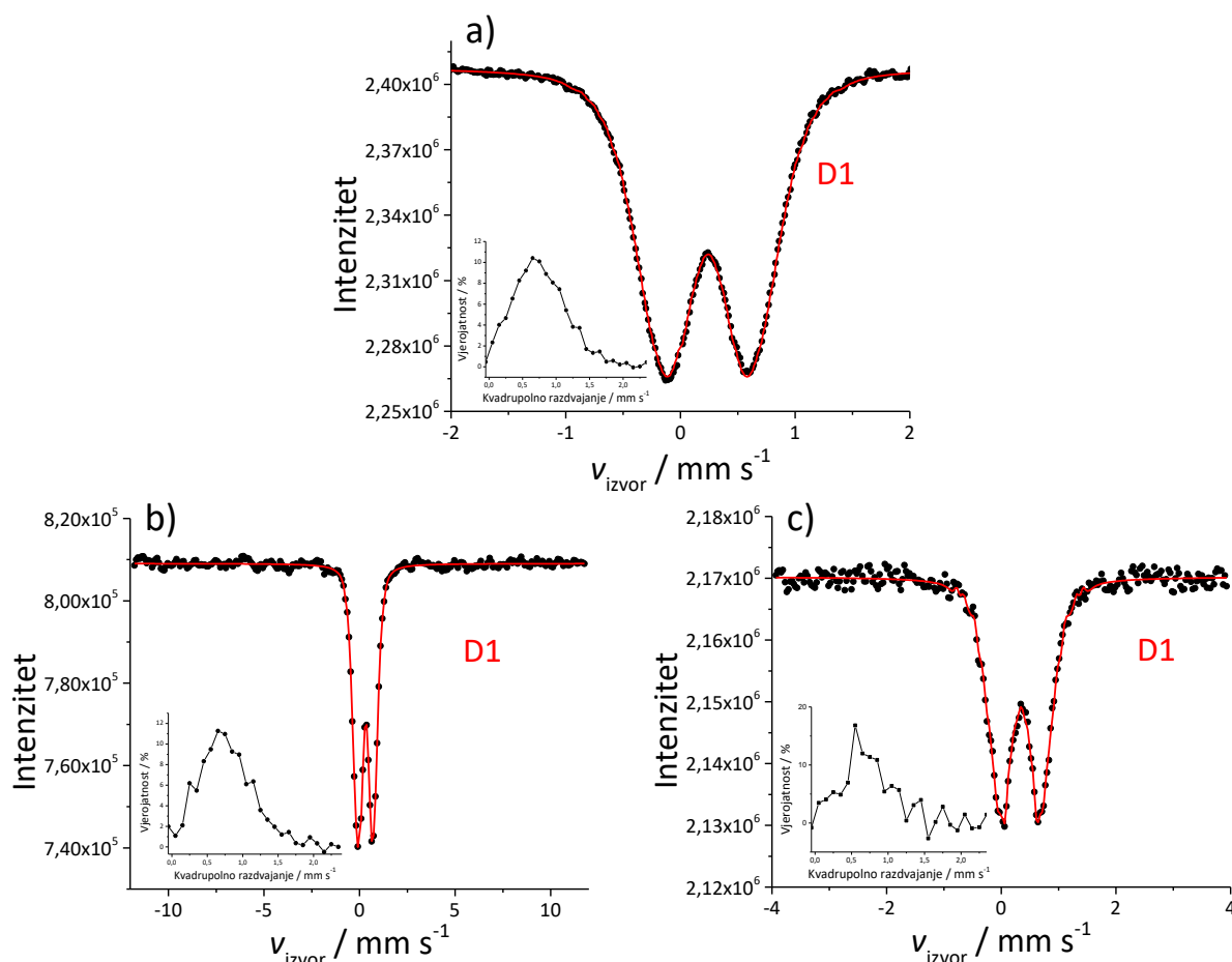
Slika 37. Mössbauerovi spektri nezračenog uzorka DD2-0, odnosno Fe(III) prekursora, pri sobnoj temperaturi (a) i pri 77 K u formi izoliranog praha (b) i suspenzije (c) (u umetcima su prikazane distribucije kvadrupolnog razdvajanja)
