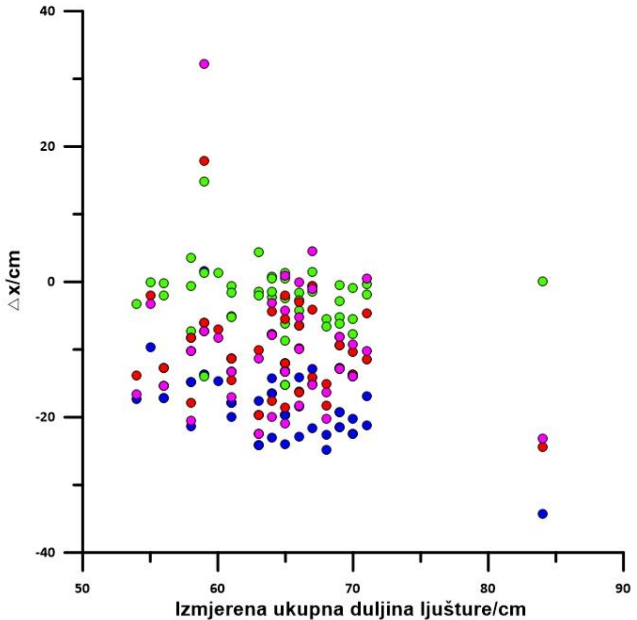
Slika 9. Grafički prikaz razlike između izračunate i izmjerene ukupne dužine školjke ( \Delta x ) za sve četiri jednadžbe za izračun procijenjene ukupne dužine ljušture iz visine nezakopanog dijela ljušture
