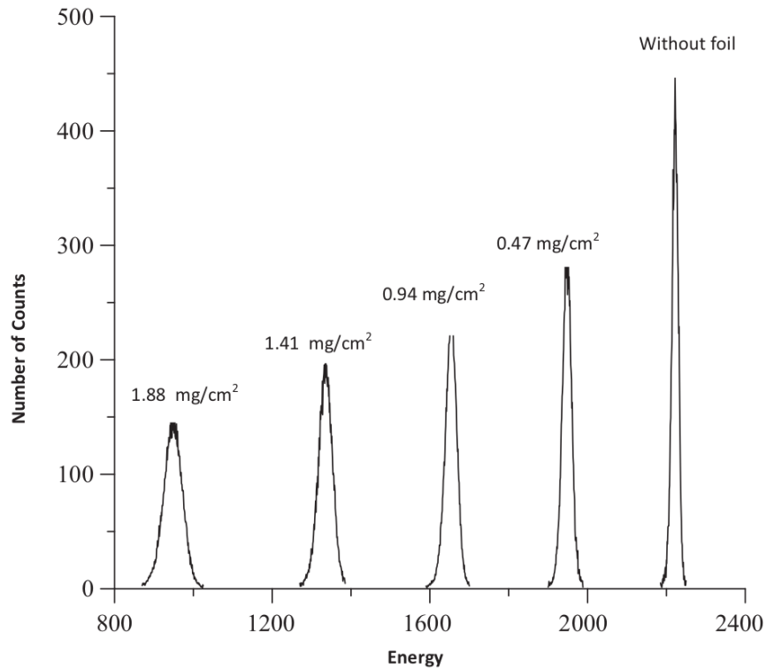
Slika 2.5: Energetski spektri iona kisika energije 30 MeV nakon prolaska kroz membrane PET polimera različitih debljina. Preuzeto iz [22].
