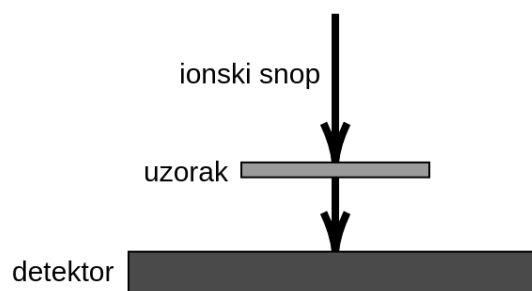
Slika 3.6: Schematski prikaz STIM metode.
