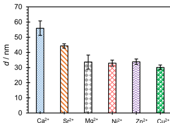
Slika 27. Debljine Si-(PDADMAC/PSS) 5 XCl 2 višesloja priređenog uz kloride različitih dvovalentnih kationa određene pomoću AFM-a.
