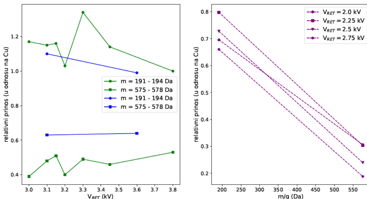
Slika 5.3: Relativni prinos cijelih molekula ftalocijanina ( m = 575-578 Da) i njegovih fragmenata ( m = 191-194 Da) za različite iznose RETARD napona, za napon ekstrakcije 4.5 kV (lijevo) i napon ekstrakcije 3 kV (desno). Prinos bakra (fragmenata molekule ftalocijanina mase 63 i 65) iznosi jedan. Na slici lijevo zelene točke su za vrijednosti REFLECT napona 4.5 kV i napona Einzel leće 1.7 kV, a plave točke su za vrijednosti napona 4.6 kV i 2.4 kV, redom.
