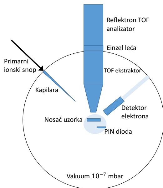
Slika 4.2: Shematski prikaz kapilarne mikroprobe za MeV TOF-SIMS s reflektrom TOF analizatorom (lijevo). Slika komore izvana (desno).
