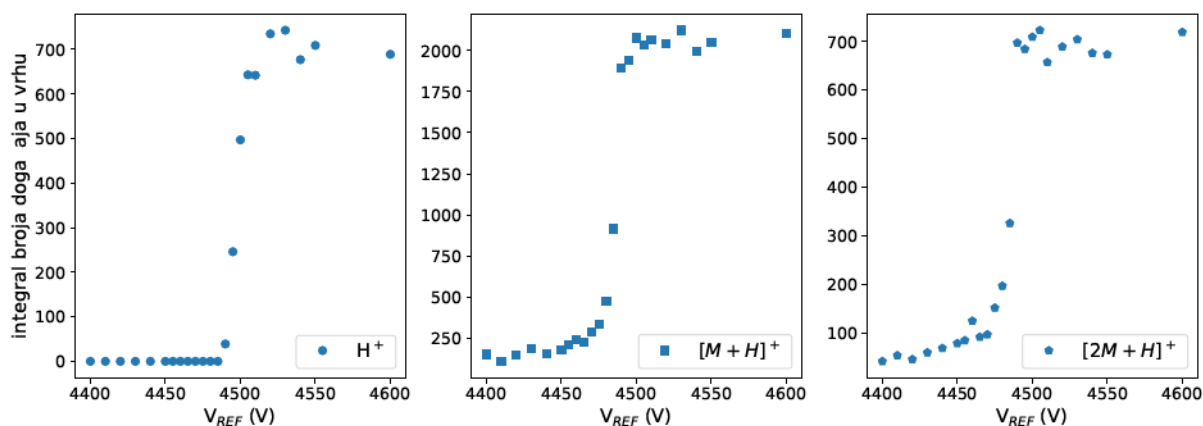
Slika 5.2: Utjecaj napona reflektрона na prinos za odabrane vrhove u spektru leucina. Mjerenje je napravljeno u transmisivskom načinu rada, s naponom ekstrakcije 4.5 kV. Na RETARD kontakt nije doveden vanjski napon. Korišten je primarni snop 14 MeV \text{Cu}^{4+} struje \sim 350 Hz.
