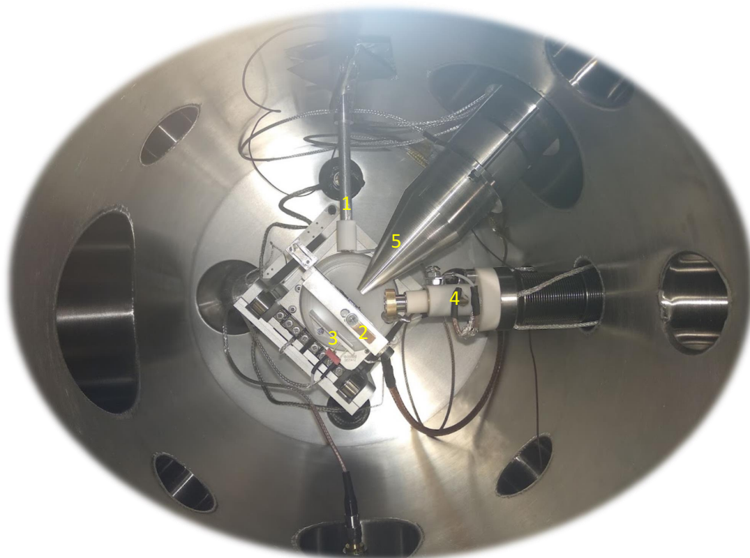
Slika 4.3: Fotografija kapilarne mikroprobe za MeV TOF-SIMS s reflektornim TOF analizatorom. Oznake: 1 - metalni nosač unutar kojeg se nalazi staklena kapilara, 2 - nosač uzorka, 3 - dioda, 4 - nosač na kojem se nalazi elektronski detektor, 5 - ekstraktor.
