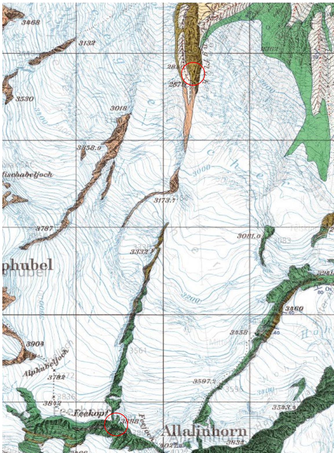
Slika 2. Geološka karta sa naznačenim lokalitetima Feeskopf i Längfluh
