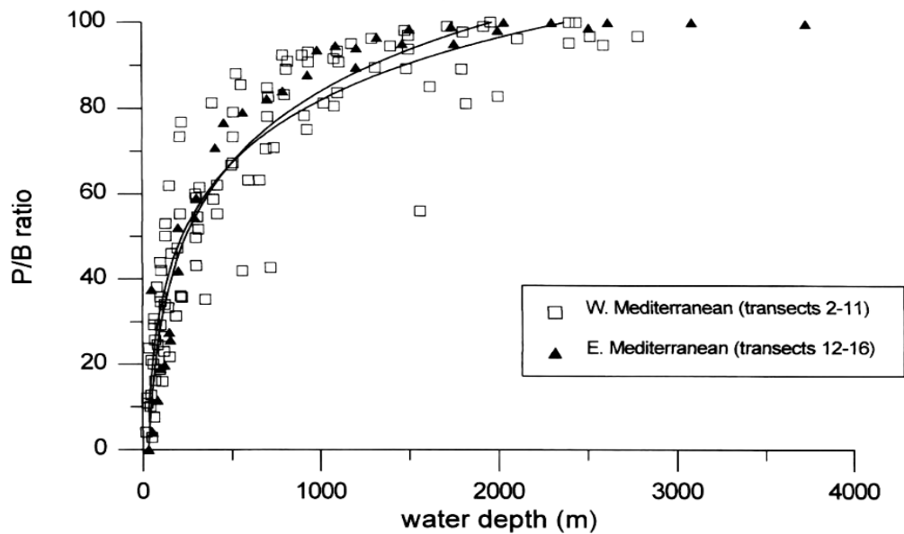
Slika 15. Udio planktonskih foraminifera u odnosu na dubinu vode u zapadnom i istočnom Mediteranu prema dubini okoliša (Wright, 1980).
