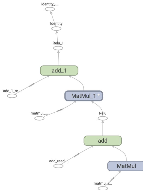
Slika 4.2: Primjer grafa u biblioteci tensorflow iz [2].
