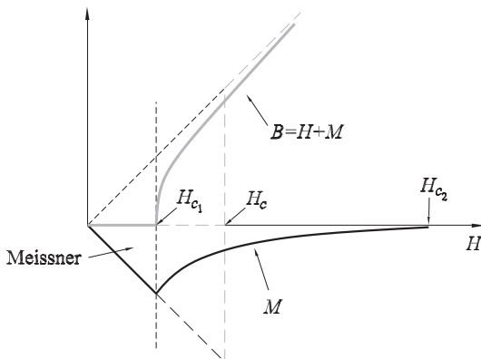
Slika 7. Prosječno polje B = M + H kroz supravodič u funkciji vanjskog polja H , te prosječnog magnetski moment M supravodiča II. vrste.
