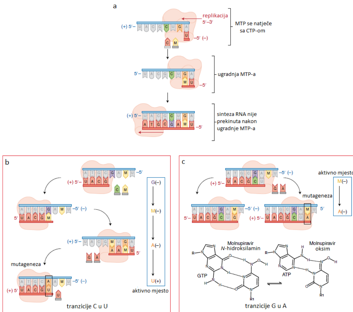
Slika 8. Shema puta mutageneze molnupiravirom. a MTP se natječe uglavnom s CTP-om za ugradnju nasuprot G. b Shematski prikaz tranzicije C u U. c Shematski prikaz tranzicije G u A. Preuzeto i prilagođeno prema izvoru 10.
