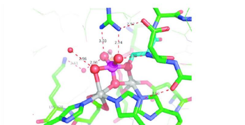
Slika 3. Prikaz vanadata u aktivnom mjestu alkalne fosfataze E. coli 11 (Izvor: T. W. Elliot, N. Miti, L. R. Gahan, L. W. Guddat, G. Schenk, J. Braz. Chem. Soc. , 2006, 17 , 1558)
