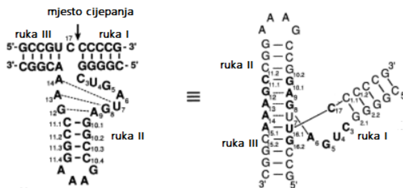
Slika 3. Sekundarna struktura čekičastog ribozima (lijevo) i prikaz čekičastog ribozima temeljen na kristalografskim podacima dobivenih difrakcijom X-zraka (desno). Preuzeto i prilagođeno prema 17
