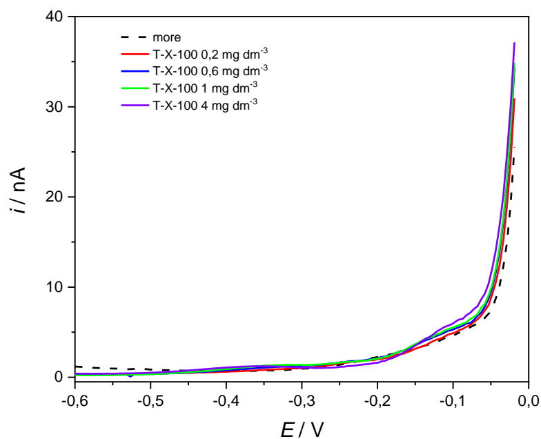
Slika 4.5. DPASV voltamogrami T-X-100 pri različitim koncentracijama u modelnom elektrolitu UVSW. Uvjeti mjerenja: E_a = -0,6 V, t_a = 60 s.
