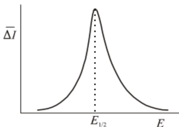
Slika 2.5. Izgled diferencijalnog pulsno voltamograma. 39
