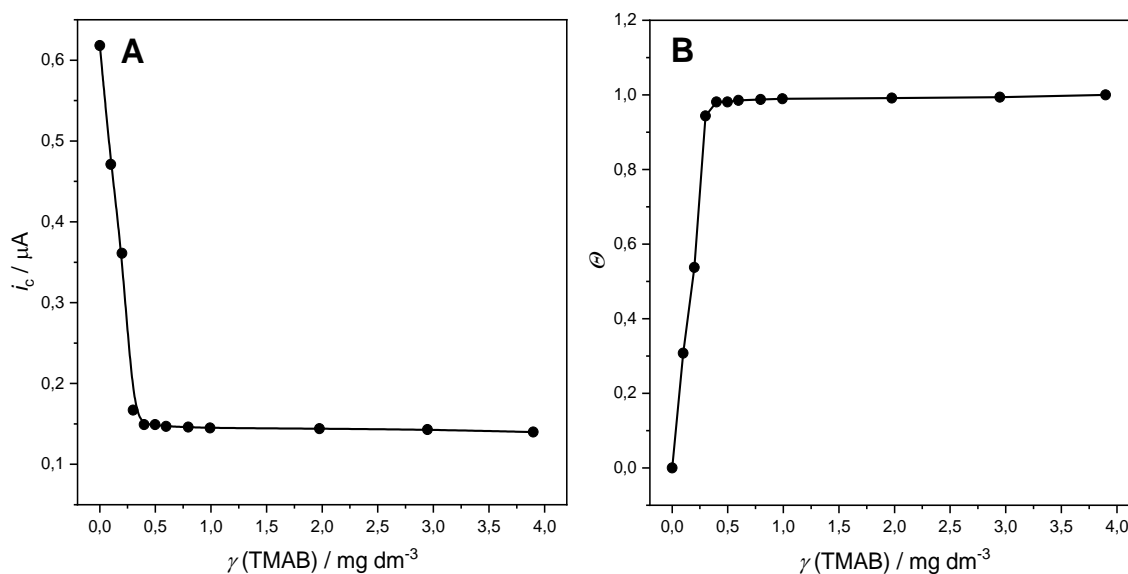
Slika 4.12. A) Sniženje kapacitetne struje dodatkom TMAB. B) Adsorpcijska izoterma TMAB. Uvjeti mjerenja: E_a = -0,6 \text{ V} , t_a = 60 \text{ s} .
