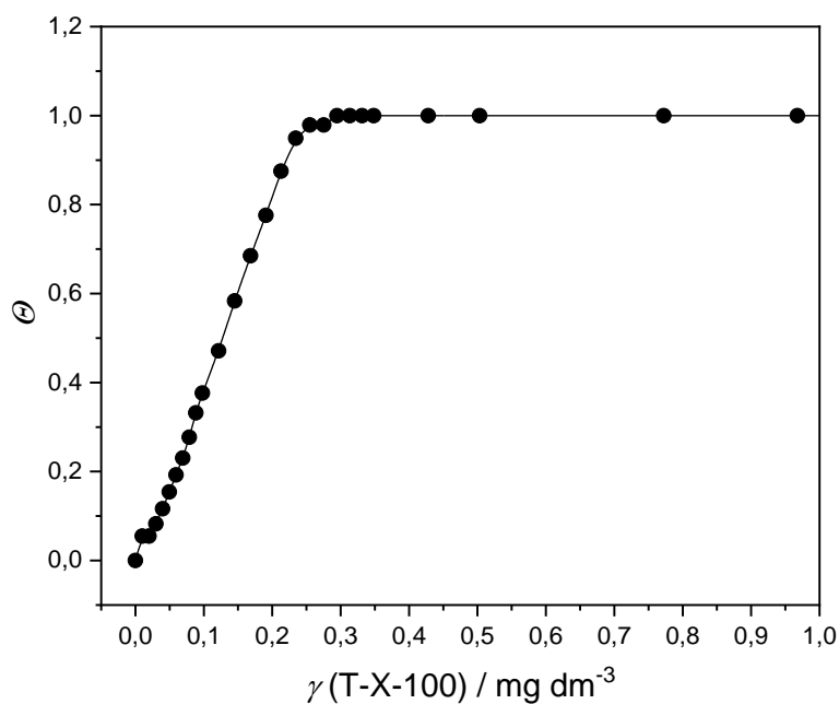
Slika 4.4. Adsorpcijska izoterma T-X-100. Uvjeti mjerenja: E_a = -0,6 V, t_a = 60 s.
