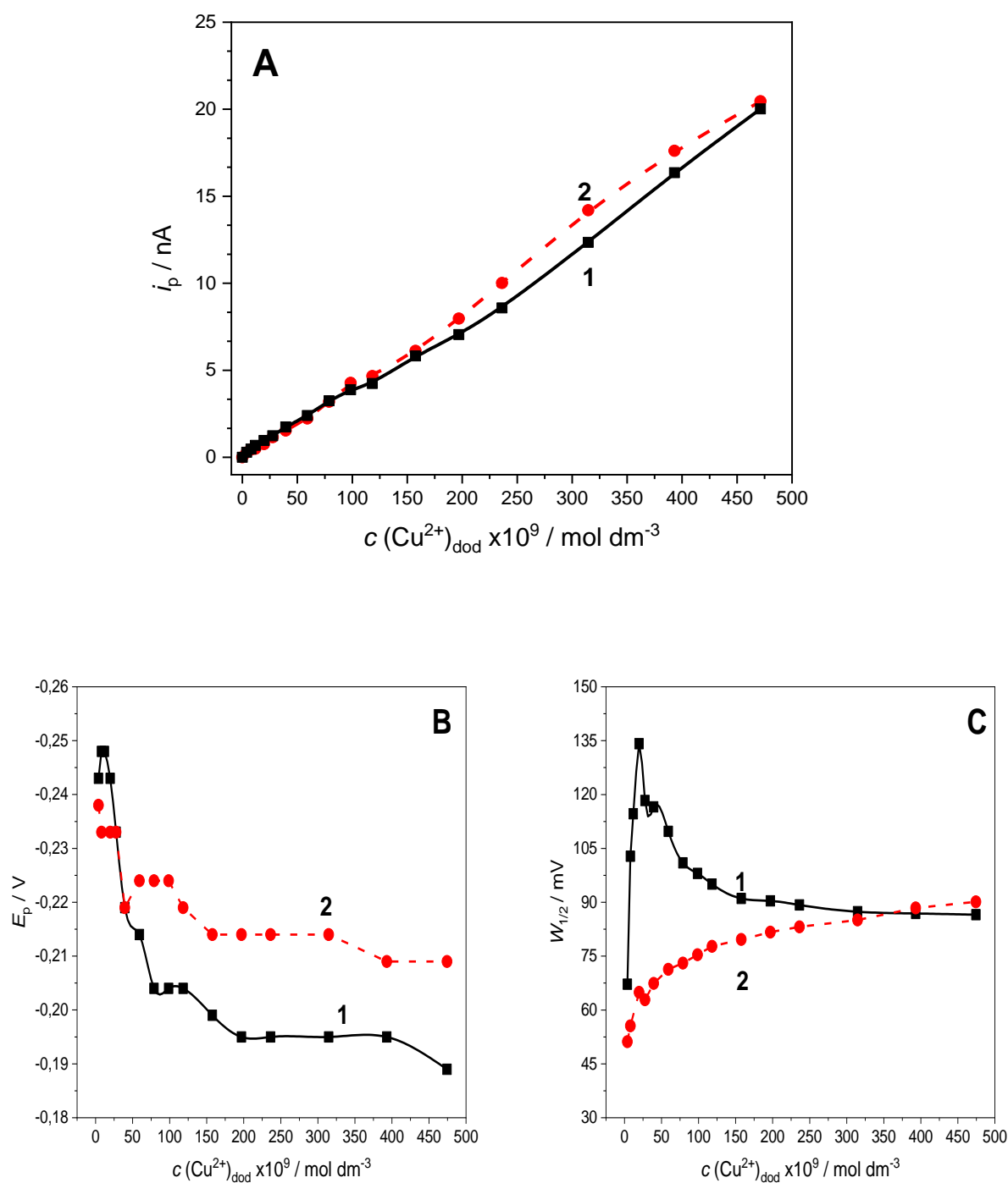
Slika 4.57. Podaci dobiveni analizom pika \text{Cu}^{2+} pri rastućoj koncentraciji \text{Cu}^{2+} -iona u otopini FA \gamma = 1 \text{ mg dm}^{-3} : A) titracijske krivulje kompleksiranja \text{Cu}^{2+} -iona, B) potencijal pika i C) širina pika na polovici visine. Uvjeti mjerenja i oznake krivulja dane su u opisu slike 4.56.
