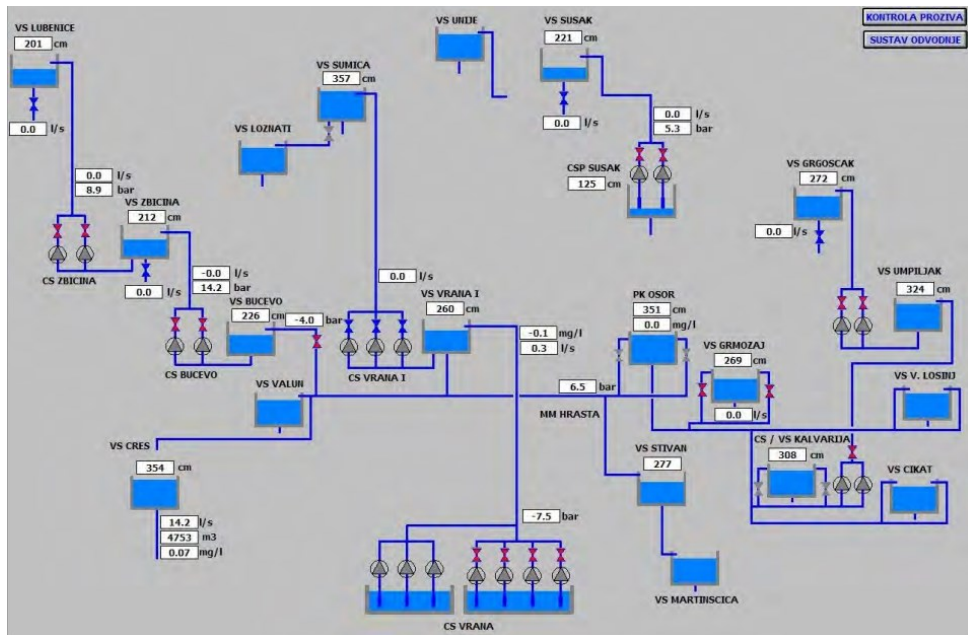
Slika 11. Shematski prikaz vodoopskrbnog sustava Cres a Lošinja
