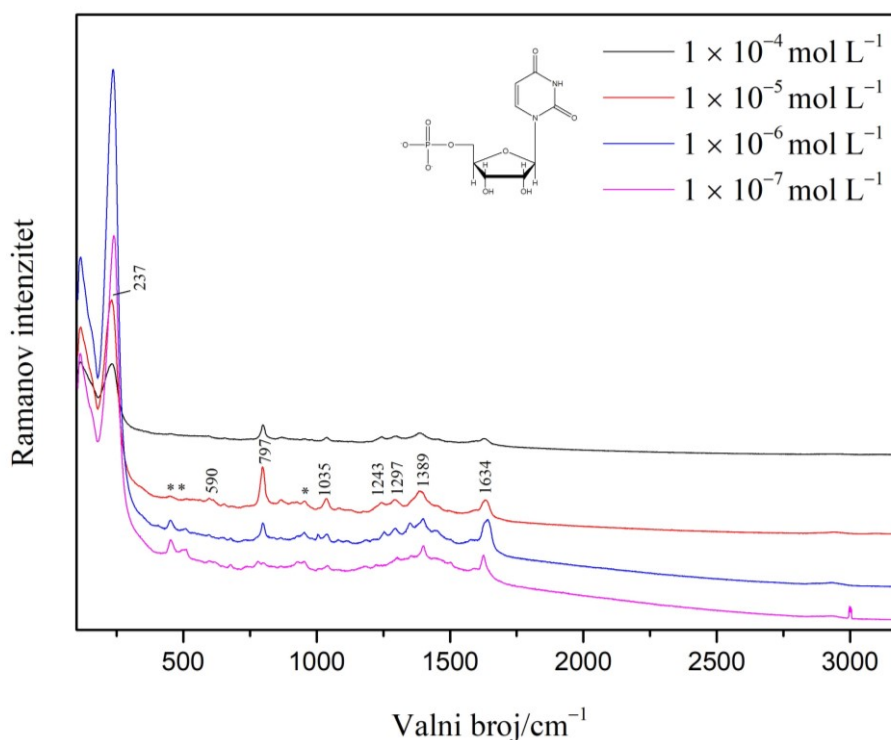
Slika 25. SERS spektri UMP u koloidnoj suspenziji srebra u koncentracijskom području 1 \times 10^{-7} - 1 \times 10^{-4} mol L -1 u prisutnosti agregirajućeg reagensa MgSO 4 (0,1 mol L -1 ) pri valnoj duljini pobude 785 nm i snazi lasera 30 mW. Vrpce koje potječu od citratnih iona označene su s (*). Spektri su razmaknuti zbog preglednosti.
