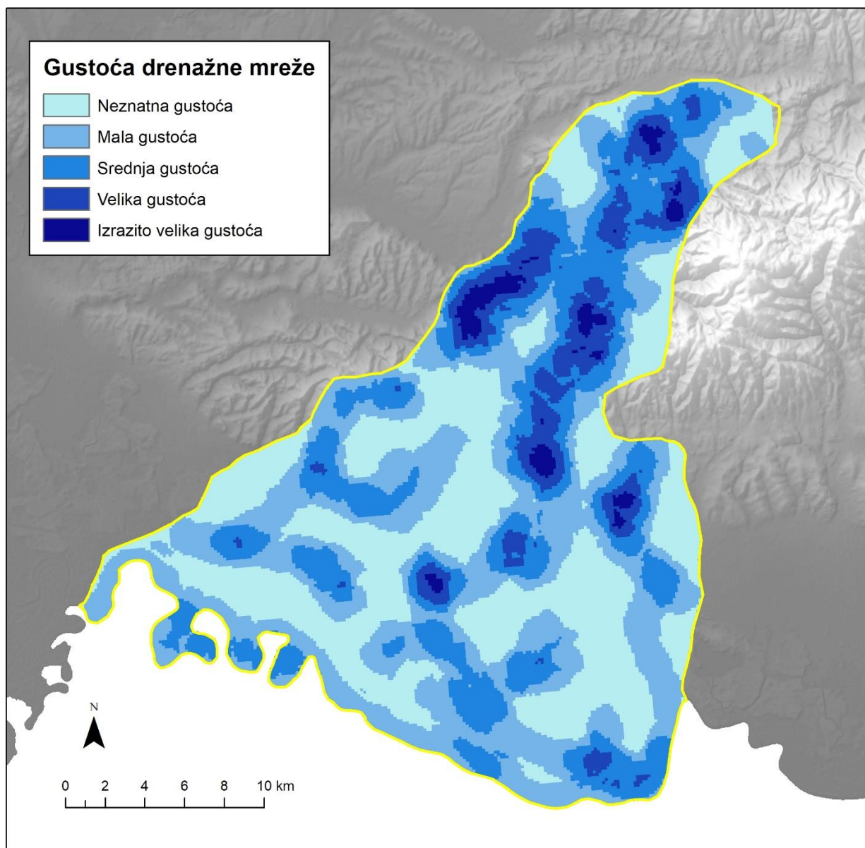
Slika 10. Gustoća drenažne mreže
