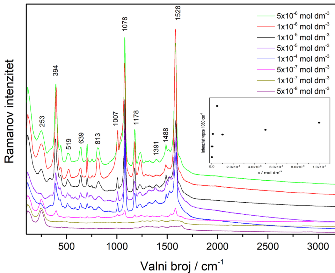
Slika 20. SERS spektri spoja PATF različitih koncentracija ( 5 \times 10^{-8} - 1 \times 10^{-4} mol dm -3 ) u koloidnoj suspenziji zlata snimljeni pri valnoj duljini pobude 785 nm, snaga lasera 3,19 mW
