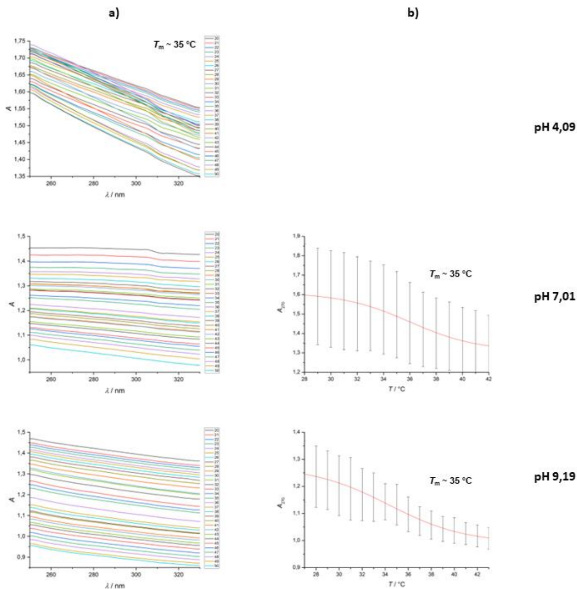
Slika 14. Temperaturno ovisni UV/Vis apsorpcijski spektri (a) SM liposoma suspendiranih u acetatnom (pH = 4,09), fosfatnom (pH = 7,01) i karbonatnom puferu (pH = 9,19) te temperaturna ovisnost apsorpcije SM liposoma suspendiranih u fosfatnom (pH = 7,01) i karbonatnom puferu (pH = 9,19) pri 270 nm (b). Posljednje nije prikazano za suspenziju u acetatnom puferu (pH = 4,09) zbog prevelike pogreške i nemogućnosti aproksimacije Boltzmannovom funkcijom
