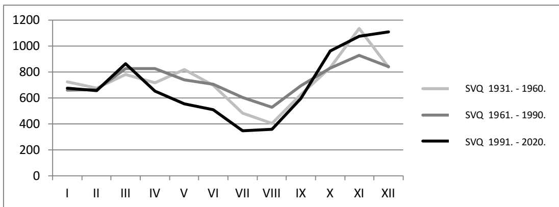
Sl. 19. Srednji mjesečni maksimumi na stanicama Zagreb i Rugvica za tri tridesetogodišnja razdoblja
