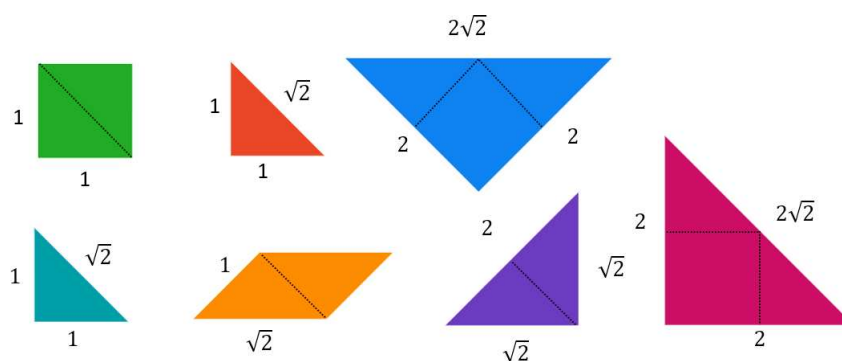
Slika 2.8: 16 jednakokranih pravokutnih trokuta
