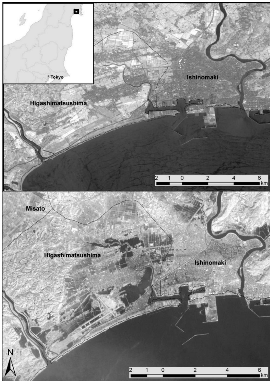
Sl. 15. Gradovi Ishinomaki i Higashimatsushima 2008. godine (gore) i 2011. godine (dolje) Izvor: Izradio autor prema podacima USGS (2022).
