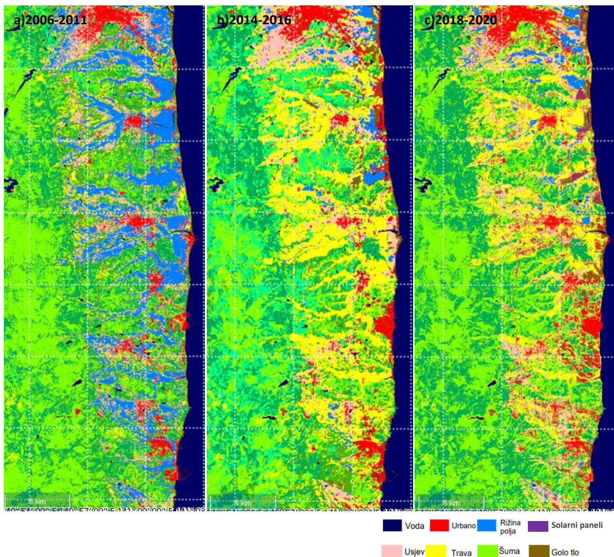
Sl. 22. LULC (Land Use Land Coverage) karta promjene zemljišnog pokrova južnog dijela prefekturu Miyagi i prefekturu Fukushima (a) 2006-2011, b) 2014-2016 i c) 2018-2020)
