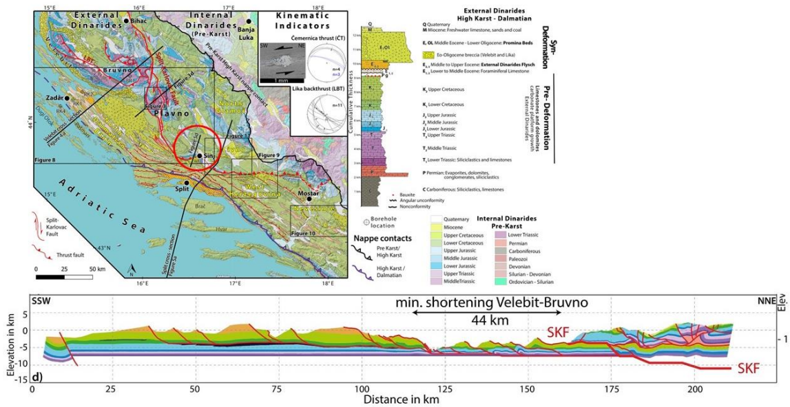
Slika 1.2.4 Detaljni profil SKF preuzet iz Balling et al. (2021) zajedno sa kartom (iznad) na kojoj je moguće vidjet kojim dijelom prolazi profil (označeno crvenim krugom)
