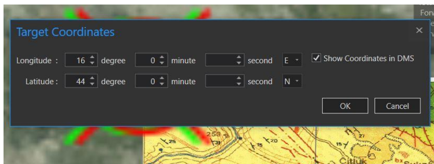
Slika 4.3 prikaz preuzet it ArcGIS Pro, naredba "Georeference -> Add Control Points" pomoću koje se upisuju zadane koordinate sa OGK Drniš
