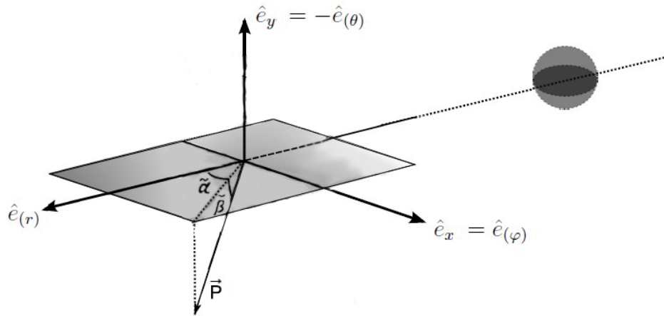
Slika 7.1: Prikaz kutova \tilde{\alpha} i \tilde{\beta} . Kutovi su nacrtani kao pozitivni. Kut \tilde{\beta} je kut između impulsa fotona i ravnine određene vektorima \hat{e}_r i \hat{e}_\phi . Kut \tilde{\alpha} je kut između projekcije impulsa fotona na ravninu određenu vektorima \hat{e}_r i \hat{e}_\phi i vektora \hat{e}_r . Vektori \hat{e}_x i \hat{e}_y određuju x-y ravninu u kojoj opažatelj vidi kritičnu krivulju crne rupe. Vidi Sliku 7.2. Preuzeto iz [47] i prilagođeno oznakama korištenim u ovom radu.
