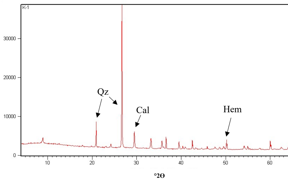
Slika 38. Rendgenogram veziva uzorka K-1. Oznake: Qz – kremen, Cal – kalcit, Hem – hematit.
