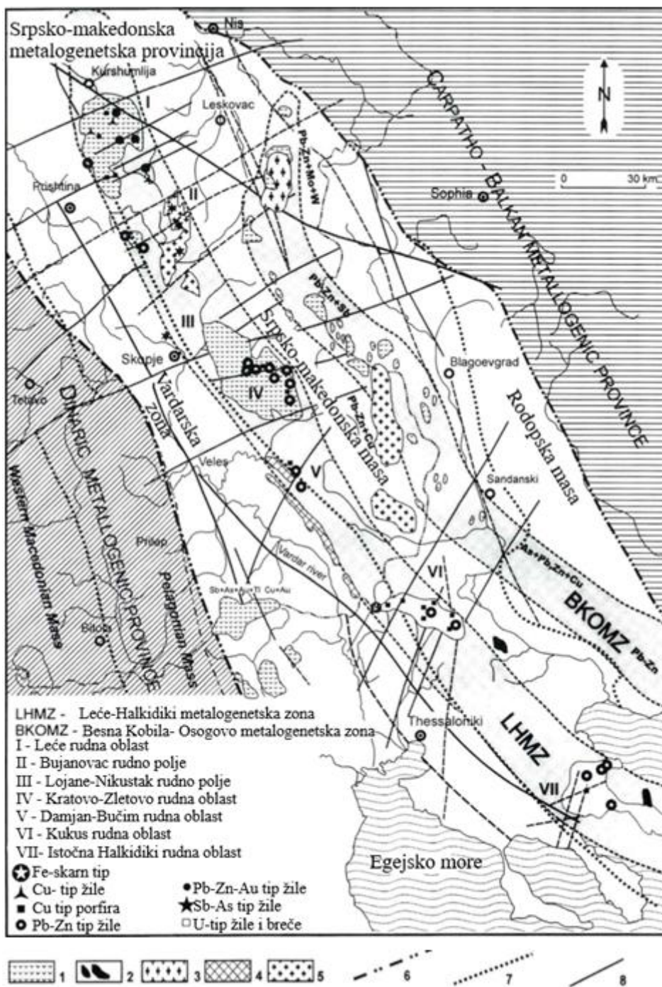
Slika 9. Geotektonski i metalogenetski smještaj Leče-Halkidiki zone: (1) neogenski vulkaniti; (2) terciarni intruzivi; (3) neogenski granitoidi; (4) jurski granodioriti; (5) hercinski graniti; (6) granice metalogenetskih provincija; (7) granice metalogenetskih zona; (8) lineamenti (prilagođeno prema: Serafimovski, 1999)
