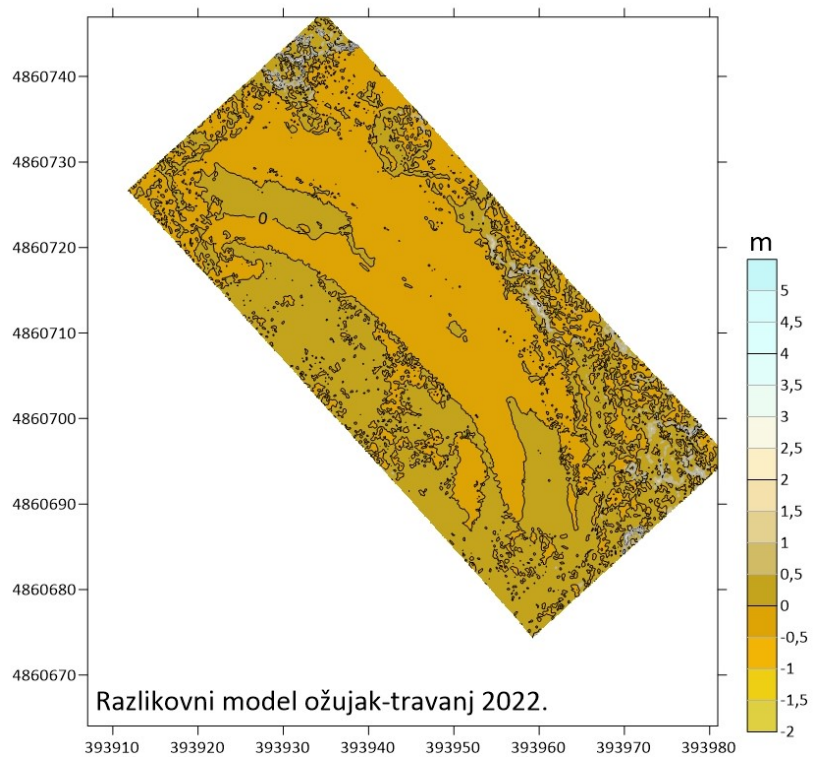
Slika 33 Razlikovni model plaže Lojšće za ožujak-travanj 2022.
