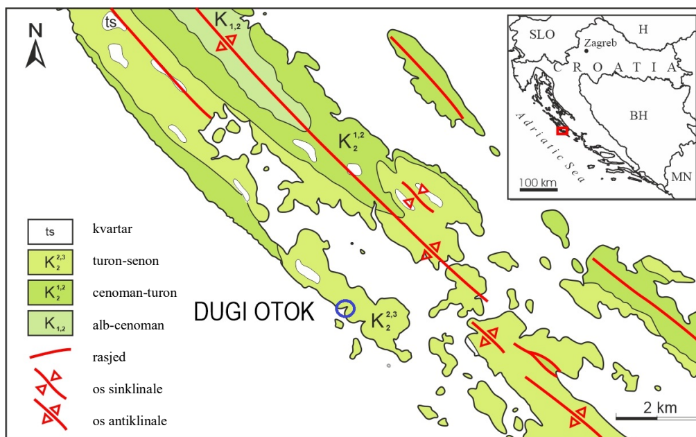
Slika 3 Geološka karta južnog dijela Dugog Otoka. Plaža Lojišće označena je plavim kružićem (prema MAMUŽIĆ i SOKAČ, 1967).
