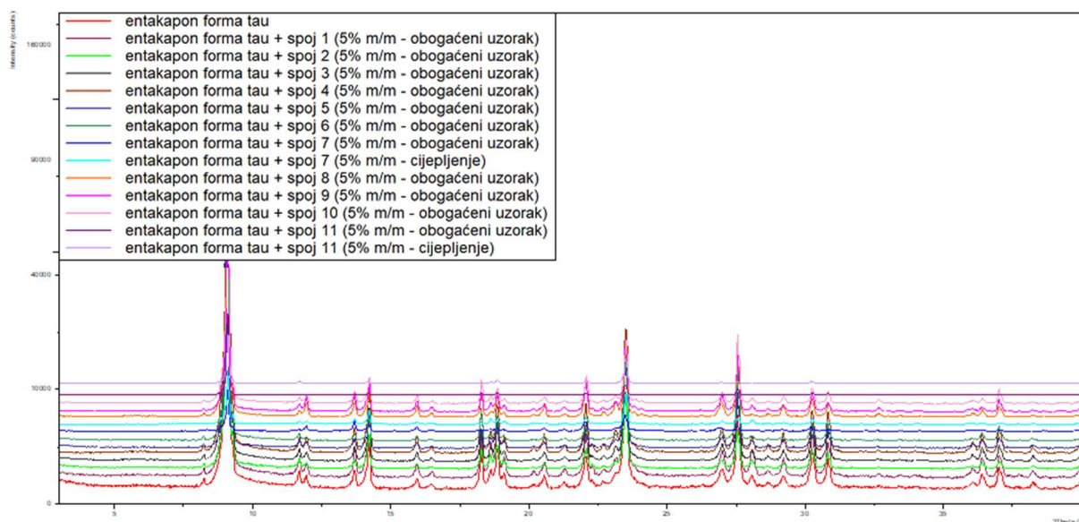
Slika D8. Usporedba difraktograma praha na polikristalnom uzorku izoliranih kristala iz pokusa utjecaja onečišćenja na ishod kristalizacije forme \tau .
