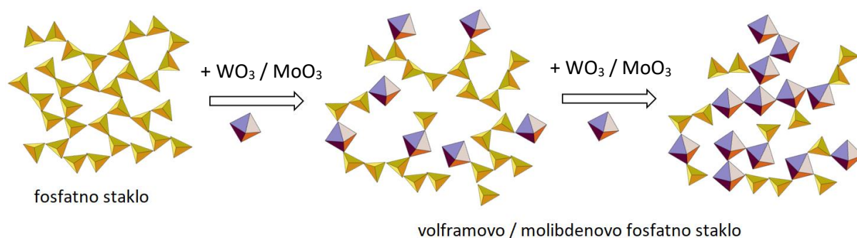
Slika 9. Shematski prikaz razvoja strukture fosfatnih stakala s dodatkom \text{WO}_3 i \text{MoO}_3 .
