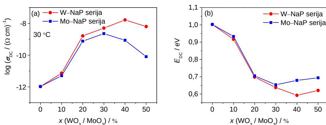
Slika 67. Ovisnost (a) DC provodnosti na 30 °C i (b) energije aktivacije za DC provodnost o množinskom udjelu \text{WO}_3 i \text{MoO}_3 u serijama stakala x\text{WO}_3\text{--}40\text{Na}_2\text{O--}(60\text{--}x)\text{P}_2\text{O}_5 i x\text{MoO}_3\text{--}40\text{Na}_2\text{O--}(60\text{--}x)\text{P}_2\text{O}_5 , x = 0\text{--}50 %.
