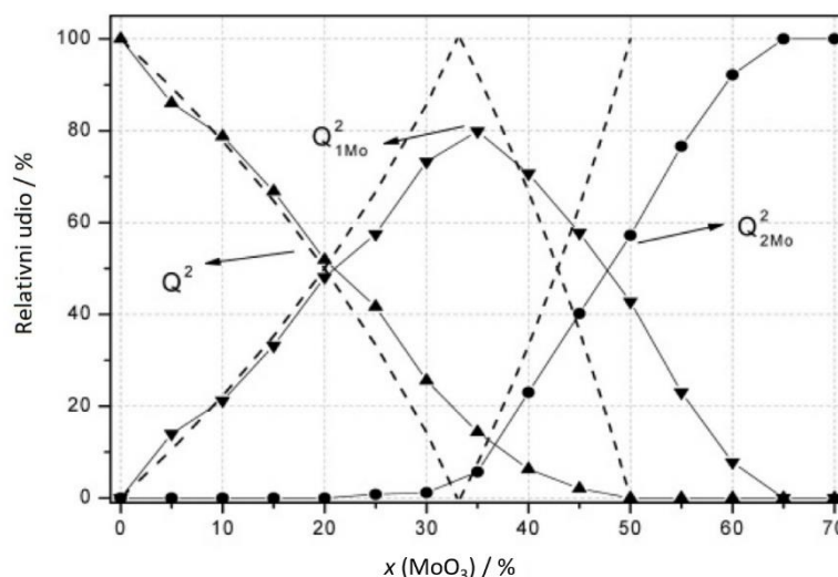
Slika 18. Relativni udjeli strukturnih jedinica dobiveni dekonvolucijom 31 P MAS-NMR spektara serije stakala (100-x)NaPO 3 -xMoO 3 (0 ≤ x ≤ 70 %). Isprekidane linije označavaju relativne udjele jedinica temeljene na teorijskom binarnom modelu. 29
