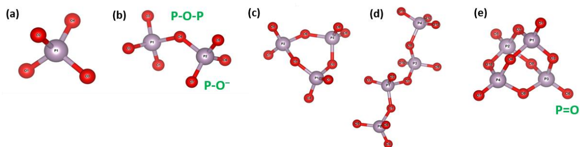
Slika 5. Optimizirane strukture različitih fosfatnih jedinica (a) ortofosfata [\text{PO}_4]^{3-} , (b) pirofosfata [\text{P}_2\text{O}_7]^{4-} , (c) cikličke [\text{P}_3\text{O}_9]^{3-} molekule, (d) polimernog lanca [\text{P}_4\text{O}_{13}]^{6-} te (e) ultrafosfatne \text{P}_3\text{O}_{10} molekule. 17
