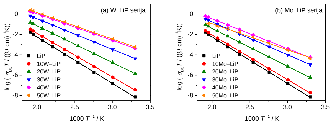
Slika 50. Arrheniusov graf ovisnosti DC provodnosti, \sigma_{DC} , o recipročnoj temperaturi za stakla iz serija (a) x\text{WO}_3\text{--}40\text{Li}_2\text{O--}(60\text{--}x)\text{P}_2\text{O}_5 i (b) x\text{MoO}_3\text{--}40\text{Li}_2\text{O--}(60\text{--}x)\text{P}_2\text{O}_5 , x = 0\text{--}50\% .
