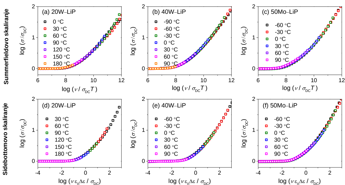
Slika 54. Spektri provodnosti 20W–LiP, 40W–LiP i 50Mo–LiP stakala iz serija x\text{WO}_3\text{--}40\text{Li}_2\text{O--}(60\text{--}x)\text{P}_2\text{O}_5 i x\text{MoO}_3\text{--}40\text{Li}_2\text{O--}(60\text{--}x)\text{P}_2\text{O}_5 , x = 0\text{--}50\% , skalirani primjenom (a-c) Summerfieldovog i (d-f) Sidebottomovog postupka.
