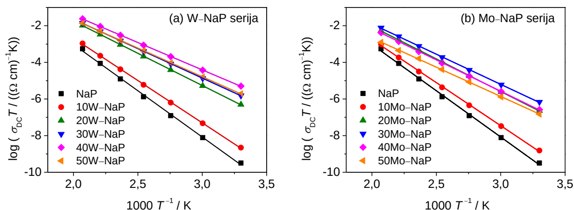
Slika 66. Arrheniusov graf ovisnosti DC provodnosti, \sigma_{DC} , o recipročnoj temperaturi za stakla iz serija (a) x\text{WO}_3\text{--}40\text{Na}_2\text{O--}(60-x)\text{P}_2\text{O}_5 i (b) x\text{MoO}_3\text{--}40\text{Na}_2\text{O--}(60-x)\text{P}_2\text{O}_5 , x = 0\text{--}50 %.
