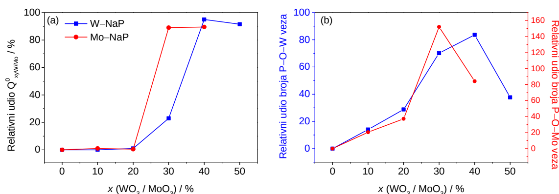
Slika 64. Ovisnost relativnog udjela (a) Q^0_{xyW/Mo} jedinica i (b) relativnog udjela broja P–O–W/Mo veza o udjelu WO_3 i MoO_3 za serije stakala xWO_3-40Na_2O-(60-x)P_2O_5 i xMoO_3-40Na_2O-(60-x)P_2O_5 , x = 0-50\% .
