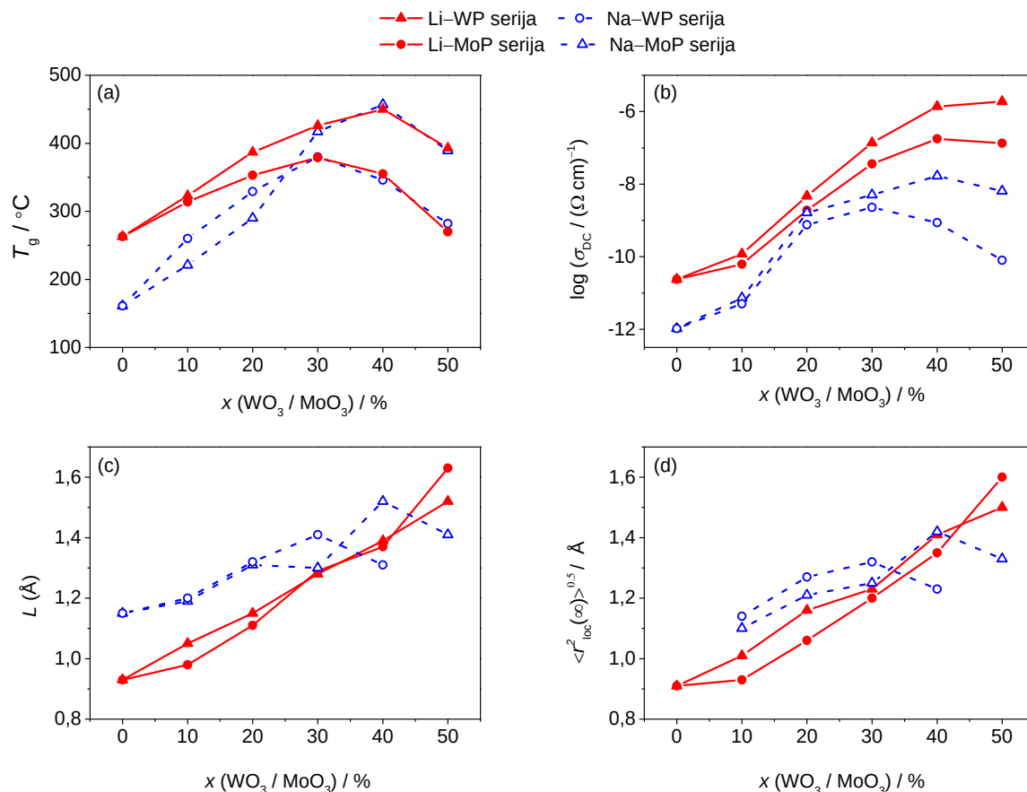
Slika 76. Usporedbe trendova ovisnosti (a) temperature staklišta, T_g , (b) DC provodnosti na 30 °C, \sigma_{DC} , (c) Sidebottomove duljine, L , i (d) dosega lokaliziranog preskoka iona, \langle r_{loc}^2(\infty) \rangle^{0,5} , o udjelu WO 3 i MoO 3 za litijeve i natrijeve serije stakala.
