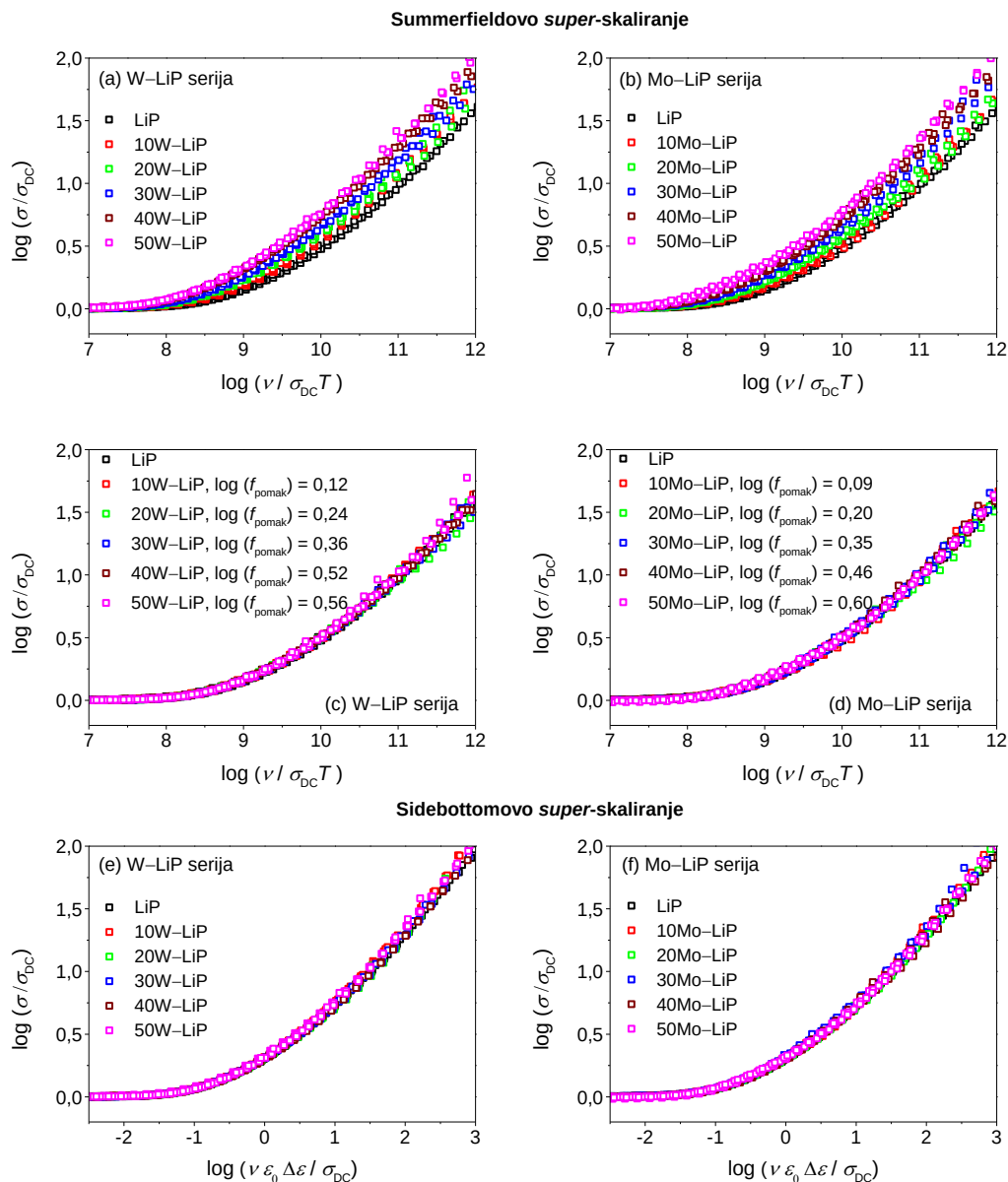
Slika 55. Konstrukcija super-master krivulja za stakla iz serija x\text{WO}_3\text{--}40\text{Li}_2\text{O--}(60\text{--}x)\text{P}_2\text{O}_5 i x\text{MoO}_3\text{--}40\text{Li}_2\text{O--}(60\text{--}x)\text{P}_2\text{O}_5 , x = 0\text{--}50\% , primjenom (a-d) Summerfieldovog i (e-f) Sidebottomovog postupka. Iznos faktora pomaka, \log(f_{\text{pomak}}) , pojedine krivulje označen je u legendi.
