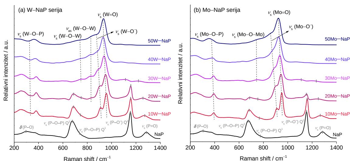
Slika 60. Ramanovi spektri serija stakala (a) x\text{WO}_3\text{--}40\text{Na}_2\text{O--}(60\text{--}x)\text{P}_2\text{O}_5 i (b) x\text{MoO}_3\text{--}40\text{Na}_2\text{O--}(60\text{--}x)\text{P}_2\text{O}_5 , x = 0\text{--}50 %.
