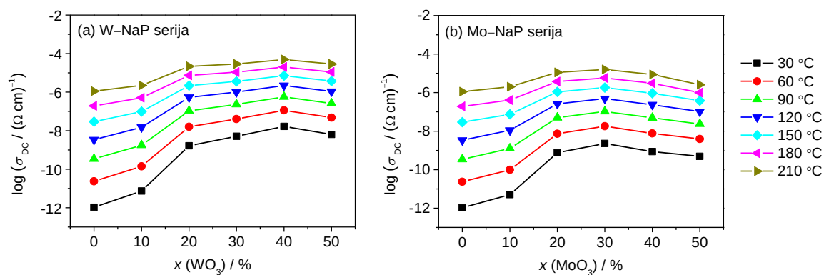
Slika D6. Ovisnost DC provodnosti na različitim temperaturama o udjelu \text{WO}_3 odnosno \text{MoO}_3 za stakla iz serija (a) x\text{WO}_3\text{--}40\text{Na}_2\text{O--}(60\text{--}x)\text{P}_2\text{O}_5 i (b) x\text{MoO}_3\text{--}40\text{Na}_2\text{O--}(60\text{--}x)\text{P}_2\text{O}_5 , x = 0\text{--}50\% .
