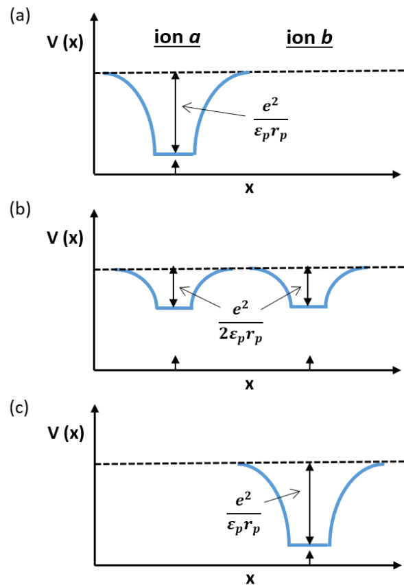
Slika 12. Shematski prikaz procesa gibanja polarona i potencijalnih jama (a) prije preskoka elektrona, (b) u trenutku termički aktiviranog stanja jednakih energija kada elektron može preskočiti i (c) nakon preskoka elektrona.
