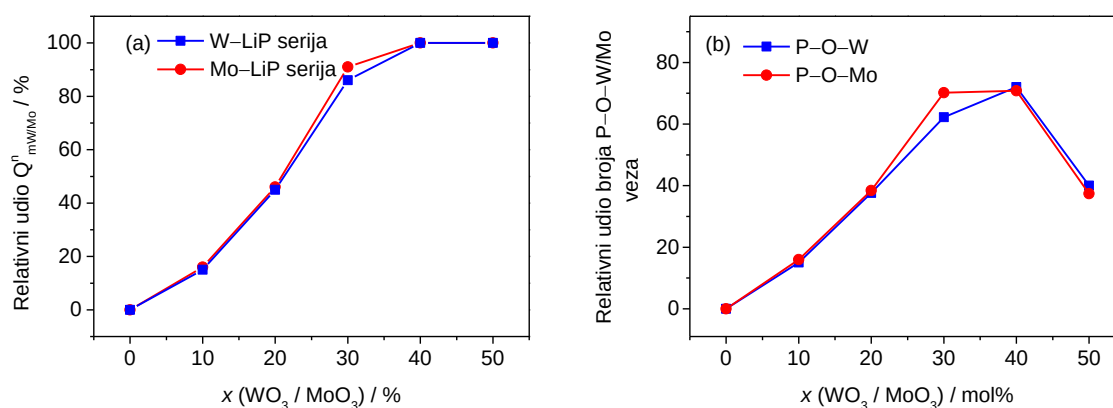
Slika 48. Ovisnost (a) ukupnog relativnog udjela „miješanih“ Q_{\text{mW/Mo}}^n jedinica i (b) relativnog udjela broja P–O–W te P–O–Mo veza za serije stakala x\text{WO}_3\text{--}40\text{Li}_2\text{O--}(60-x)\text{P}_2\text{O}_5 i x\text{MoO}_3\text{--}40\text{Li}_2\text{O--}(60-x)\text{P}_2\text{O}_5 , x = 0\text{--}50\% .
