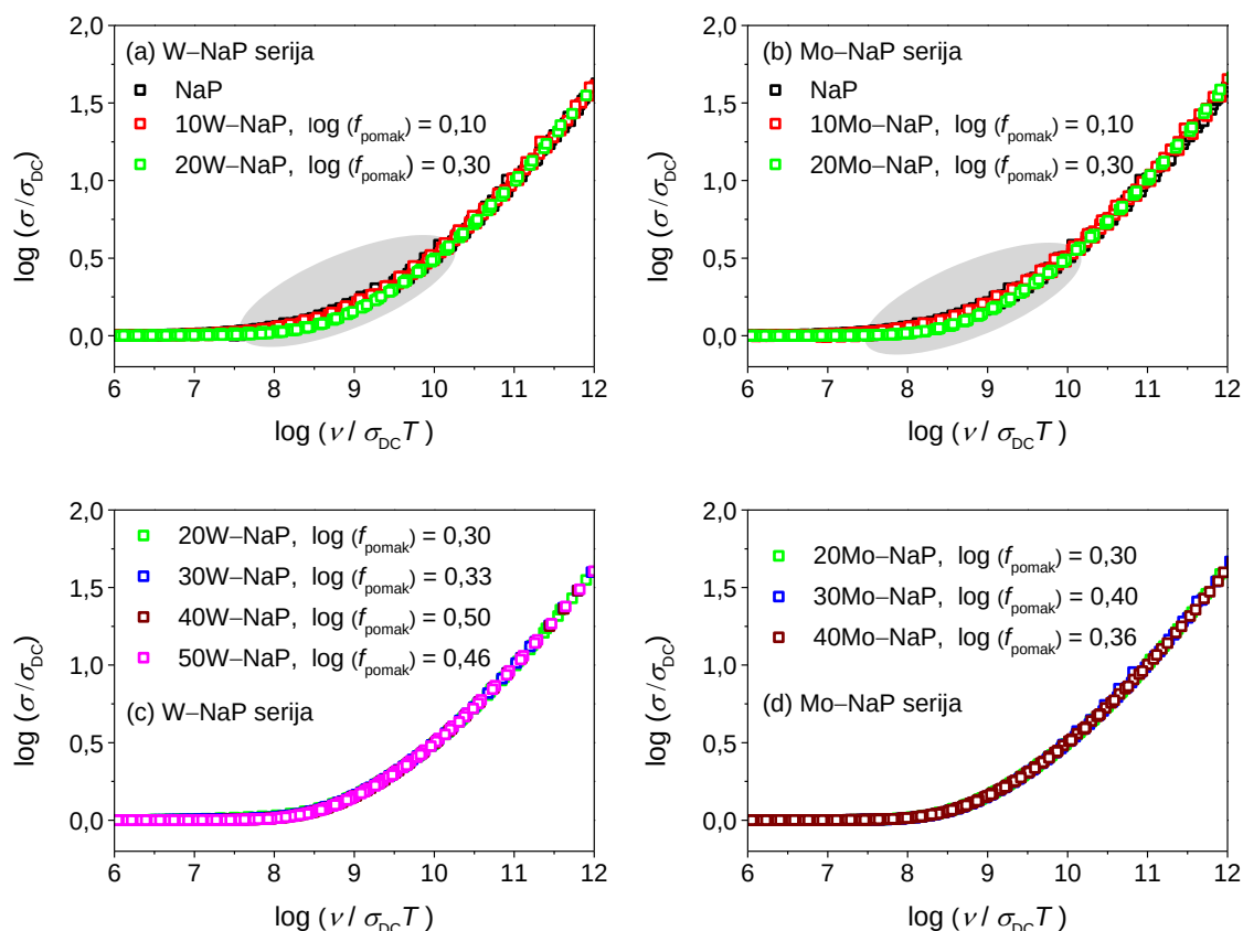
Slika 72. Master krivulje provodnosti pomaknute duž osi x primjenom odgovarajućeg faktora pomaka, \log(f_{\text{pomak}}) , za stakla s (a) x(\text{WO}_3) = 0\text{--}20\% , (b) x(\text{MoO}_3) = 0\text{--}20\% , (c) x(\text{WO}_3) = 20\text{--}50\% , i (d) x(\text{MoO}_3) = 20\text{--}40\% . Iznos faktora pomaka pojedine krivulje označen je u legendi.
