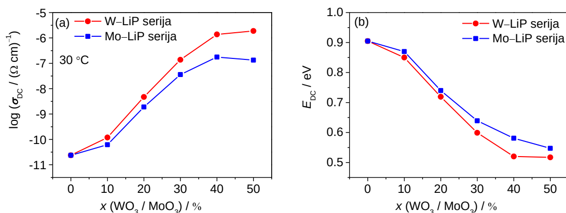
Slika 51. Ovisnost (a) DC provodnosti na 30^\circ \text{C} i (b) energije aktivacije za DC provodnost o množinskom udjelu \text{WO}_3 i \text{MoO}_3 u serijama stakala x\text{WO}_3-40\text{Li}_2\text{O}-(60-x)\text{P}_2\text{O}_5 i x\text{MoO}_3-40\text{Li}_2\text{O}-(60-x)\text{P}_2\text{O}_5 , x = 0-50\% .
