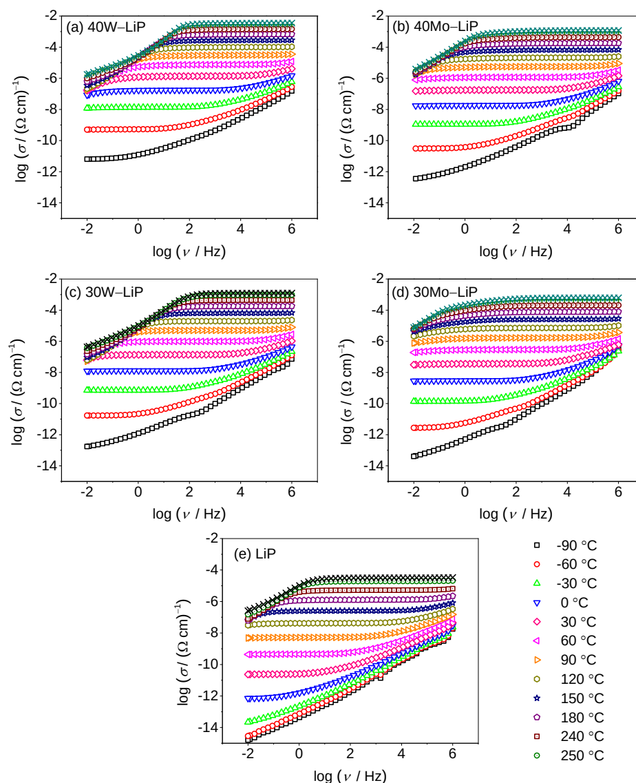
Slika 49. Spektri električne provodnosti pri različitim temperaturama za odabrana stakla iz serija x\text{WO}_3\text{--}40\text{Li}_2\text{O--}(60-x)\text{P}_2\text{O}_5 i x\text{MoO}_3\text{--}40\text{Li}_2\text{O--}(60-x)\text{P}_2\text{O}_5 , x = 0\text{--}50\% .
