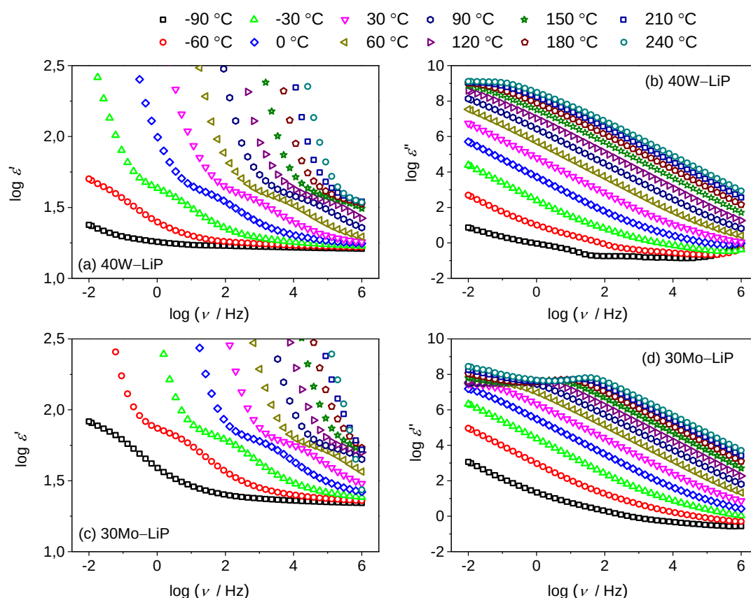
Slika 53. Frekvencijska ovisnost (a i c) realnog, \epsilon' , i (b i d) imaginarnog, \epsilon'' , dijela permitivnosti pri različitim temperaturama za 40W-LiP staklo i 30Mo-LiP staklo.
