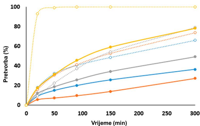
Slika 40. Pretvorba ciklooktena u odnosu na vrijeme s Mo(VI) kompleksima. Kompleksi: [\text{MoO}_2(\text{SalNH})_n (plava linija), [\text{MoO}_2(3\text{OMeSalNH})_n (narančasta linija), [\text{MoO}_2(4\text{OMeSalNH})_n (siva linija) i [\text{MoO}_2(4\text{OMeSalNH})_4 \cdot 0,5\text{MeCN}] (žuta linija). Puna linija označava reakciju s vodenom otopinom TBHP, dok isprekidana linija označava reakciju uz upotrebu TBHP u dekanu.
