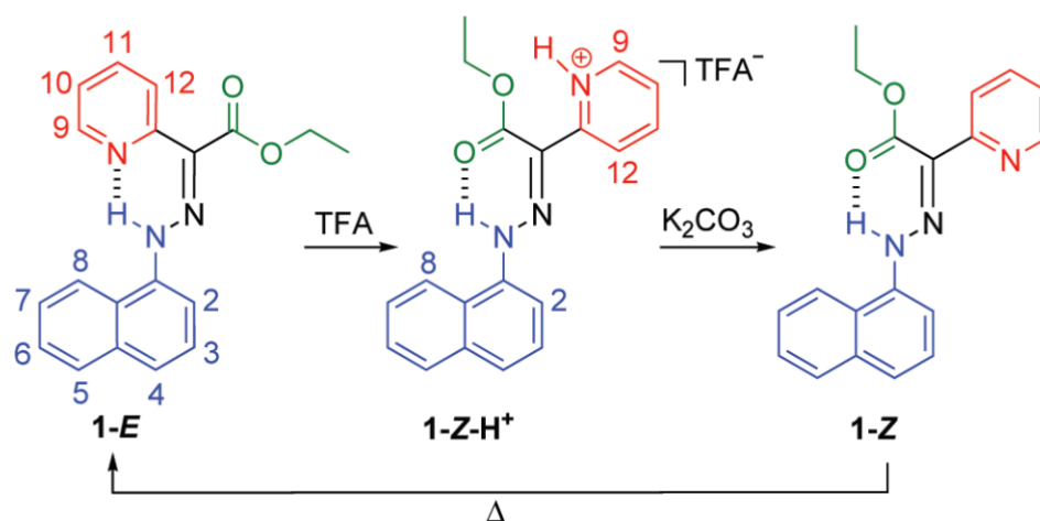
Slika 8. Prikaz izomerije hidrazona kontrolirane trifluorooctenom kiselinom (TFA) i kalijevim karbonatom. 34
