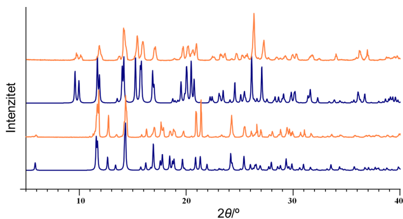
Slika D11. Usporedba izračunatog (plavo) difraktograma praša i eksperimentalno dobivenih (narančasto) ( [\text{MoO}_2(3\text{OMeSIH})(\text{MeOH})] ( \alpha i \beta ): polimorf \alpha dobiven reakcijom [\text{MoO}_2(\text{acac})_2] i \text{H}_23\text{OMeSIH} u metanolu (gore) i polimorf \beta dobiven deprotonacijom [\text{MoO}_2(\text{H3OMeSIH})\text{Cl}]\cdot \text{MeOH} (dole).
