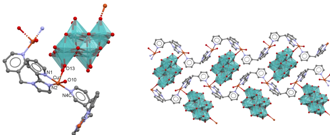
Slika 32. Koordinacija oko Cu(II) iona u spoju [\text{CuL}(\text{H}_2\text{O})(\beta\text{-Mo}_8\text{O}_{26})_{0.5}] \cdot 2\text{H}_2\text{O} i 2D mreža koju čine metalo-organski polimer i oktamolibdatni anioni.
