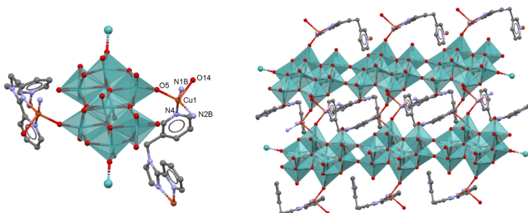
Slika 33. Koordinacija oko Cu(II) iona u spoju [\text{CuL}(\text{H}_2\text{O})(\gamma\text{-Mo}_8\text{O}_{26})_{0.5}] \cdot 2\text{H}_2\text{O} i mreža koju čine metalo-organski polimer i oktamolibdatni anioni.
