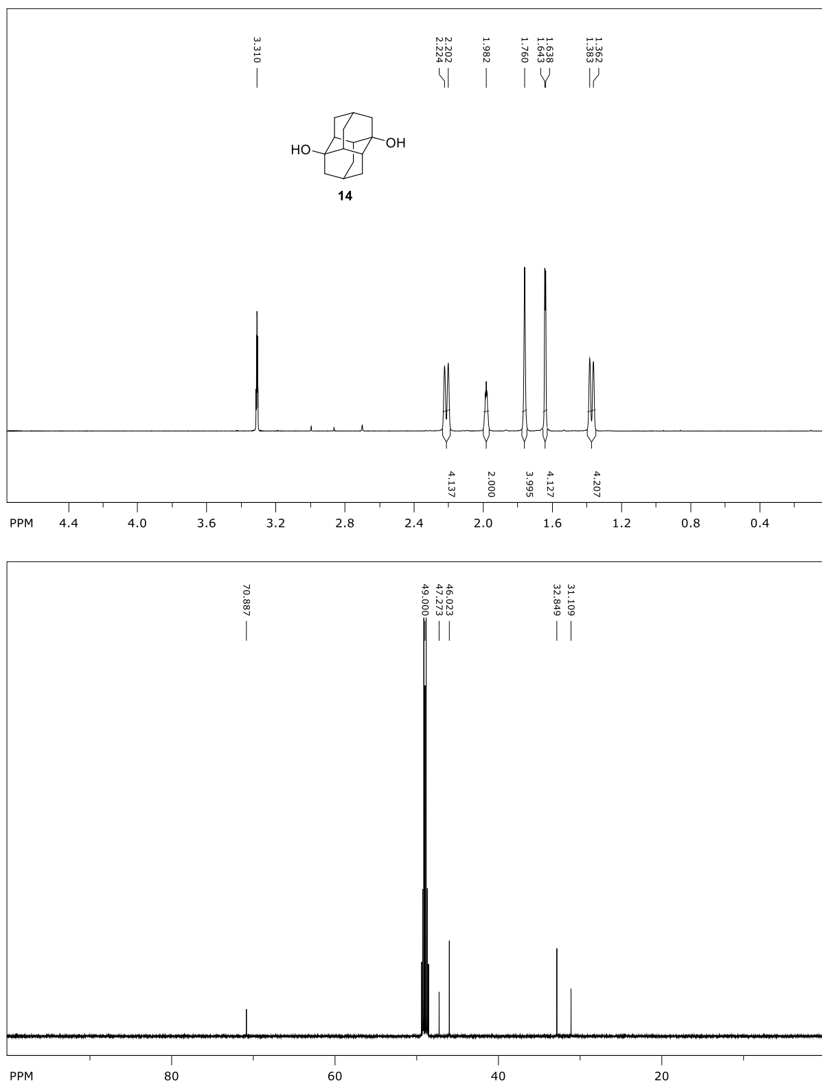
Prilog 10. ^1\text{H} ( \text{CDCl}_3 , 600 MHz) i ^{13}\text{C} ( \text{CDCl}_3 , 150 MHz) NMR spektri spoja 14 .
