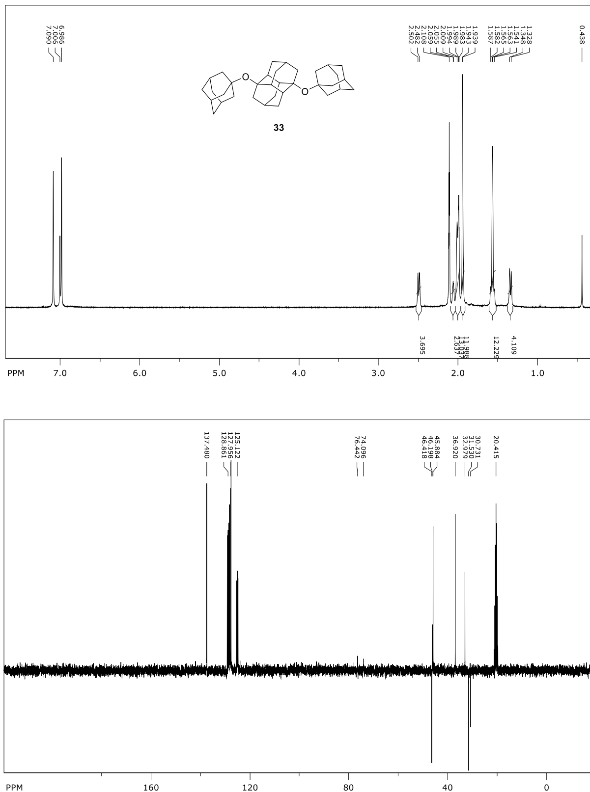
Prilog 27. 1 H (600 MHz, toluene- d 8 , 70 °C) i 13 C NMR (75 MHz, toluene- d 8 , 70 °C) spektri spoja 33 .
