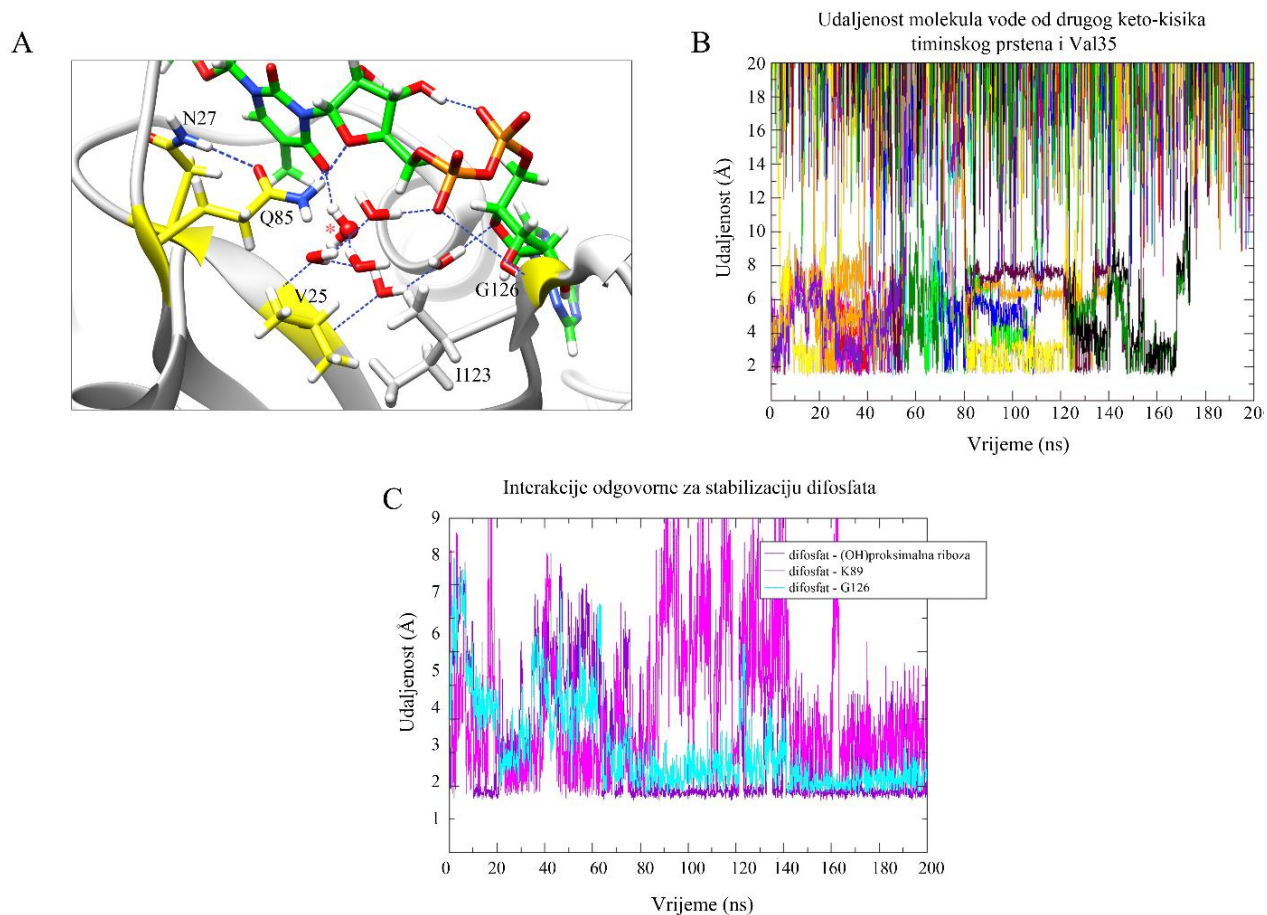
Slika 23. Interakcije odgovorne za pravilno pozicioniranje razvijene mreže molekula vode unutar aktivnog mjesta proteina SCO6735 u kompleksu s pripadnim supstratom (dT-ADPr). Mreža molekula vode pravilno pozicioniranih unutar aktivnog mjesta između Gln85 i difosfata pripadnog supstrata (A). Molekula vode koja je ugniježđena između drugog keto-kisikovog atoma u timinskom prstenu supstrata te okosnice Val35 i koja bi mogla započeti enzimsku katalizu je označena crvenom zvjezdicom. Grafički prikaz udaljenosti molekula vode koje se tijekom 200 ns simulacije izmjenjuju i ugnježđuju između drugog keto-kisikovog atoma timina i okosnice Val35 (B). Grafički prikaz udaljenosti između atoma difosfata i proksimalne riboze, Lys89, i Gly126 s kojima ostvaruje stabilnu vodikovu vezu tijekom 200 ns simulacije (C).
