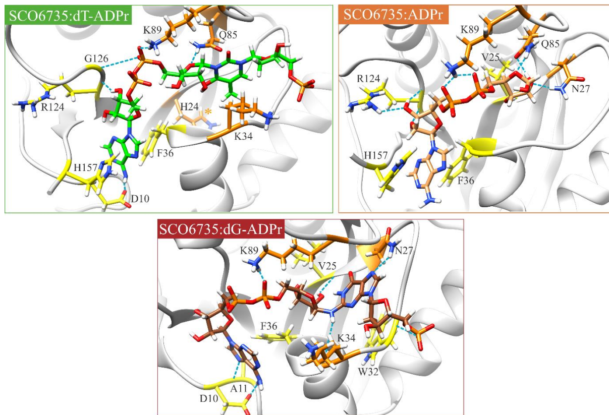
Slika 21. Glavne interakcije koje protein SCO6735 ostvaruje s ADPr te pripadnim (dT-ADPr) i neprirodnim (dG-ADPr) supstratom tijekom 200 ns simulacija. Interakcije koje se ostvaruju u kompleksu s dT-ADPr prikazane su u zelenom, s ADPr u narančastom i dG-ADPr u crvenom kvadratu. Označene interakcije detektirane su u više od 20 % simulacijskog vremena. Aminokiseline čiji su doprinos katalizi i vezanju liganda istraženi mjesno-specifičnom
