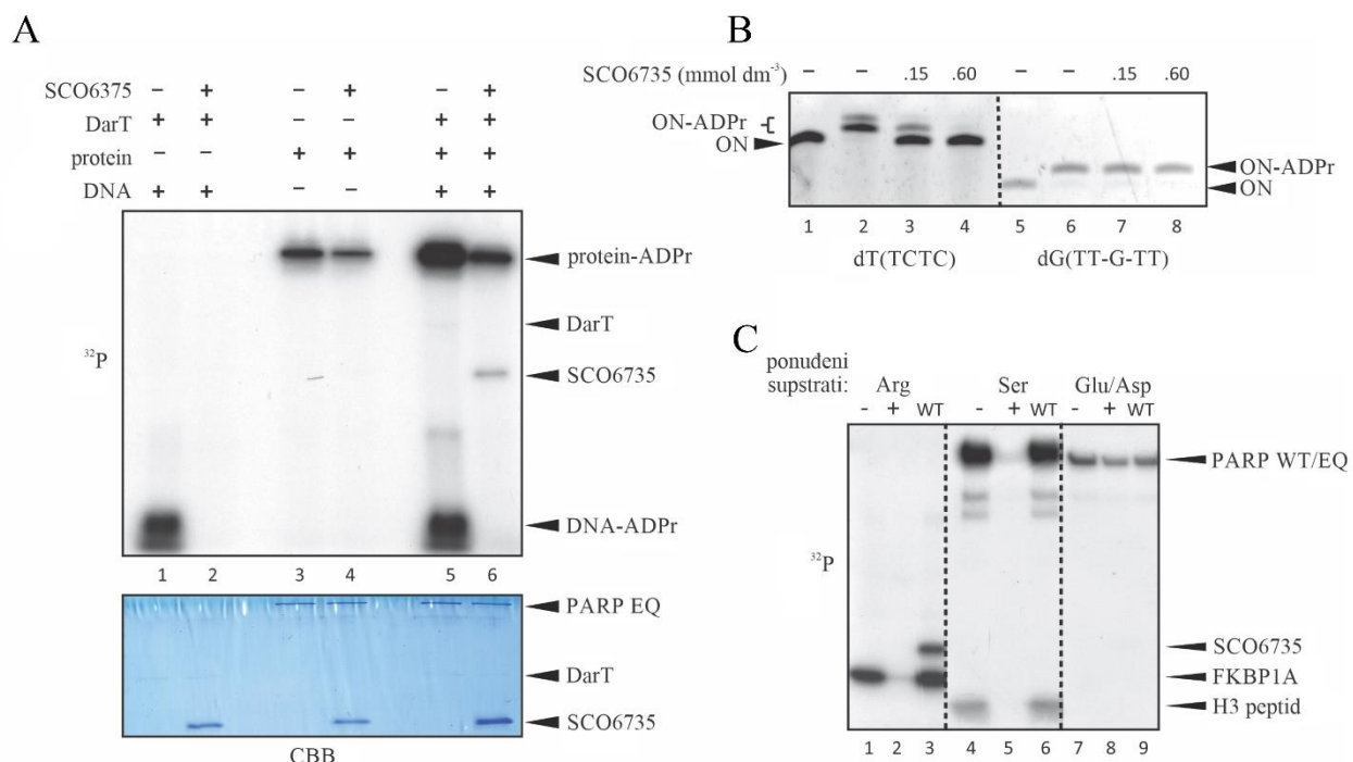
Slika 15. Testiranje aktivnosti proteina SCO6735 na različitim proteinskim i DNA supstratima. Rezultati kompetencijskog eksperimenta u kojem je testirana preferencije prema proteinskom ili DNA supstratu (A). U eksperimentu su korišteni radioaktivno obilježeni supstrati, a produkti reakcije su razdvojeni na SDS-PAGE gelu i potom detektirani autoradiografski. Na donjoj slici prikazan je isti gel, pri čemu su proteinski uzorci obojani CBB bojom u svrhu kontrole količine proteina i pravilnog nanošenja uzorka. Testiranje djelovanja proteina SCO6735 na modificiranim timinima i gvaninima (B). Produkti reakcijske smjese su razdvojeni na poliakrilamidnom urea gelu i vizualizirani pomoću SYBR™ Gold boje. Testiranje aktivnosti SCO6735 na proteinima kojima su ADP-ribozilirani bočni ogranci Ser ili Arg (C). Produkti reakcije su razdvojeni na SDS-PAGE gelu, te vizualizirani autoradiografski.
