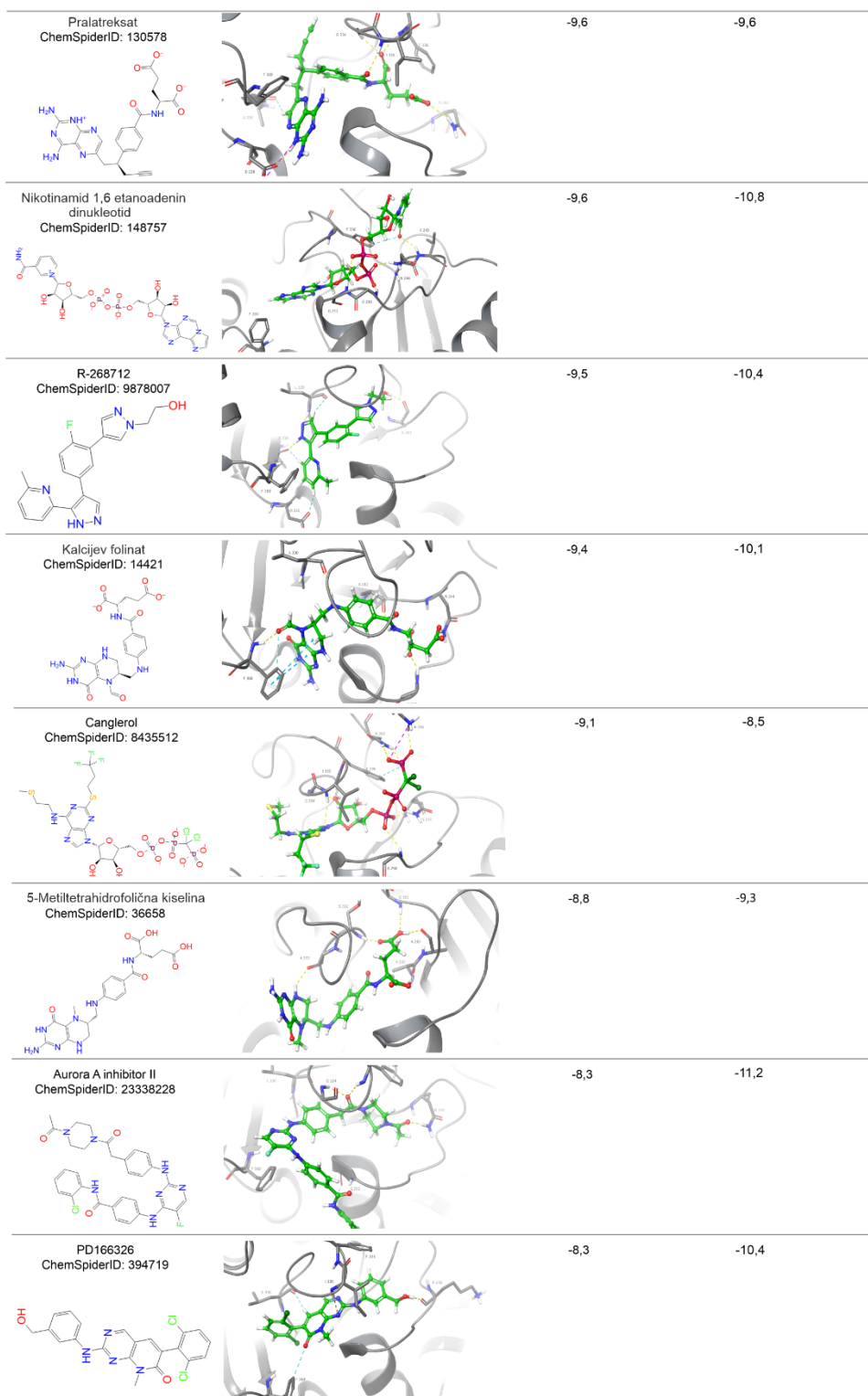
Slika D4. Predviđeni načini vezanja spojeva koji nisu pokazali dobar afinitet vezanja tijekom ITC mjerenja u zadanim uvjetima. Prikazani su načini vezanja dobiveni programom Glide opcijom Standard Precision . Desno su prikazani bodovi molekuskog vrednovanja dobiveni
