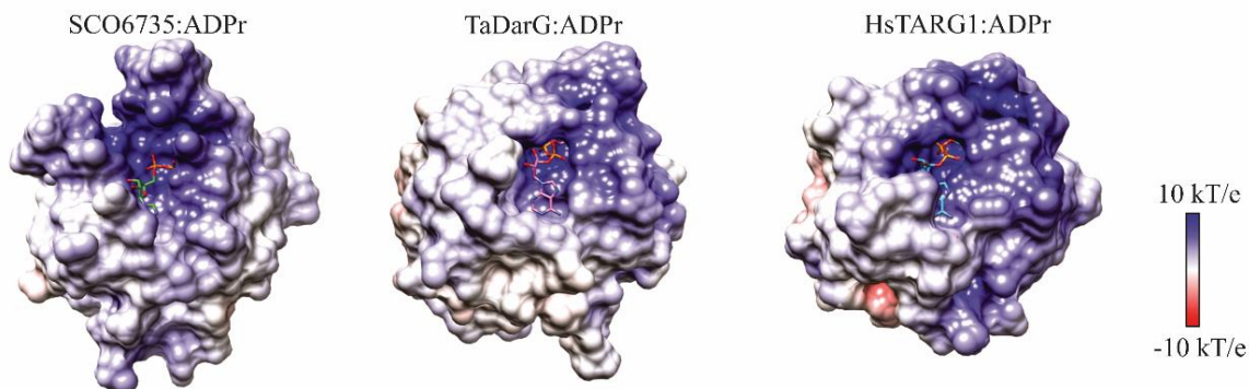
Slika 19. Usporedba elektrostatske površine proteina SCO6735, HsTARG1 (PDB: 4J5S) i TaDarG (PDB: 5M3E) u kompleksu s ADPr izračunate mrežno dostupnim programom APBS 85 . Sukladno prikazanoj legendi, tamno plavom bojom su naznačeni najelektropozitivniji, a crvenom najelektronegativniji dijelovi strukture.
