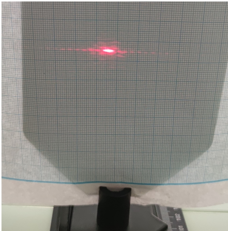
Slika 6.23: Ogibna slika na pukotini širine d = 0,2\text{mm}
