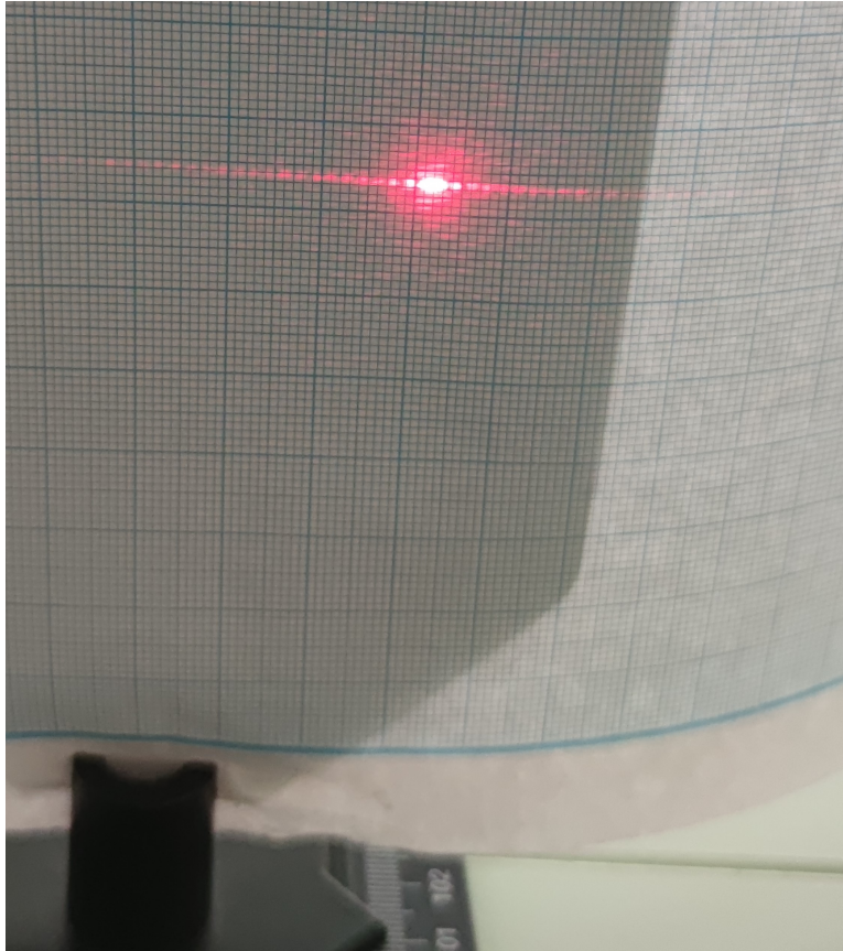
Slika 6.22: Ogibna slika na pukotini širine d = 0,4\text{mm}
