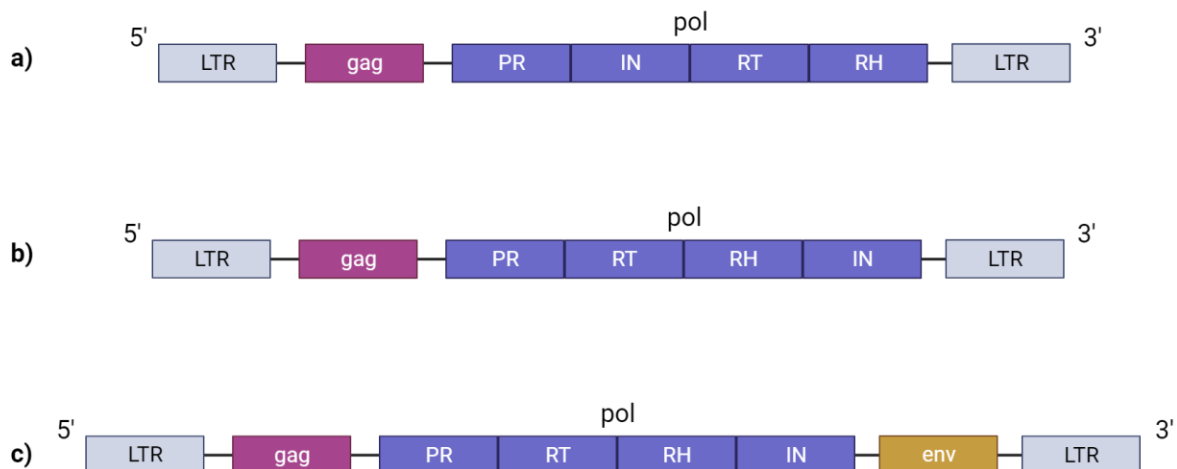
Slika 1. Struktura LTR retroelementa. a) Ty1/Copia skupina s redoslijedom domena u genu pol PR-IN-RT-RH; b) Ty3/Gypsy i Bel/Pao skupine s redoslijedom PR-RT-RH-IN; c) retrovirusi te pripadnici skupina Ty1/Copia, Ty3/Gypsy i Bel/Pao koji su neovisno stekli gen env , s redoslijedom PR-RT-RH-IN. Shematski prikaz prilagođen prema Llorens i sur. (2011), Wang i Han (2022), Warren i sur. (2015).
