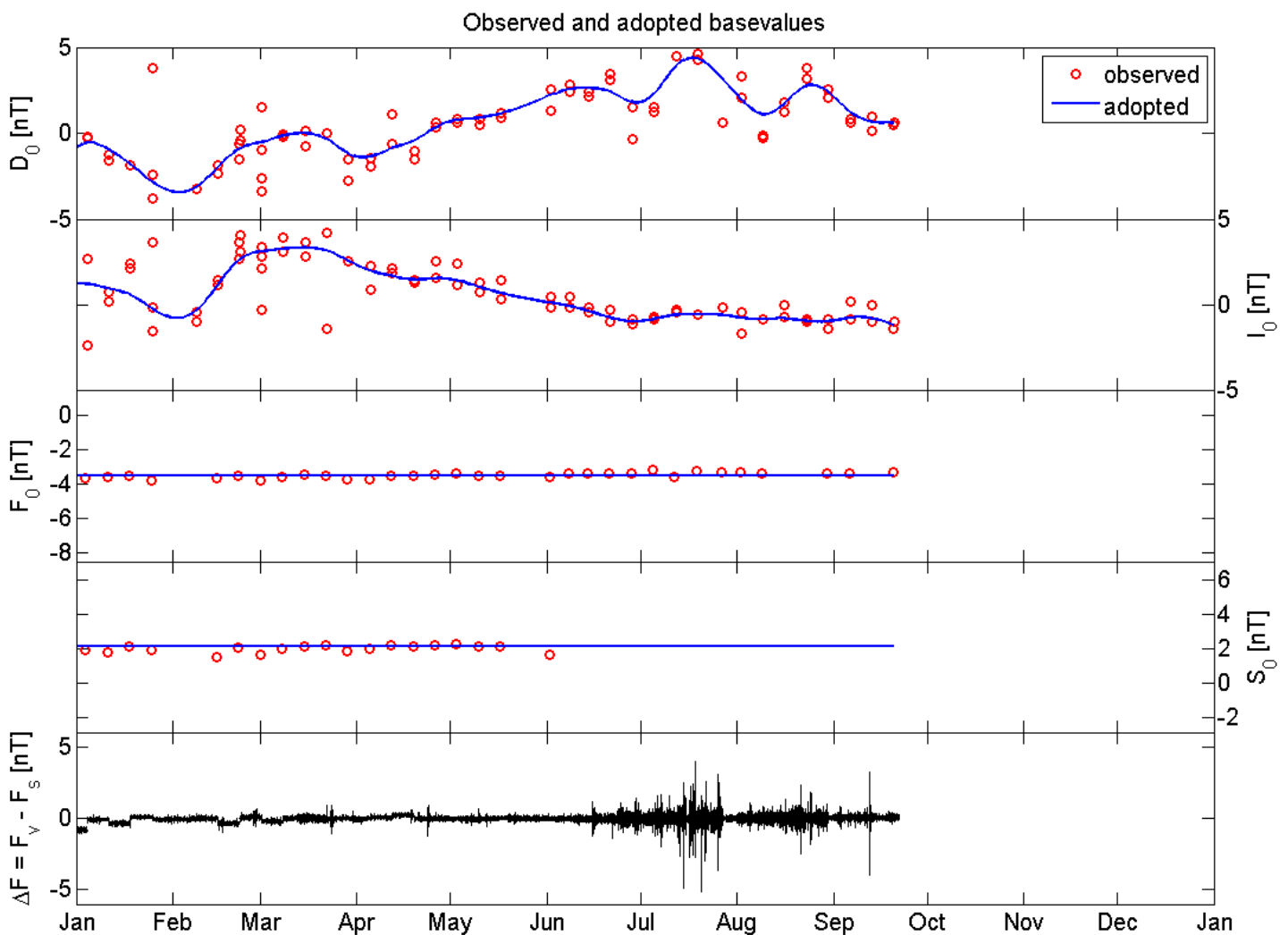
Slika 2.2 – Opažene ( engl. observed ) i prilagođene ( engl. adopted ) kalibracijske vrijednosti za DIDD variometar. Na slici su također prikazani rezultati motrenja s početka rujna koji su korišteni u izračunu kalibracijskih krivulja za kolovoz.
