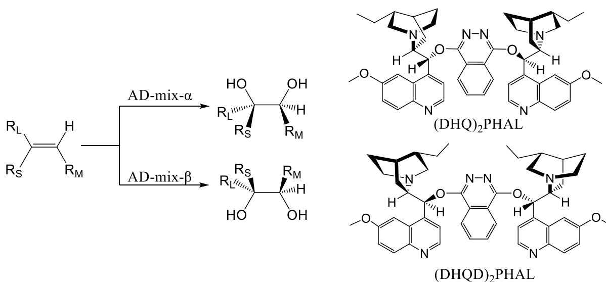
Slika 10. Sharplessova asimetrična dihidroksilacija alkena. Desno su dane strukture ftalizinskih adukata kiralnih kininskih liganada (\text{DHQD})_2\text{PHAL} i (\text{DHQD})_2\text{PHAL} sadržanih u komercijalnim smjesama reagensa za ovu reakciju AD-mix- \alpha , odnosno AD-mix- \beta . Kratice S, M i L označavaju veličinu supstituenata, a dolaze od engleskih riječi small , medium i large .
