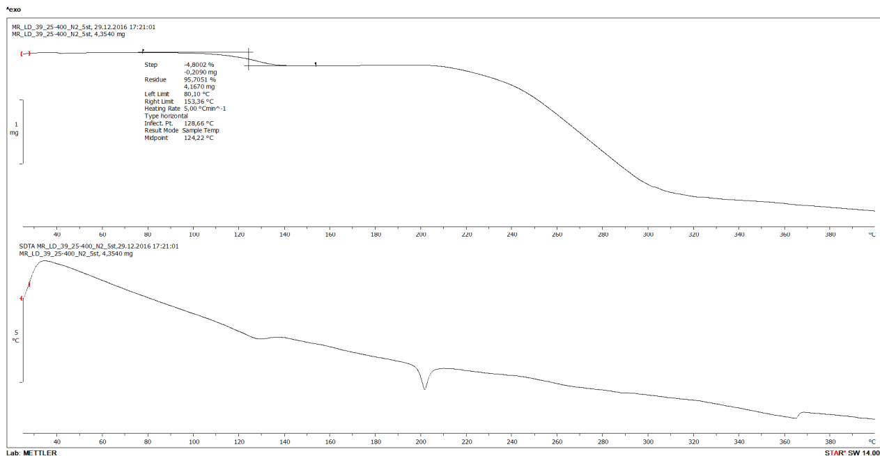
Slika XXX. TG krivulja (gore) i SDTA krivulja (dolje) spoja \text{H}_3\text{L}^{\text{py-sal}} \cdot \text{H}_2\text{O} . Analiza je provedena u struji dušika u temperaturnom području od 25 °C - 600 °C.
