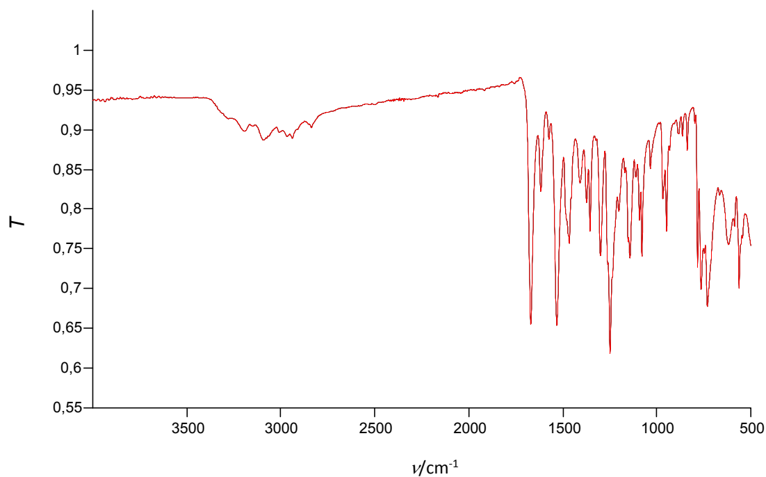
Slika XVI. IR spektar spoja H_4L^{sal-ovan} pripremljenog klasičnom otopinskom sintezom opisanom u poglavlju 3.2.4. Postupak III .
