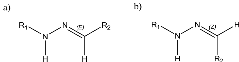
Slika 2. Dijastereoizomeri hidrazona
