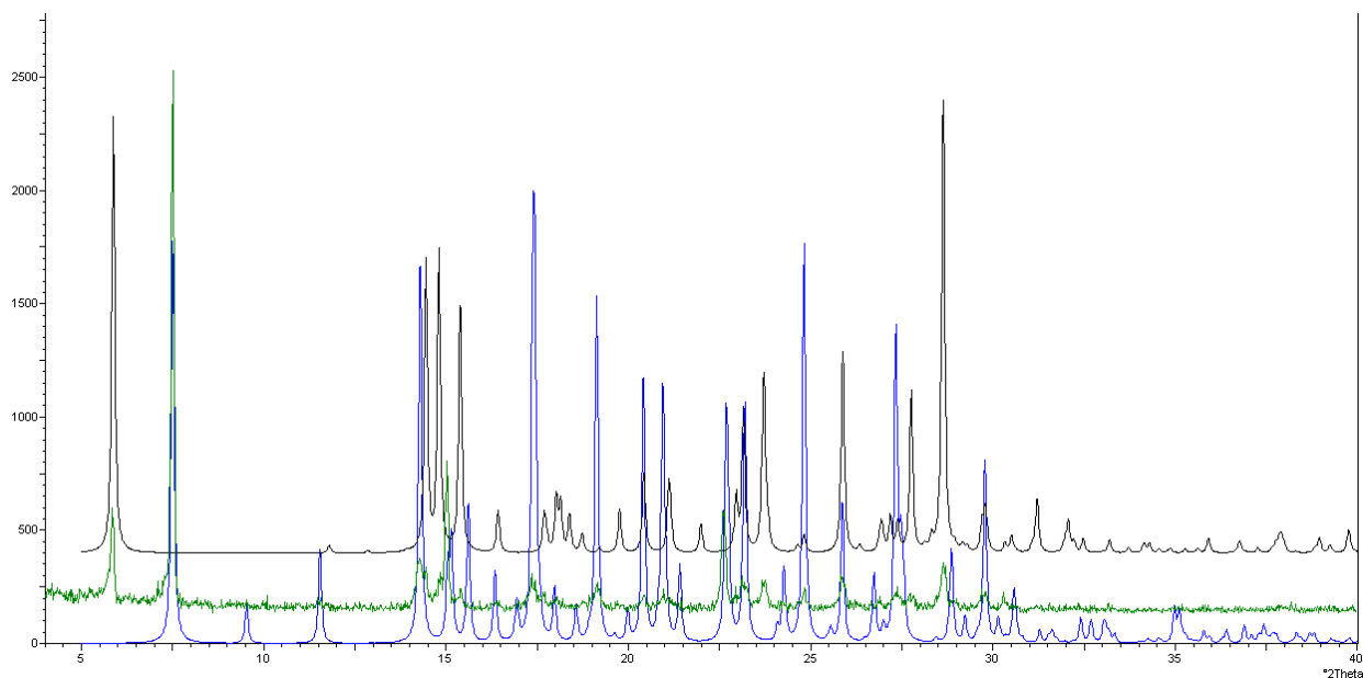
Slika XXXIII. Usporedba difraktograma praškastog uzorka produkta dobivenog iz matičnice u sintezi opisanoj u poglavlju 3.2.6. Postupak II. (zeleno) sa simuliranim difraktogramom praha spoja H_3L^{py-sal} (plavo) i spoja H_3L^{py-sal} \cdot H_2O (crno)
