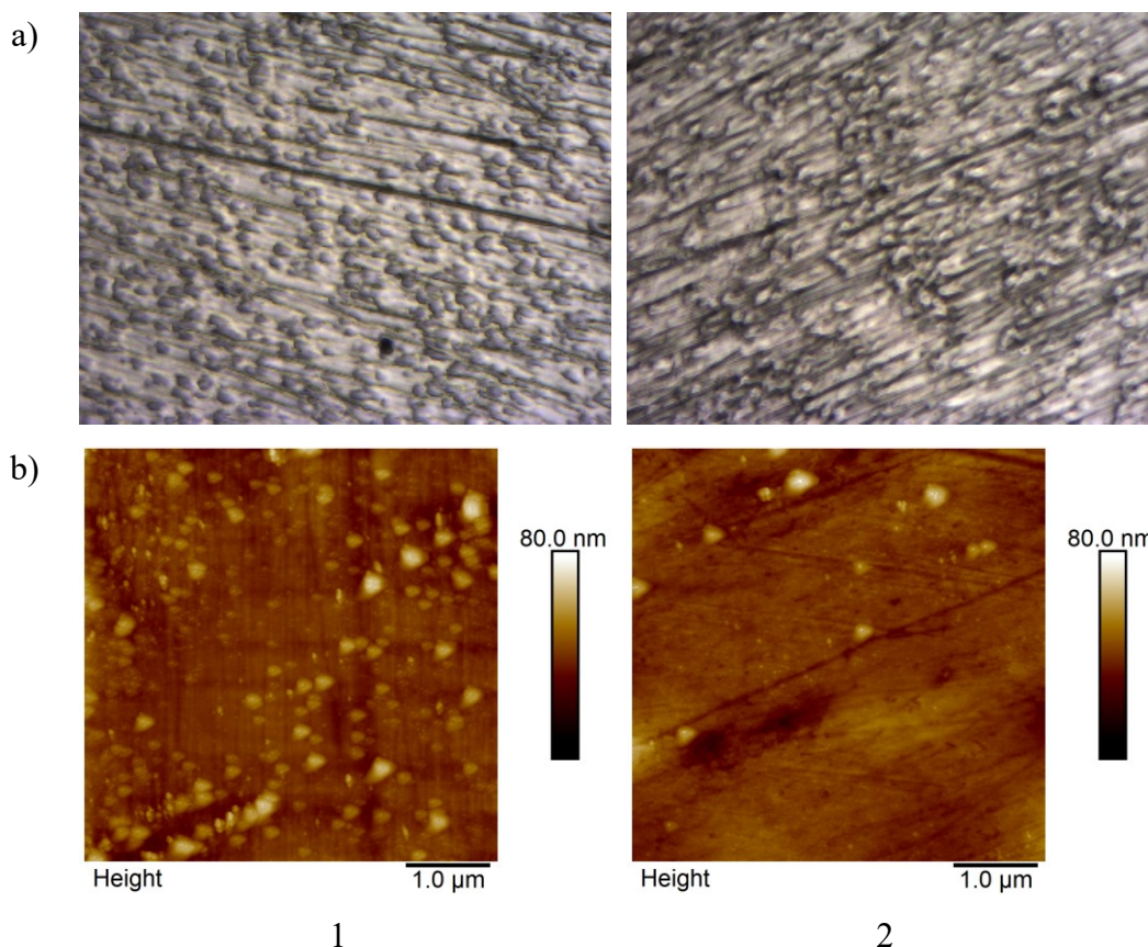
Slika 4.18. Površina pločica titanijsa sa slojem titanijsva dioksida nakon adsorpcije polikationa P4VP-a dobivene a) optičkim mikroskopom ( 500 \times 400 \mu\text{m} ), b) mikroskopijom atomskih sila; c(\text{P4VP}) = 0,05 \text{ mol dm}^{-3} ; c(\text{NaCl}) = 10^{-1} \text{ mol dm}^{-3} (1); 10^{-3} \text{ mol dm}^{-3} (2); \text{pH} = 10 ; \theta = 25 \text{ }^\circ\text{C}
