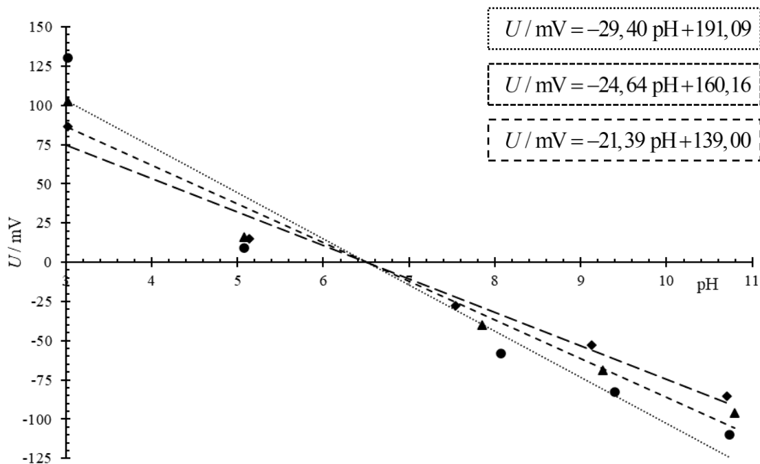
Slika 4.7. Površinski potencijal elektrode Ti/TiO 2 mjereno u otopini natrijeva klorida pri različitim pH-vrijednostima; c(\text{NaCl}) = 1 \times 10^{-3} mol dm -3 (●); 1 \times 10^{-2} mol dm -3 (▲); 1 \times 10^{-1} mol dm -3 (◆), \theta = 25 °C
