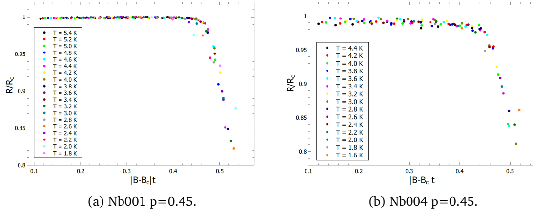
Slika 5.7: Grafovi dobiveni analizom skaliranja za dio izmjerenih uzoraka.
