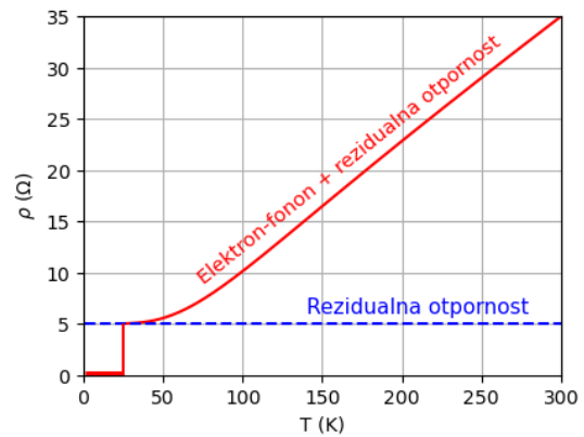
(b) Ovisnost otpornosti o temperaturi kod supravodljivih metala.
