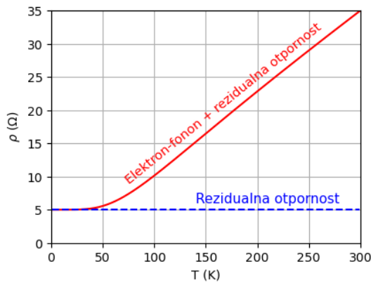
(a) Ovisnost otpornosti o temperaturi kod normalnih metala.
