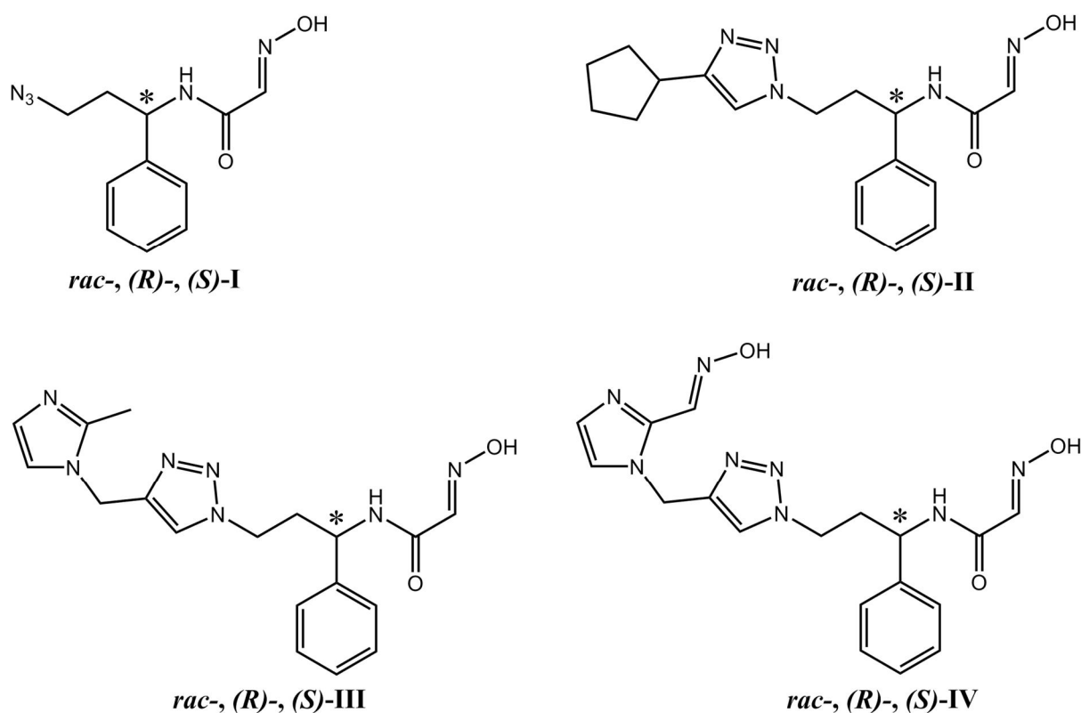
Slika 39. Strukture predloženih novih kiralnih N -supstituiranih 2-hidroksiiminoacetamida.
