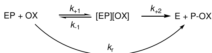
Shema 2. Kinetički model reaktivacije fosfiliranog enzima oksimskim reaktivatorom.
