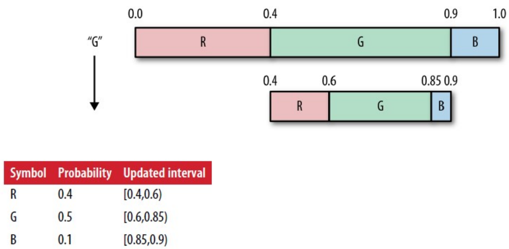
Slika 2.7: Prvi korak aritmetičkog kodiranja.
