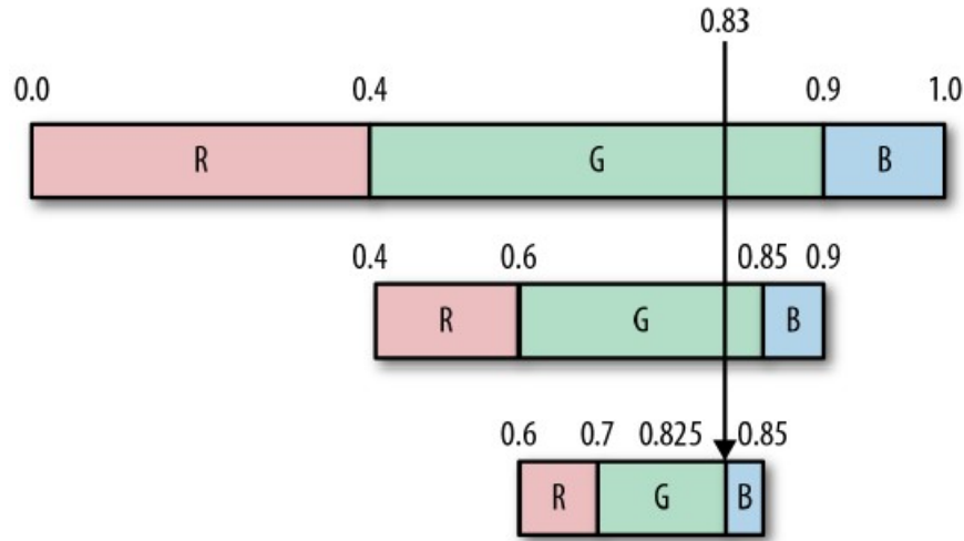
Slika 2.10: Dekodiranje aritmetički kodiranog zapisa.
