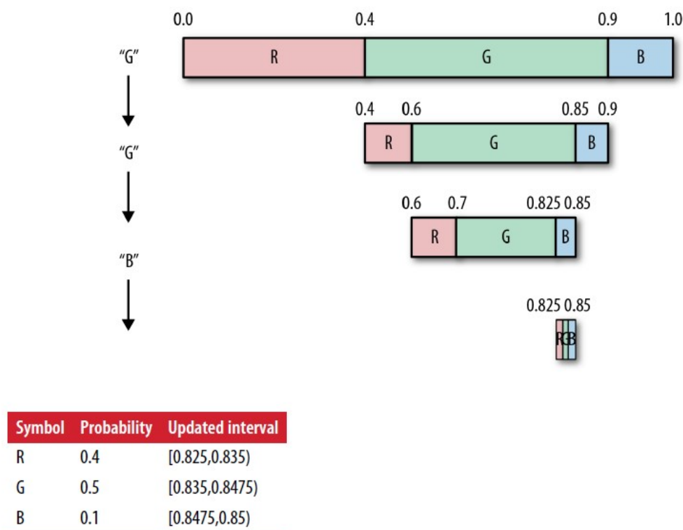
Slika 2.9: Završno stanje algoritma.
