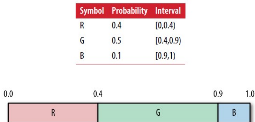
Slika 2.6: Podjela intervala prema tablici.
