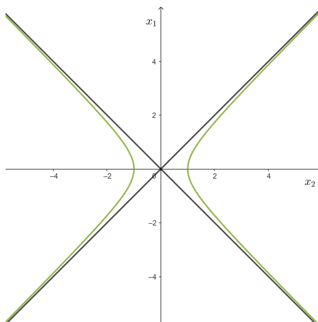
Slika 2.5: Kružnica imaginarnog radijusa
