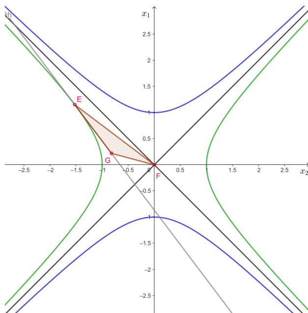
Slika 2.7: Pravokutni trokut - Minkowskijeva ravnina
