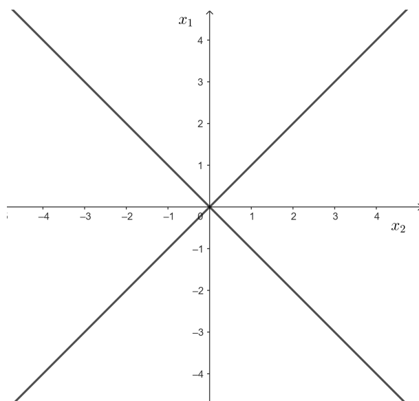
Slika 2.3: Kružnice radijusa 0
