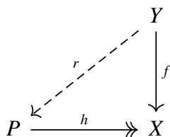
Slika 3.1: Projektivnost
